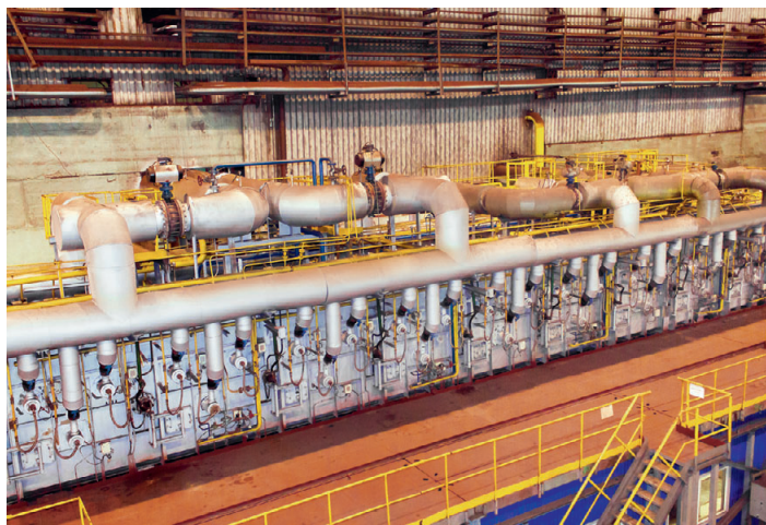
Рис. 3. Печная часть агрегата
