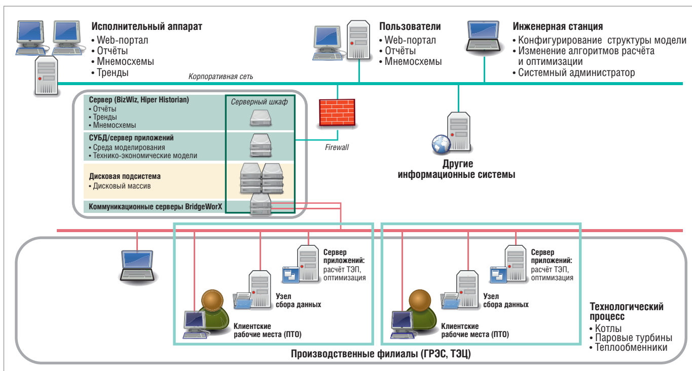
Рис. 11. Структурная схема системы в рамках энергокомпании
