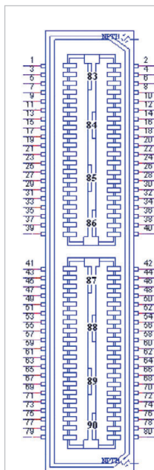
Рис. 1. Схема расположения выводов и распиновка разъёма Samtec QTE-040
