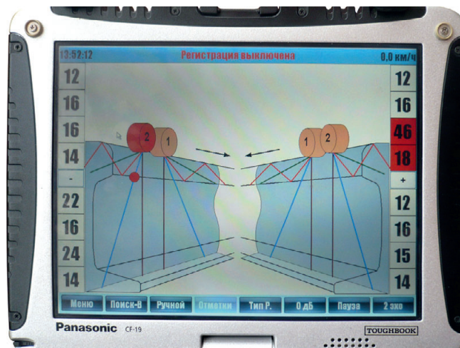
Рис. 8. Новое мнемоническое представление сигналов на экране дефектоскопа АВИКОН-14 (дефект и номер сработавшего канала выделены красным пятном)
