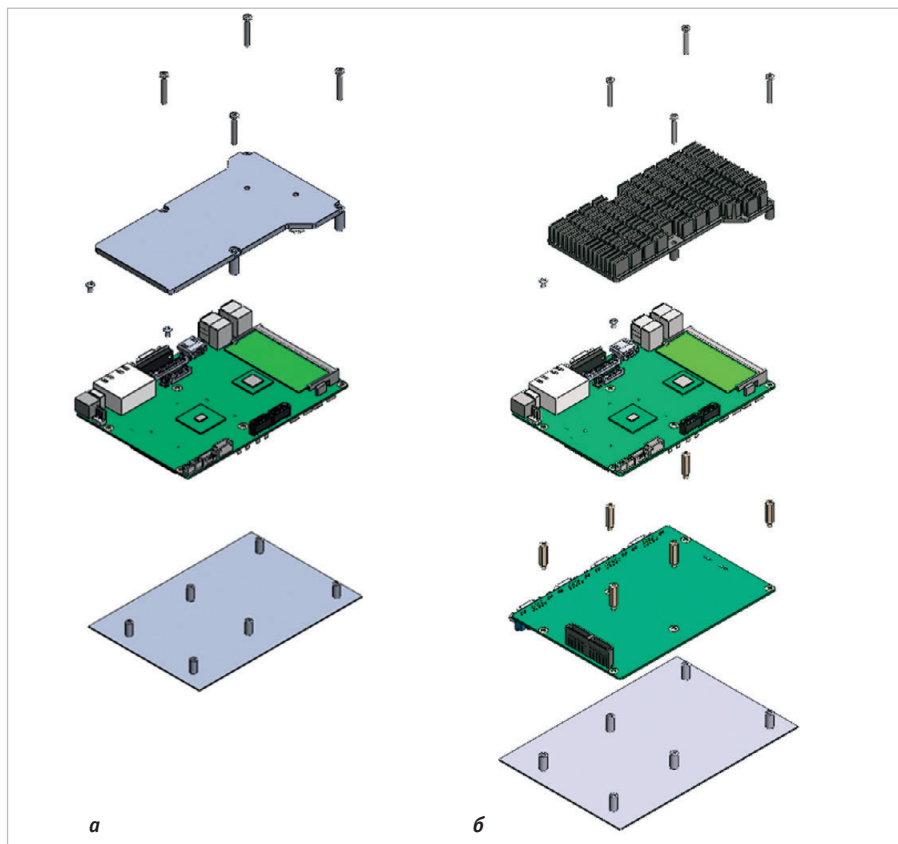
Рис. 2. Варианты монтажа системы:
