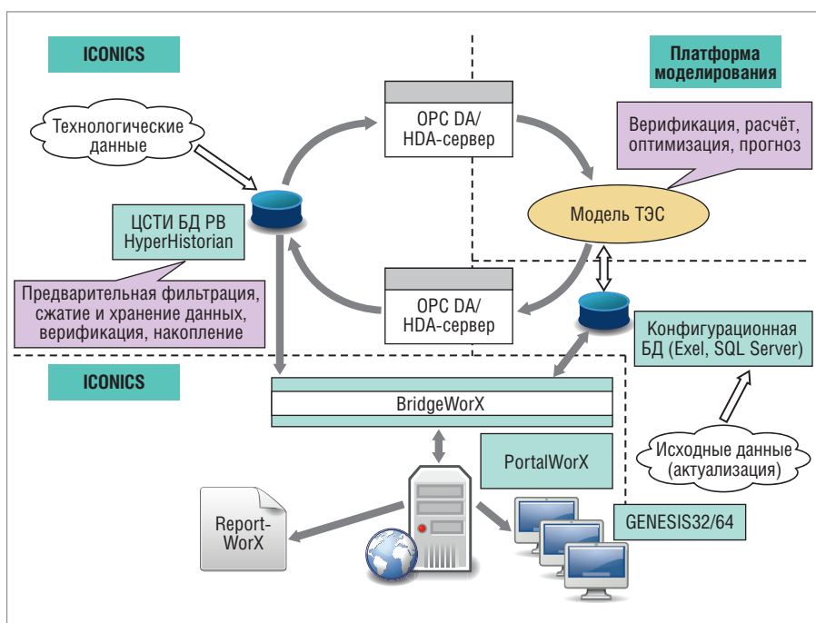
Рис. 1. Архитектура решения
