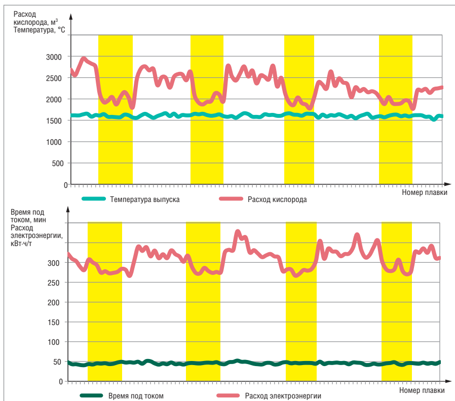
Рис. 7. Графики, иллюстрирующие экономический эффект от применения комплекса управления. Здесь жёлтым цветом выделены смены, работавшие с введёнными в действие системами компенсации
