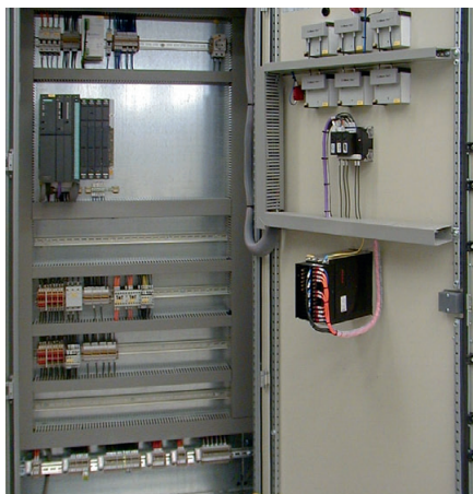
Рис. 3. Контроллер S7-400 на этапе монтажа в шкаф управления
