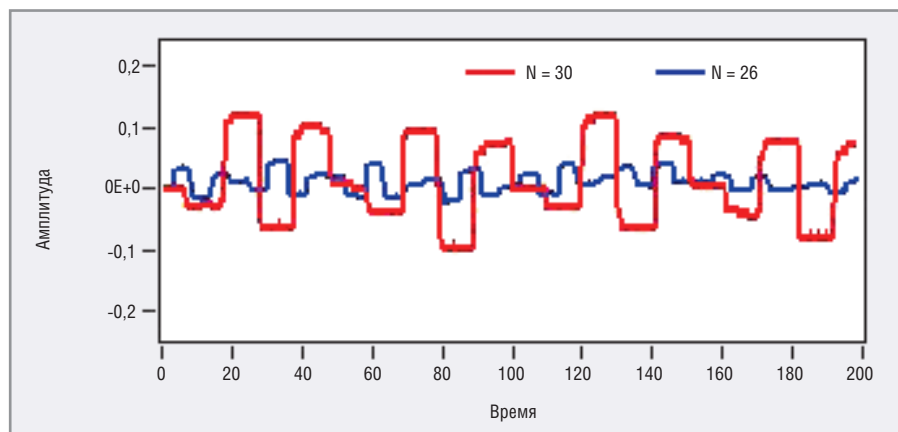
Рис. 2. Амплитуда предельных циклов при нулевом входе
