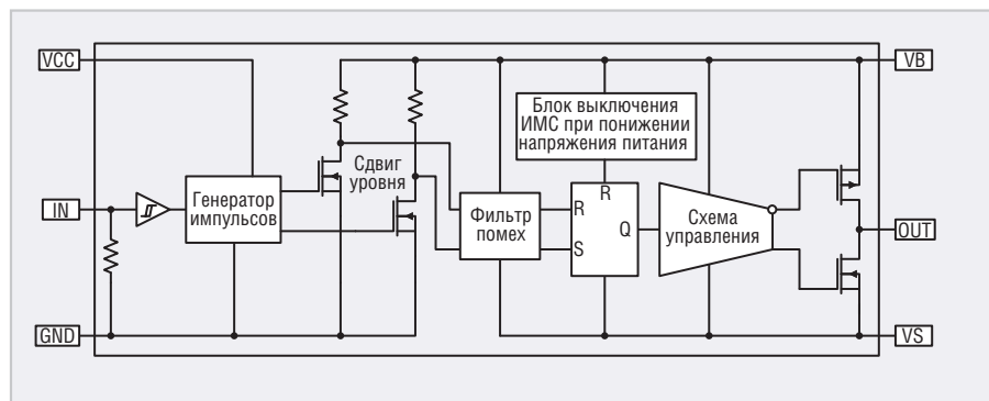
Рис. 10. Обобщённая структурная схема драйвера верхнего ключа
