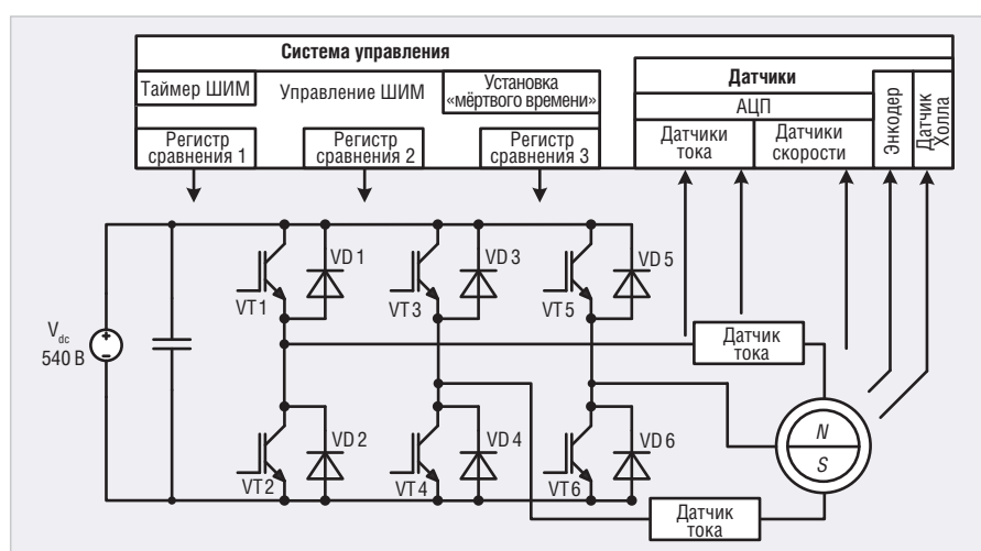
Рис. 6. Функциональная схема электропривода с синхронным двигателем с постоянными магнитами N/S
