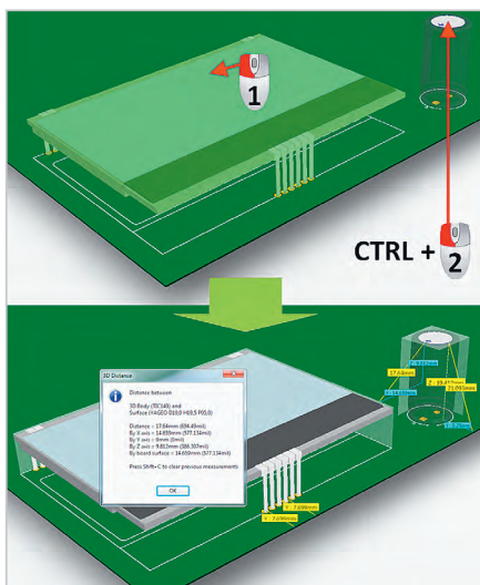
Рис. 11. Команда Measure 3D Object – измерение расстояния между 3D-объектами
