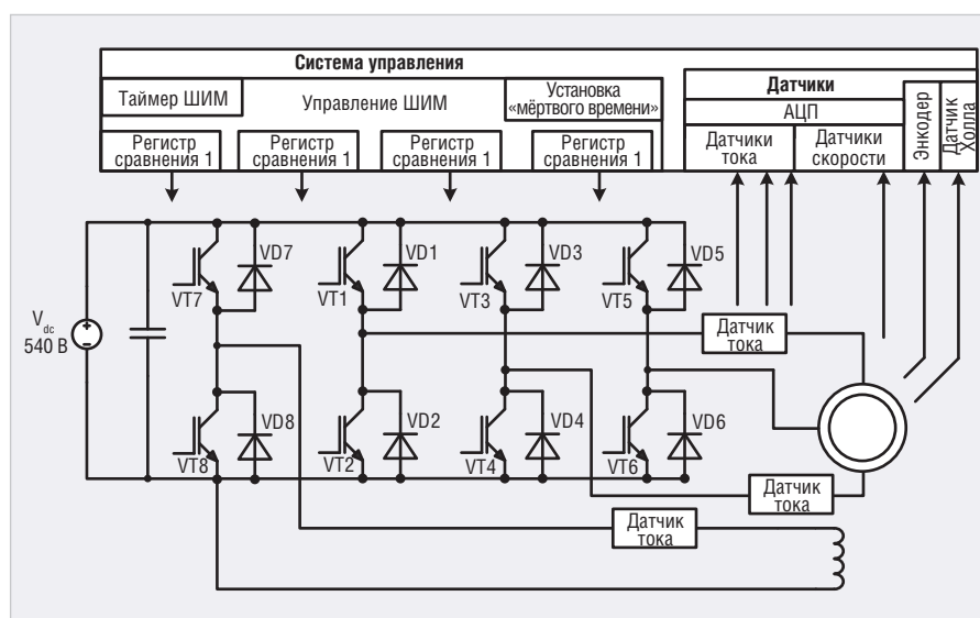
Рис. 7. Функциональная схема электропривода с синхронным двигателем с обмоткой возбуждения
