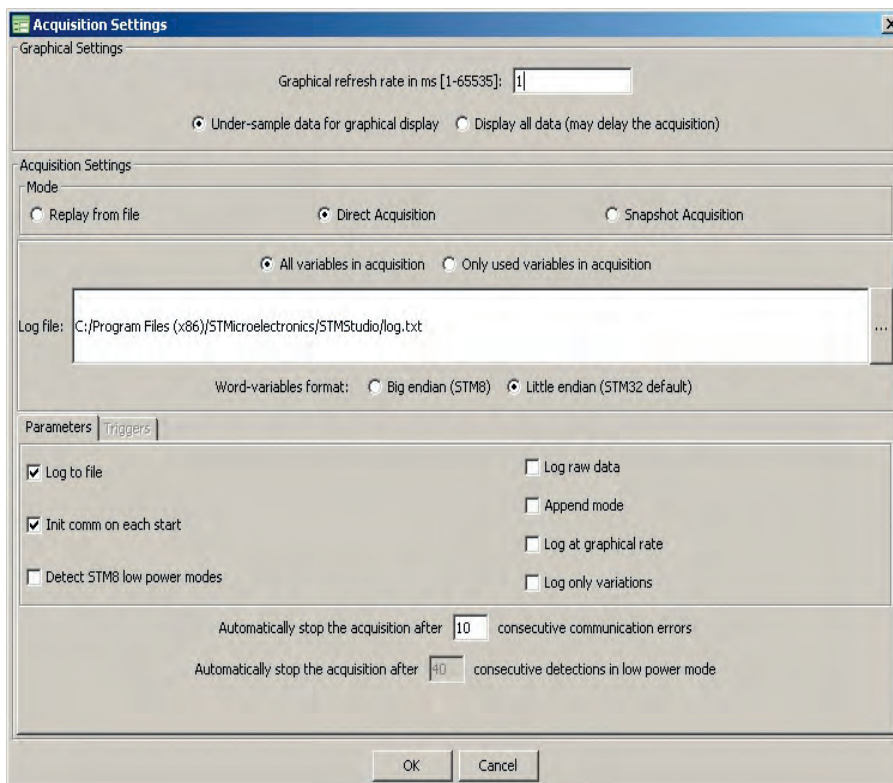
Рис. 3. Окно дополнительных настроек
