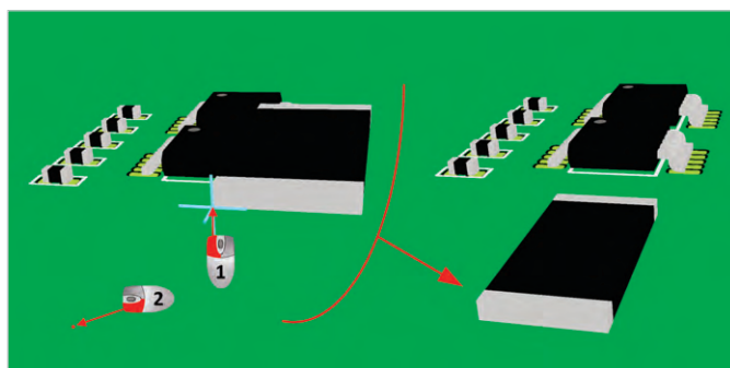
Рис. 6. Команда Position 3D Body – перенос модели за счёт совмещения двух точек
