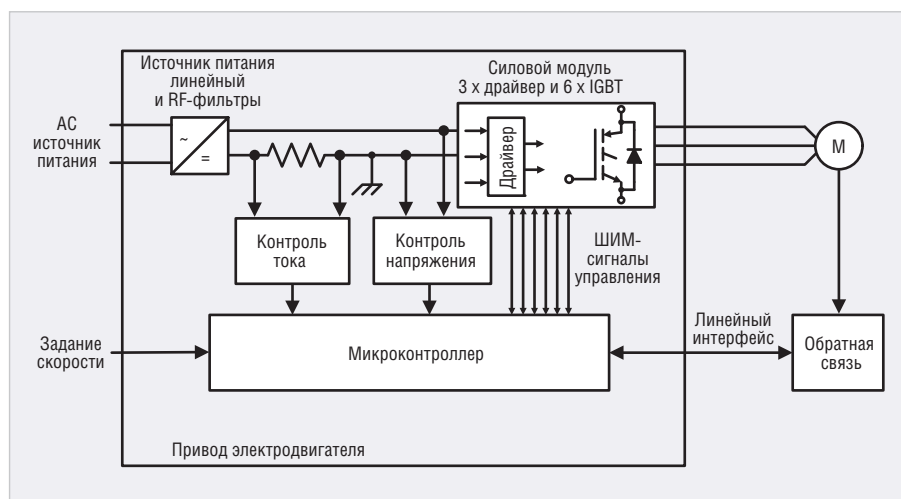
Рис. 1. Блок-схема электропривода с процессорным управлением
