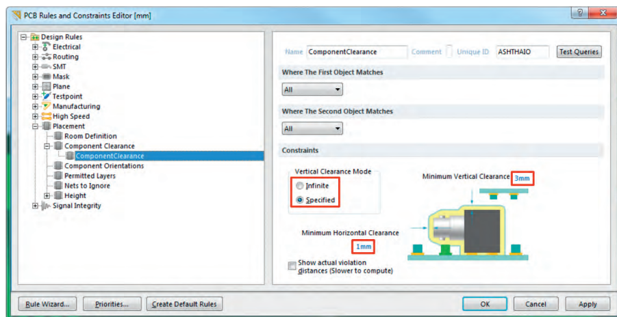
Рис. 12. Правило Component Clearance
