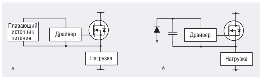
Рис. 9. Схема питания драйверов верхнего ключа от «плавающего» источника питания (а) и от бутстрапной ёмкости (б)
