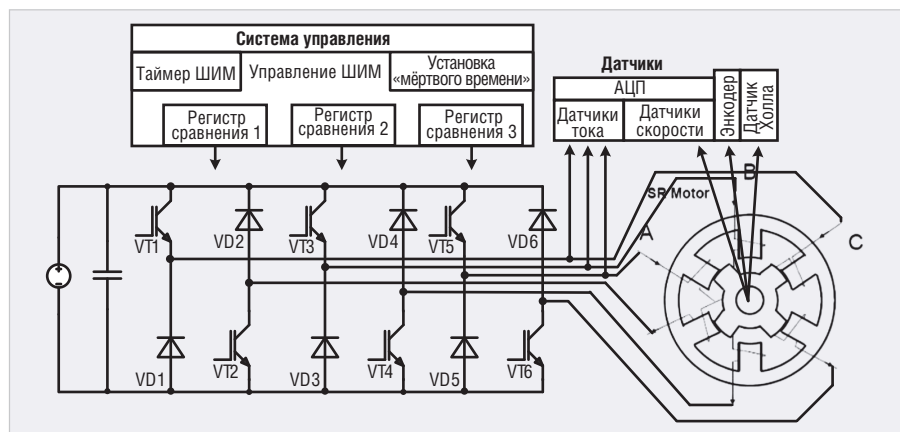
Рис. 8. Функциональная схема вентильно-индукторного электропривода
