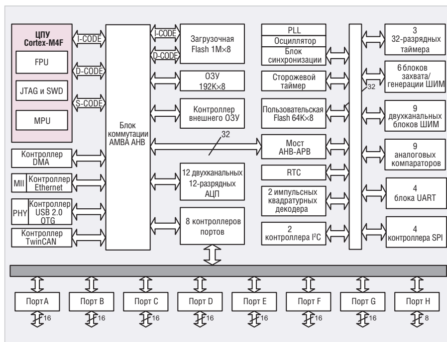
Рис. 3. Блок-схема 32-разрядного микроконтроллера на базе ядра ARM Cortex M4F
