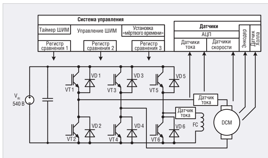
Рис. 4. Функциональная схема электропривода с двигателем постоянного тока DCM
