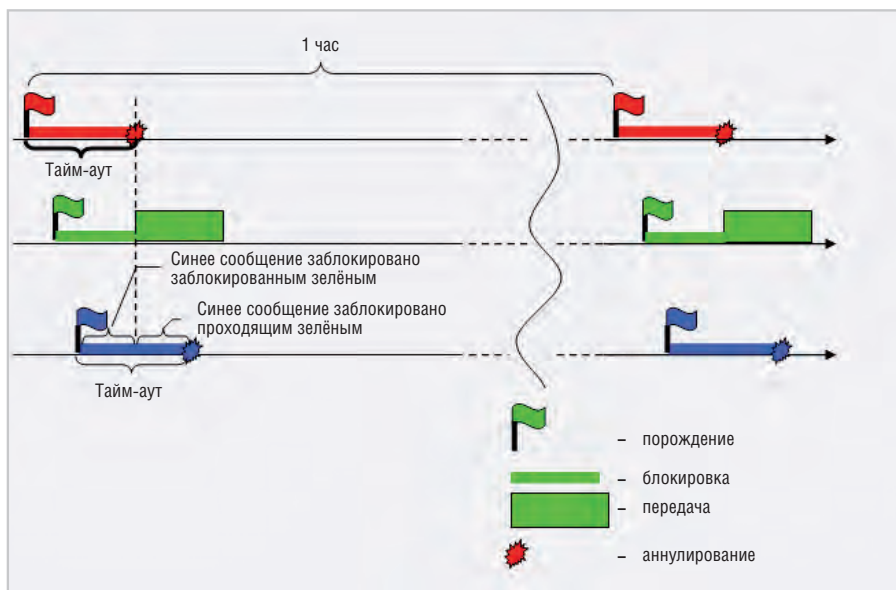
Рис. 7. Временная диаграмма синхронизированных столкновений
