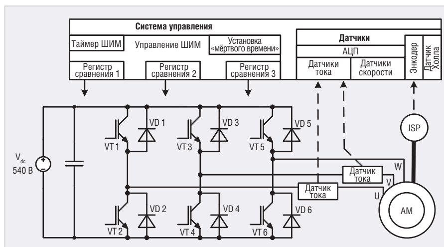
Рис. 5. Функциональная схема электропривода с асинхронным двигателем AM
