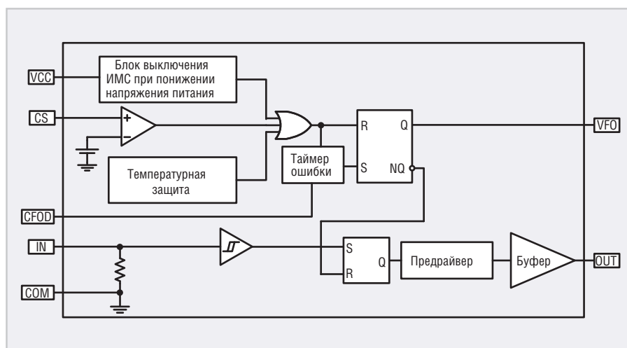
Рис. 11. Обобщённая структурная схема драйвера нижнего плеча
