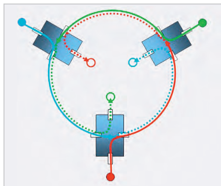
Рис. 8. Deadlock на циклической сети
