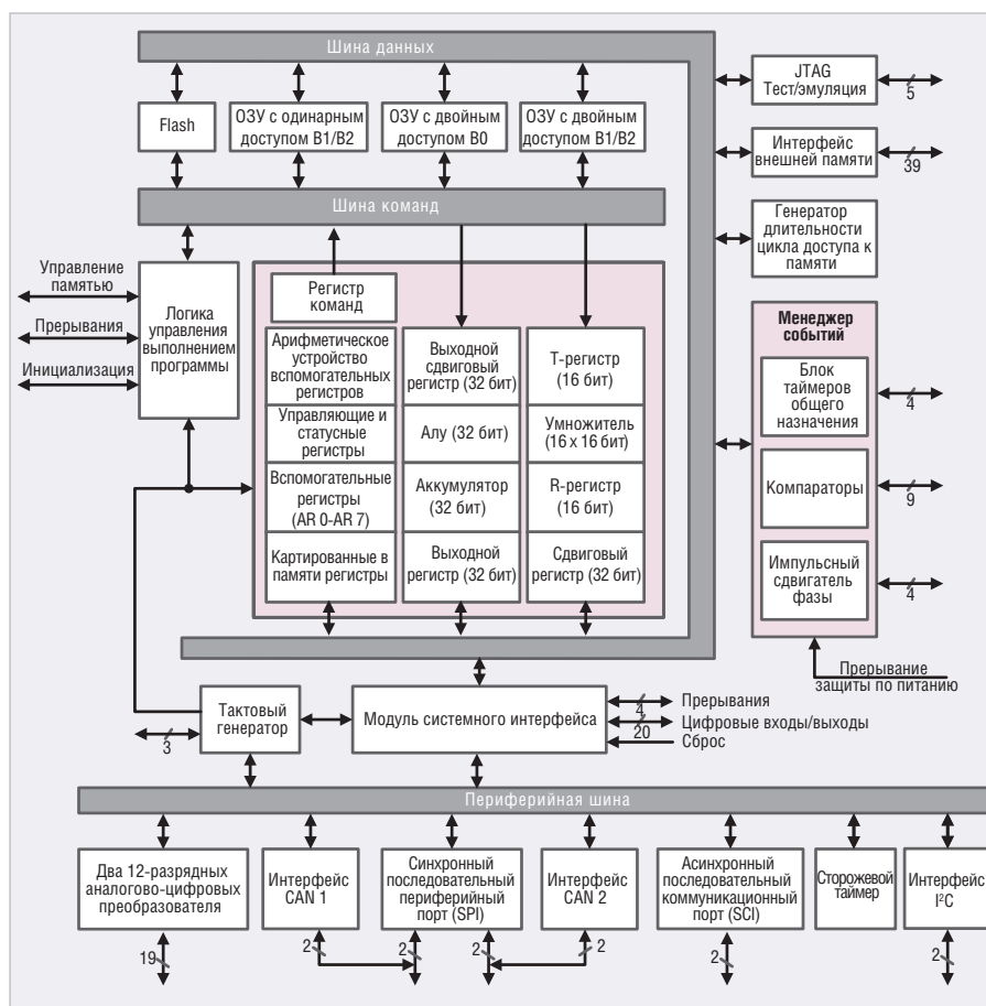
Рис. 2. Блок-схема 16-битного микроконтроллера цифровой обработки сигналов с фиксированной запятой
