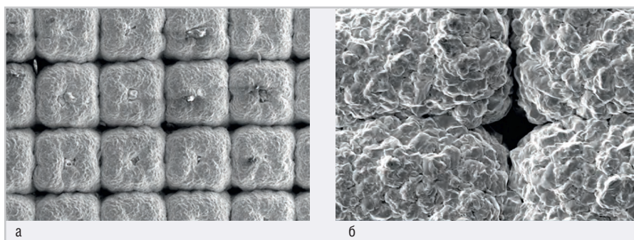
Рис. 6. Микрофото керамической подложки после гальванического покрытия медью: а) вид при увеличении \times 100 ; б) вид при увеличении \times 400
