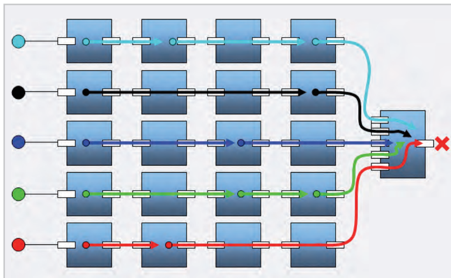
Рис. 2. Исходные узлы, неспособные диагностировать блокировку
