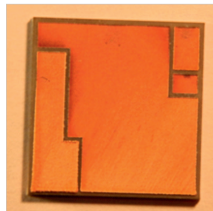
Рис. 8. Фото керамической подложки с топологическим рисунком, покрытым медным слоем толщиной 50 мкм
