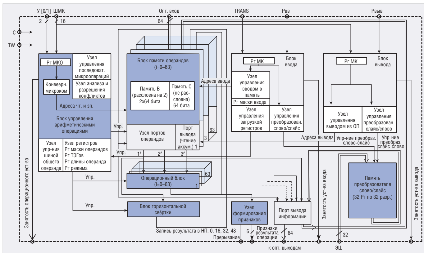
Рис. 32. Блок-схема 3D М ФЭ СБИС ПФ
