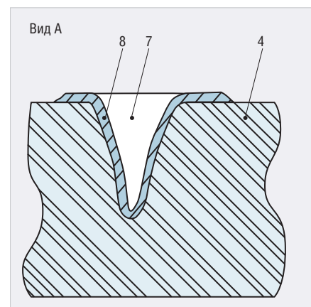
Рис. 2. Вид лунки (кратера) в поперечном сечении после воздействия на неё лазерного излучения
