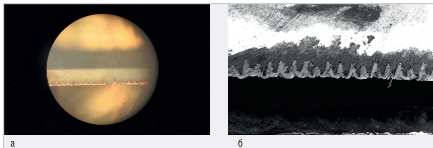
Рис. 7. Микрофото поперечной структуры лазерных микроканалов (треков), заполненных медью: а) выполненное с помощью оптического микроскопа при увеличении \times 10 ; б) выполненное с помощью электронного микроскопа при увеличении \times 50
