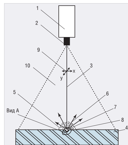
Рис. 1. Схема воздействия мощного сфокусированного лазерного излучения на поверхность областей металлизации топологического рисунка керамической пластины
