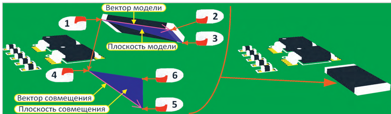
Рис. 5. Команда Orient And Position 3D Body – перенос модели с поворотом
