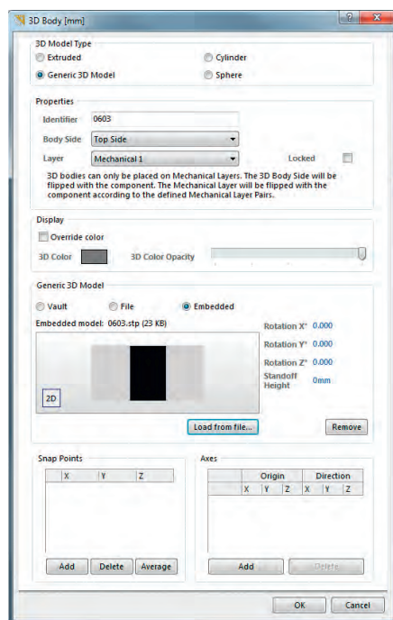
Рис. 1. Окно 3D Body
