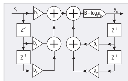
Рис. 1. Структура звена рекурсивного ЦЦФ
