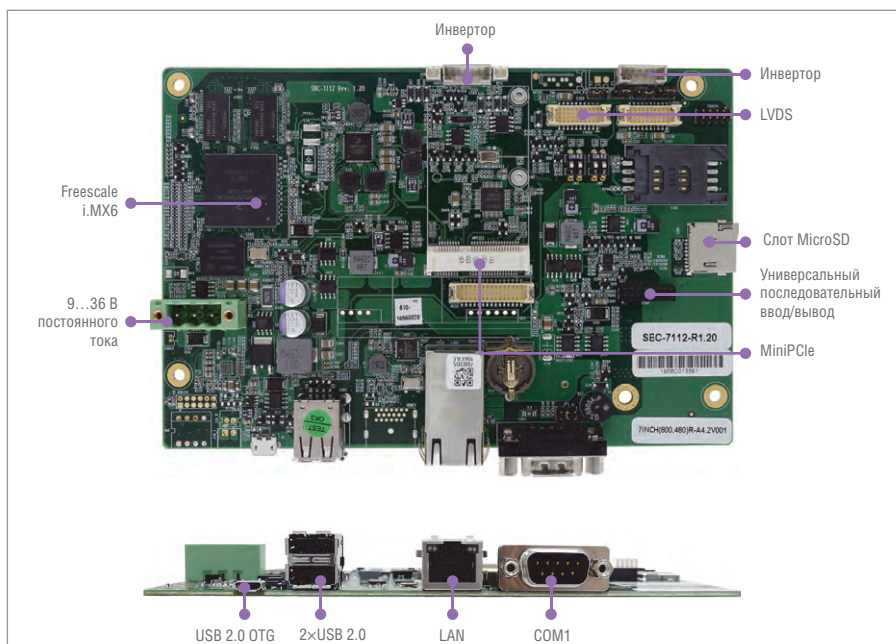
Рис. 1. Одноплатный компьютер SBC-7112
