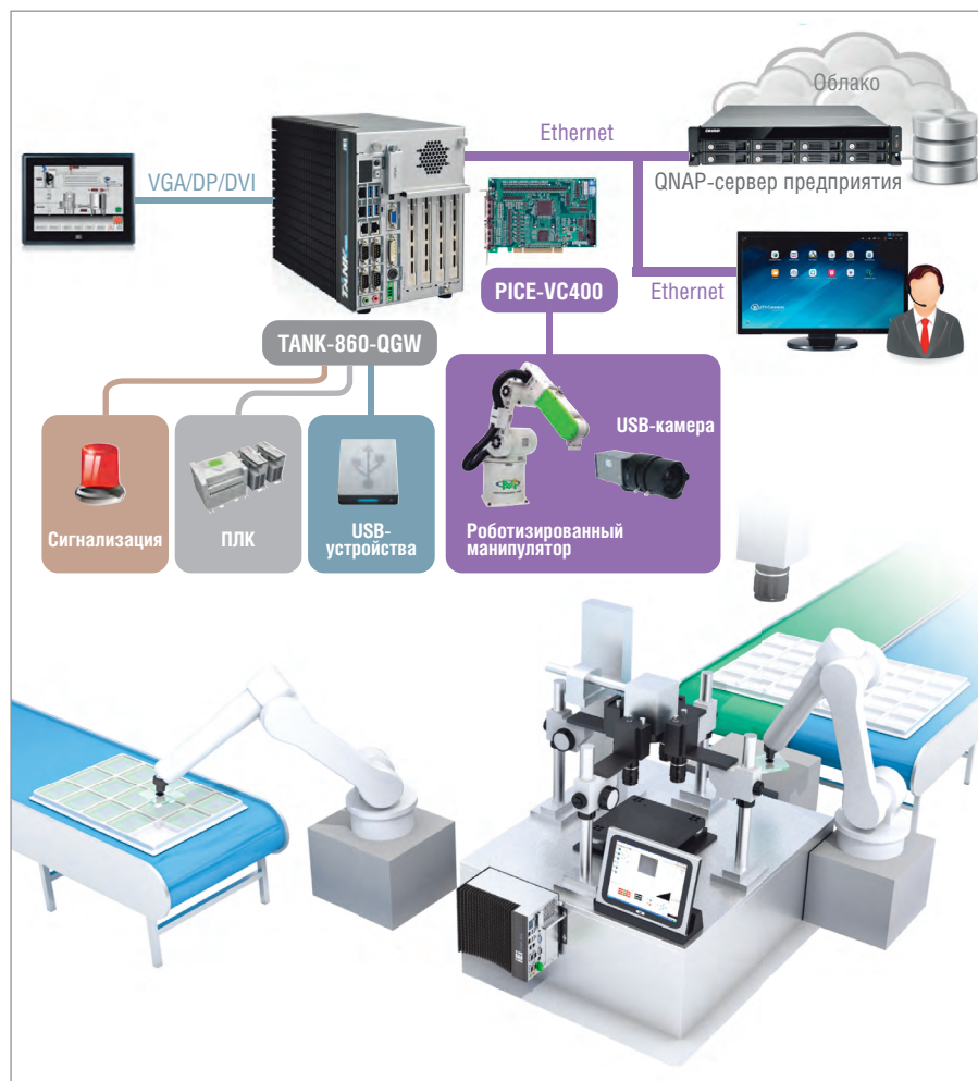
Рис. 5. Схема управления роботом
