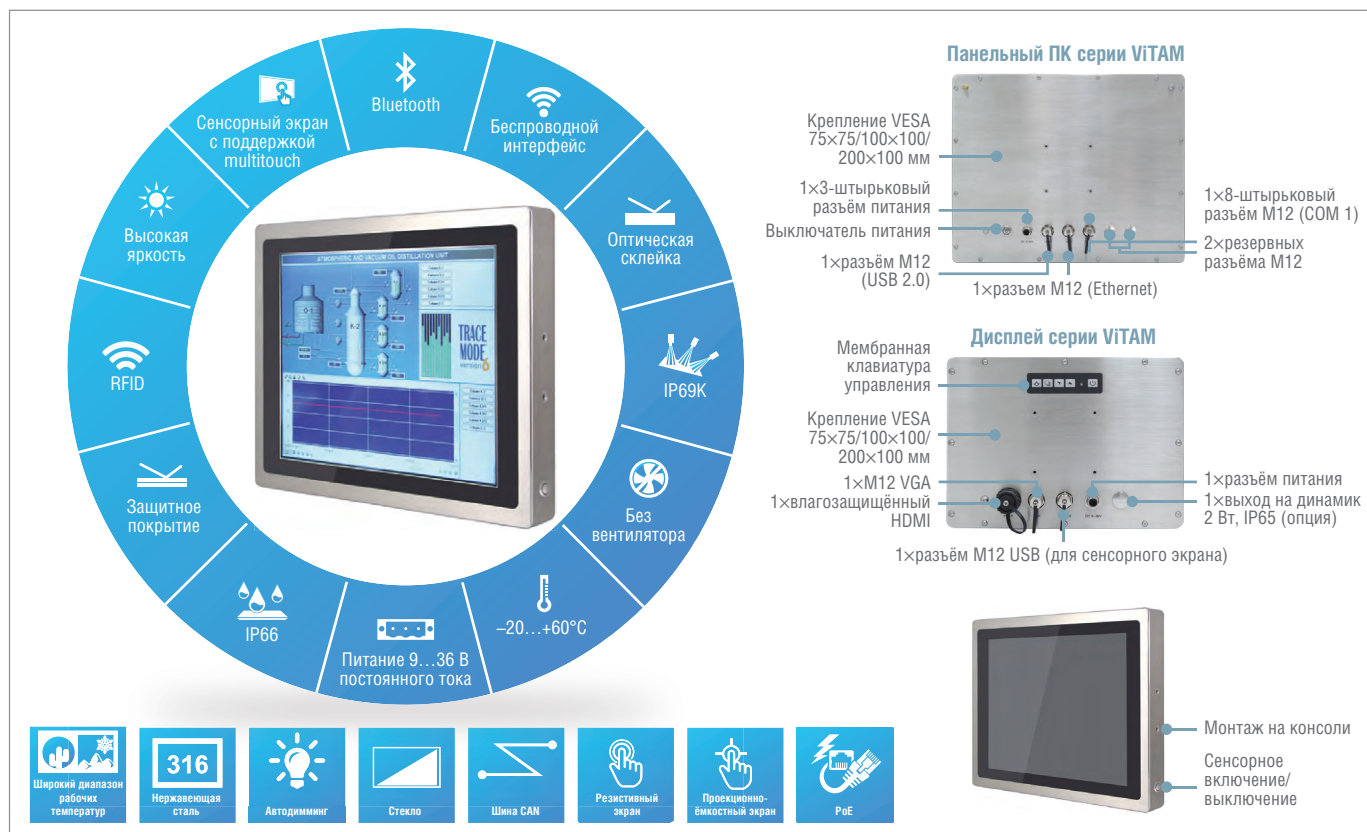
Рис. 5. Конструктивное исполнение и особенности серии ViTAM
