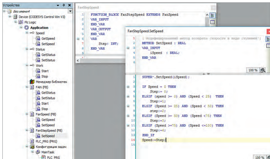
Рис. 17. Преобразование метода SetSpeed
