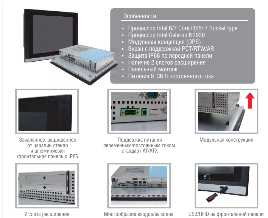
Рис. 4. Панельные компьютеры ViPAC
