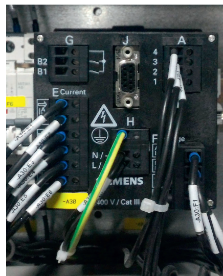
Рис. 4. Измеритель мощности SIMEAS P
