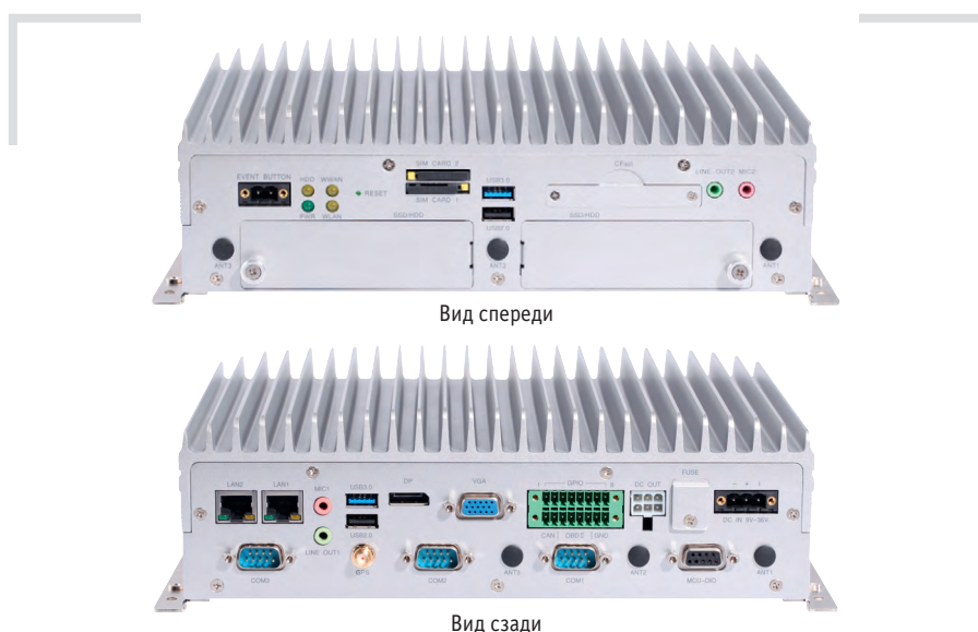
Рис. 3. Мобильный видеорегистратор GV-MNVR2100
