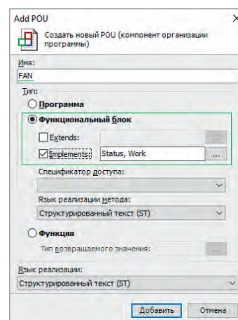
Рис. 7. Поле Implements позволяет добавлять интерфейсы, реализованные в данном классе
