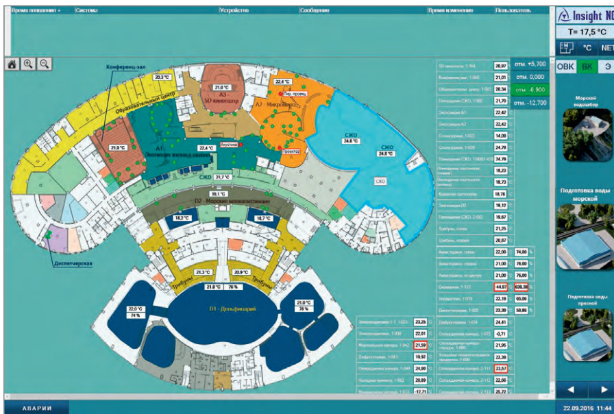
Рис. 5. План здания. Отметка –6,900
