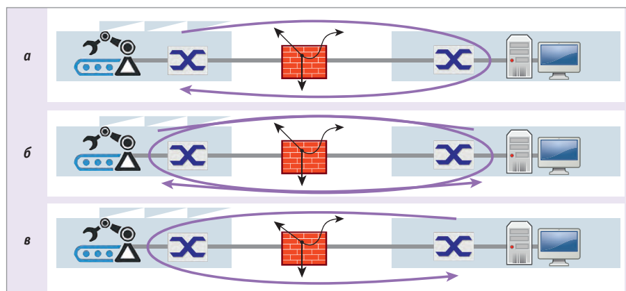
Рис. 6. Построение соединения при помощи различных режимов NAT:
