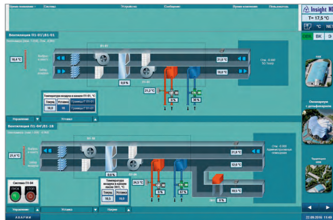
Рис. 4. Пример мнемосхемы системы вентиляции
