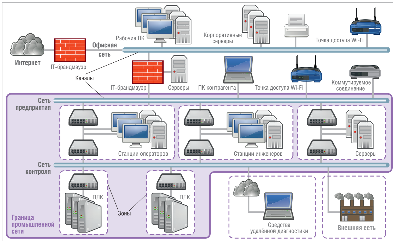
Рис. 1. Пример сети промышленного объекта
