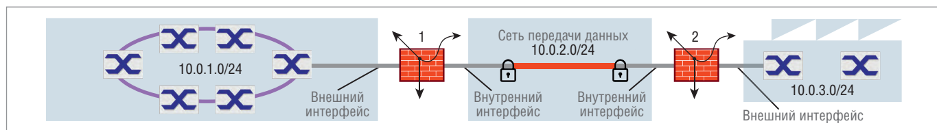
Рис. 7. Защищённое соединение на основе VPN-туннеля: 1, 2 – промышленные брандмауэры
