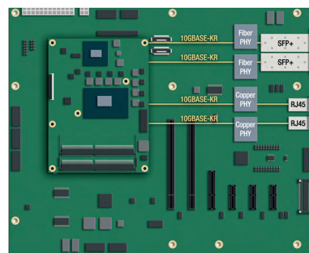
Рис. 5. 4 порта 10 GbE-KR по оптоволокну/медному проводу, SFP+/RJ
