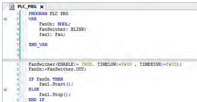
Рис. 10. Объект fan1, принадлежащий классу Fan
