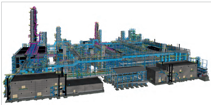
Рис. 1. Визуализация проекта комбинированной установки ЛК-2Б ООО «КИНЕФ»
