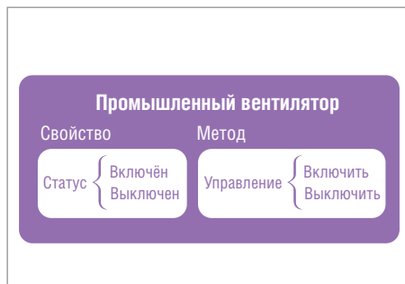
Рис. 2. Структурная схема класса, описывающего промышленные вентиляторы
