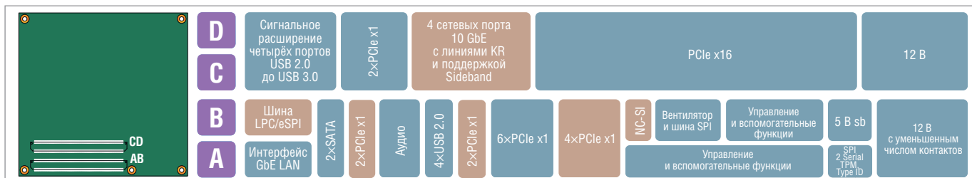
Рис. 1. Оптимизированная раскладка разъёма COM Express тип 7
