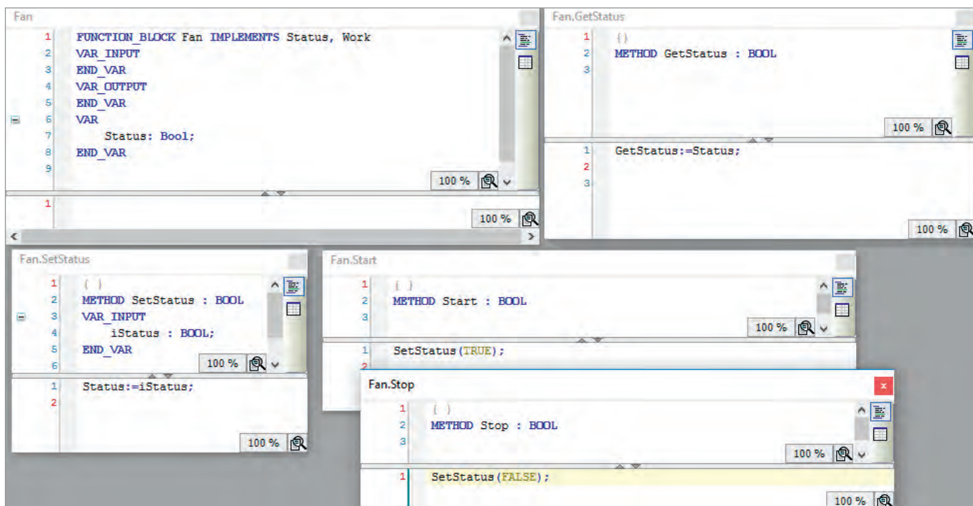
Рис. 8. Созданный класс вентиляторов Fan (методы, созданные в интерфейсе, автоматически перенесены в этот класс)
