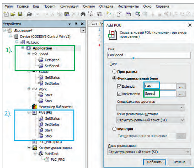
Рис. 12. Создание нового класс FanSpeed
