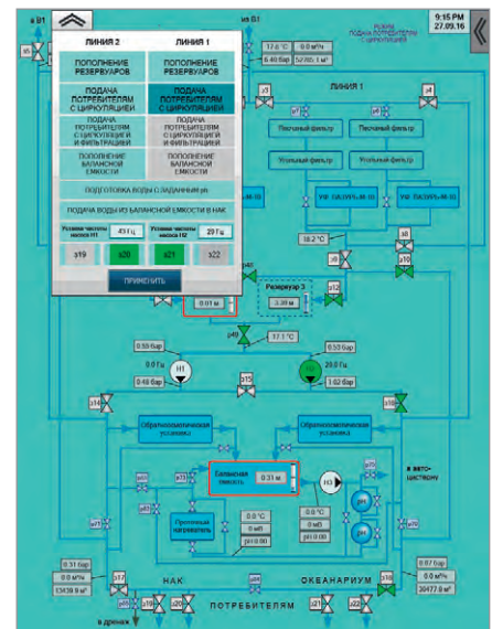
Рис. 6. Мнемосхема мониторинга системы водоподготовки на сенсорной панели
