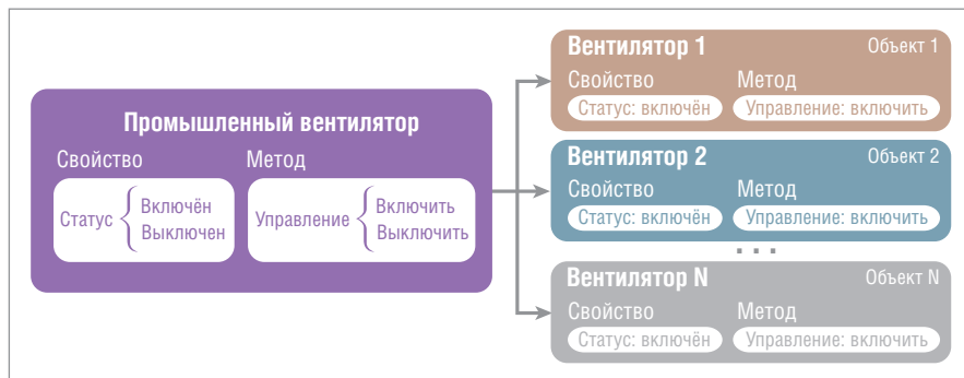
Рис. 3. N объектов (экземпляров), относящихся к классу вентиляторов
