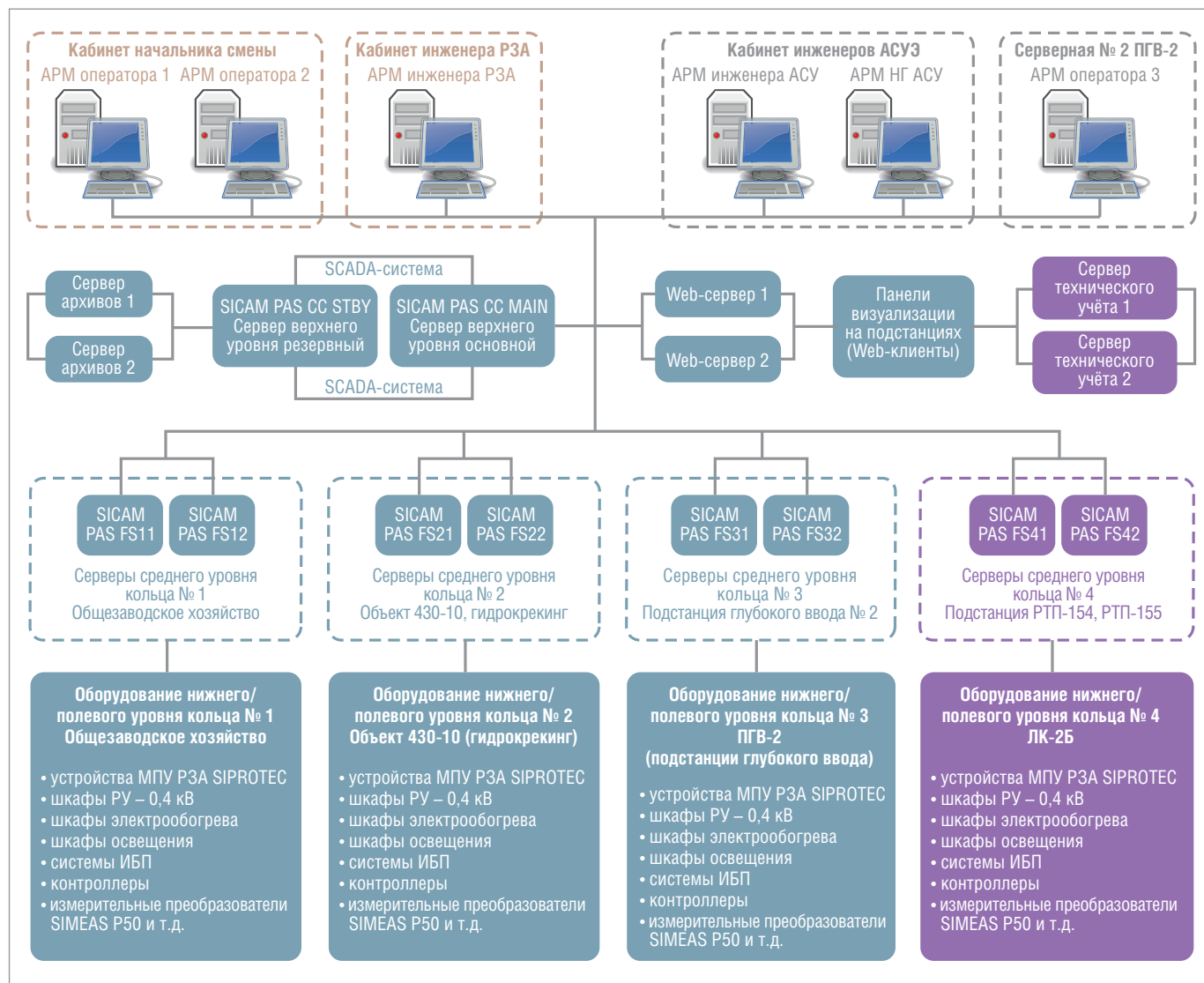
Рис. 3. Структурная схема АСУЭ ЗГПН с учётом объекта ЛК-2Б: голубой цвет – существующее оборудование, фиолетовый цвет – оборудование для ЛК-2Б
