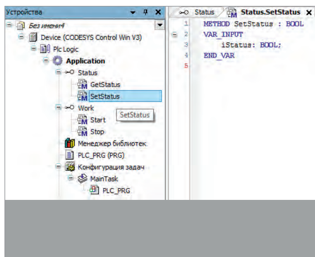
Рис. 6. Реализация метода SetStatus, имеющего возвращаемый тип BOOL
