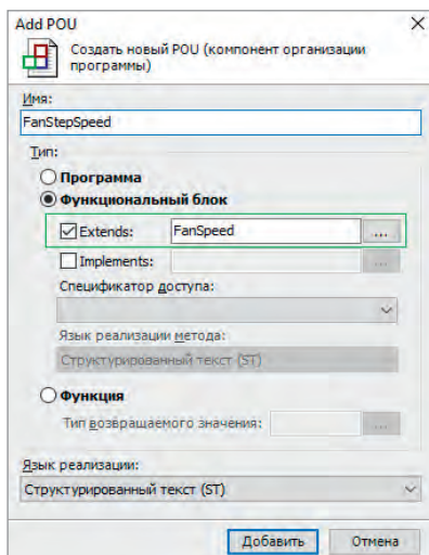
Рис. 16. Класс FanStepSpeed, созданный на базе класса FanSpeed
