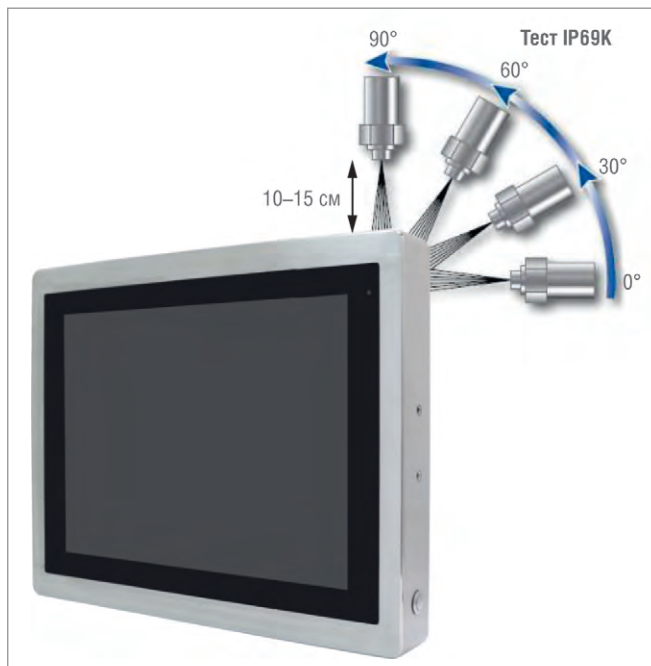
Рис. 2. Процесс тестирования на соответствие IP69K
