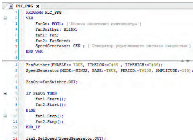
Рис. 14. Код, вызывающий объекты классов Fan и FanSpeed
