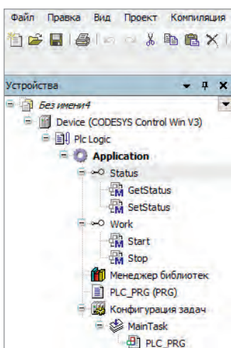
Рис. 5. Интерфейсы, определяющие работу класса
