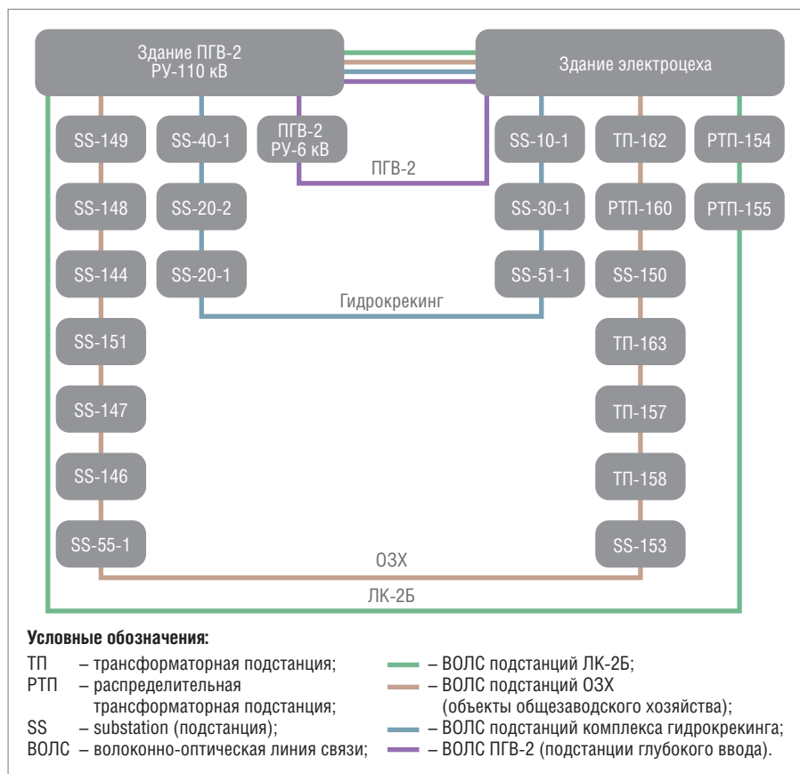
Рис. 2. Расширение существующего перечня колец АСУЭ ЗГПН кольцом АСУЭ ЛК-2Б
