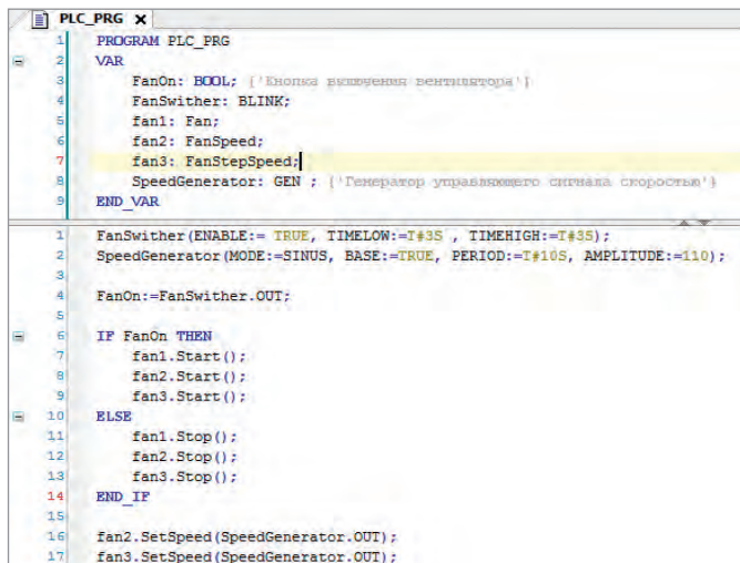
Рис. 18. В программный код добавлен объект fan3, принадлежащий классу FanStepSpeed
