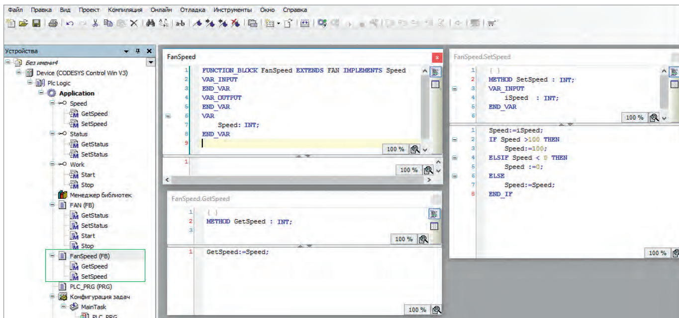
Рис. 13. Реализация нового класса FanSpeed
