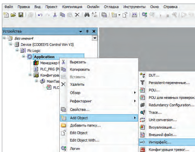
Рис. 4. Создание интерфейса класса
