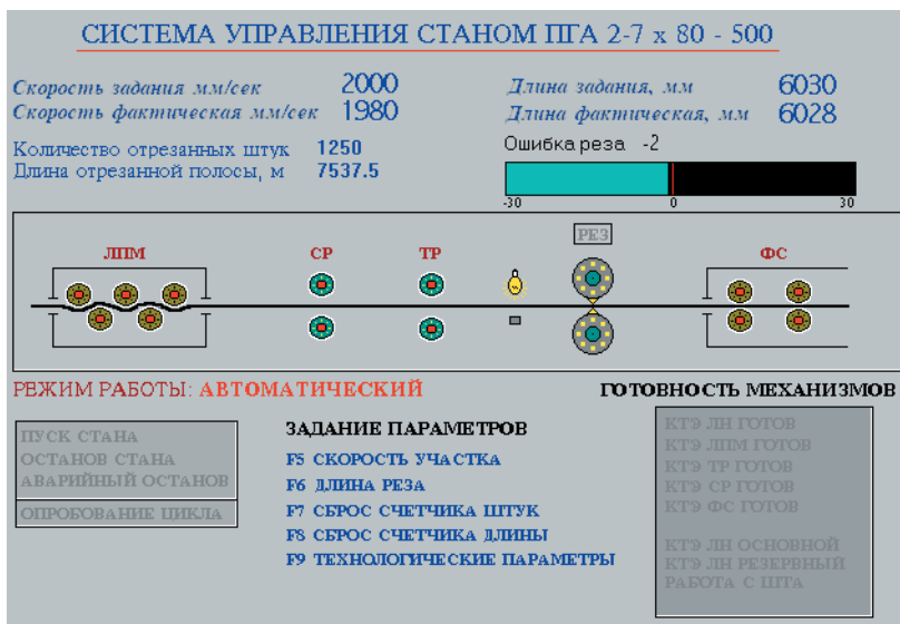
Рис. 4. Вид рабочего экрана на пульте управления
