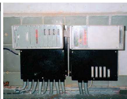
Два контроллера заменили старую систему управления тепловым пунктом
