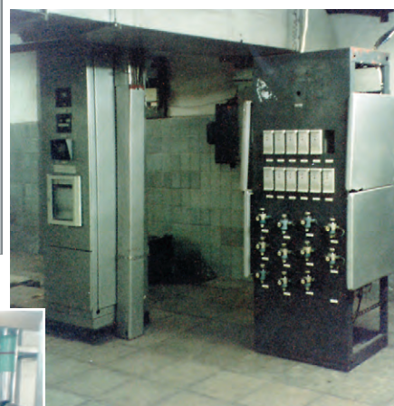
Так выглядела старая система управления тепловым пунктом
