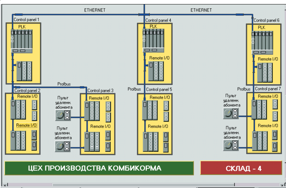
Рис. 3. Структура распределенной системы управления АС «Композит-2М» (уровень технологических станций)
