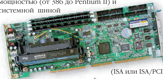
Высокопроизводительная процессорная плата PCA-6175 на базе Pentium II
