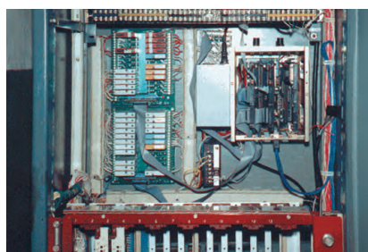
Рис. 2. Внешний вид контроллера промышленной автоматики
