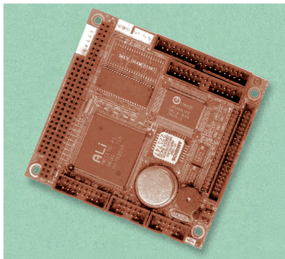
Процессорный модуль РСМ-3335 (386SX/40 МГц) в формате PC/104
