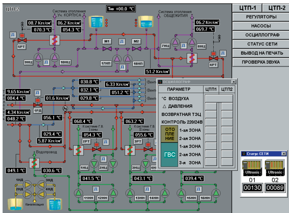
Рис. 2. Фрагмент мнемосхемы системы управления теплоснабжением
