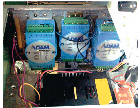
Рис. 3. Расположение модулей ADAM в стойке управления установки
