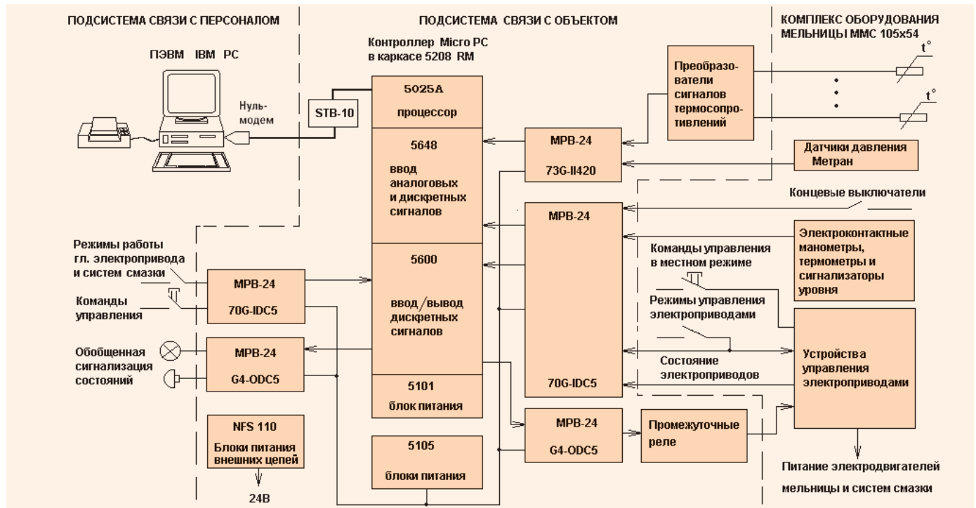
Рис. 2. Упрощенная структурная схема АСУ мельницы ММС 105*54
