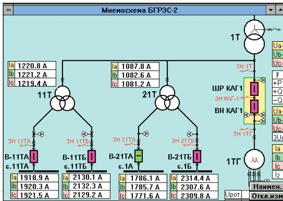
Рис. 7. Пример мнемосхемы объекта
