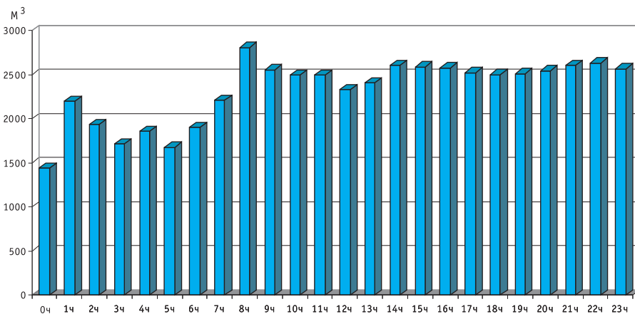
Рис. 8. Суточная расходограмма
