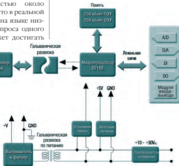
Рис. 3. Структурная схема контроллера на базе ADAM-5510
