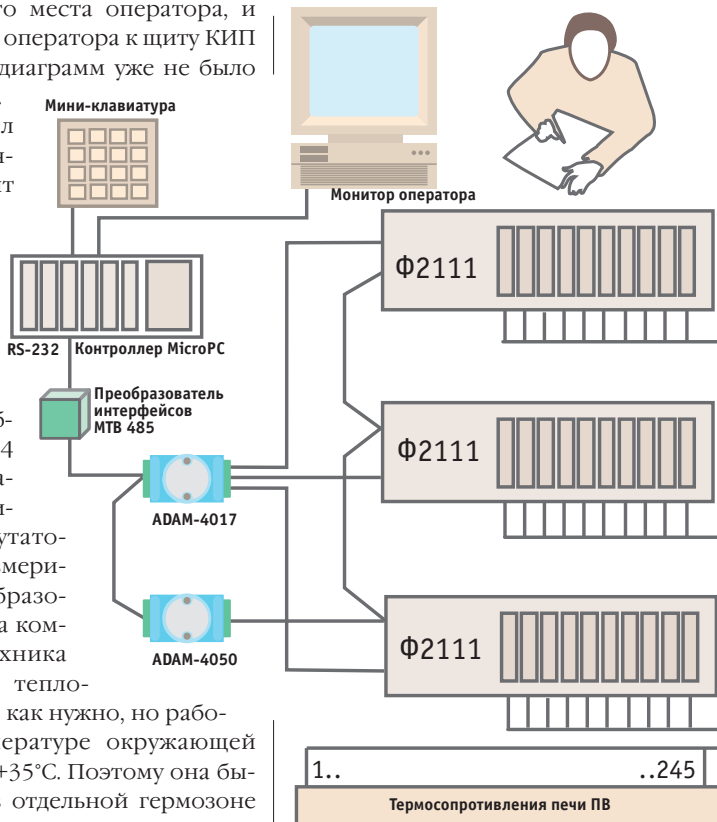
Рис. 2. Блок-схема системы теплоконтроля печи
