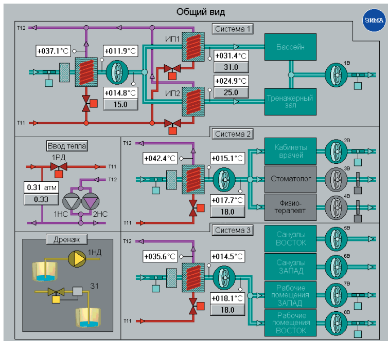
Рис. 3. Фрагмент мнемосхемы управления вентилляцией
