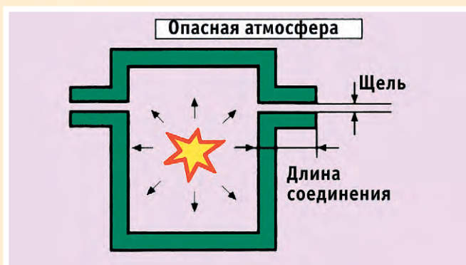
Рис. 2. Взрывонепроницаемая оболочка
