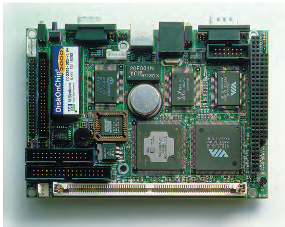
Одноплатный компьютер РСМ-4823 (5x86/133 МГц) с VGA, Ethernet и флэш-дискон
