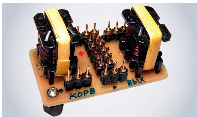
Рис. 29. Фотография платы регулятора громкости на Ш-образных сердечниках Е 13/7/4
