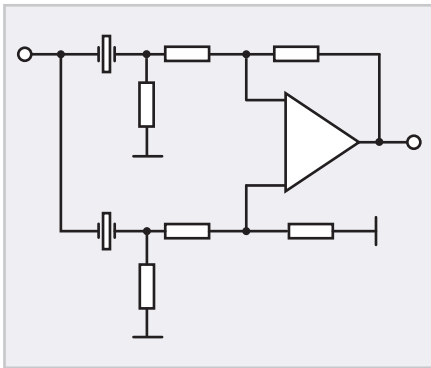
Рис. 3. Схема активного кварцевого фильтра, подключенного к вычитателю, реализованного с помощью операционного усилителя, включенного по дифференциальной схеме
