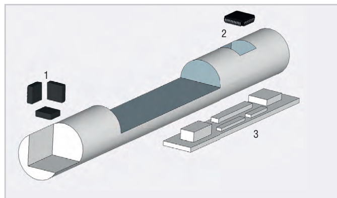
Рис. 1. Классическая компоновка навигационного модуля скважинного оборудования: 1 – акселерометры, 2 – гироскопы/магнитометры, 3 – блок электроники
