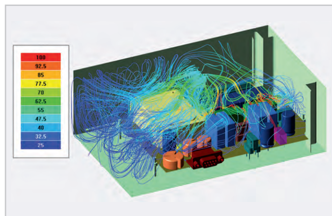
Рис. 9. Линии тока воздуха и их температура, °C
