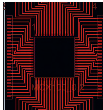
Рис. 5. Ортогональная однослойная трассировка прямоугольной буферной зоны
