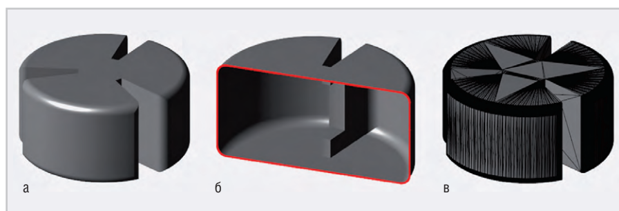
Рис. 3. Геометрическая модель на примере катушки: а – твердотельная ; б – поверхностная, в – сеточная
