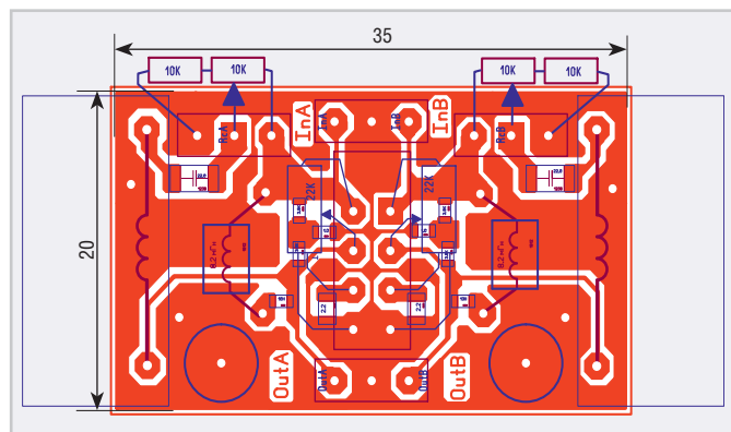
Рис. 30. Печатная плата регулятора громкости на кольцах TX16/9,6/6,3-3E12
