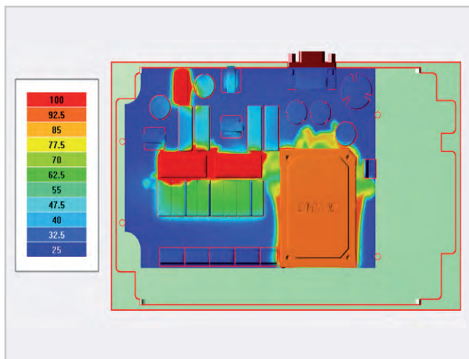
Рис. 10. Температура поверхности компонентов платы, °C
