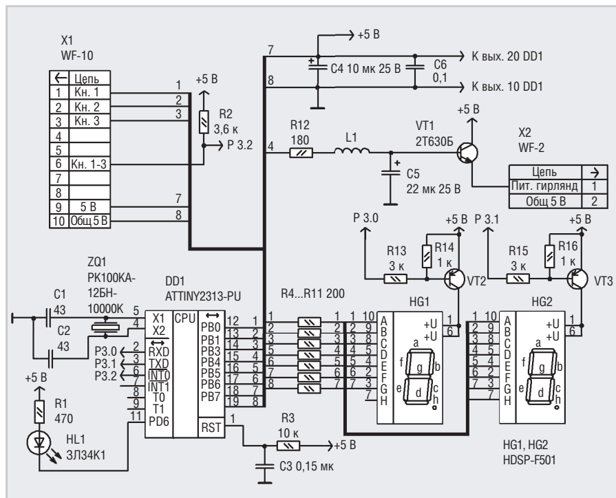
Рис. 3. Принципиальная схема контроллера управления яркостью
