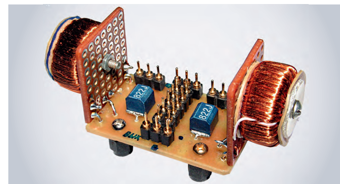
Рис. 31. Фотография платы регулятора громкости на кольцах TX16/9,6/6,3-3E12
