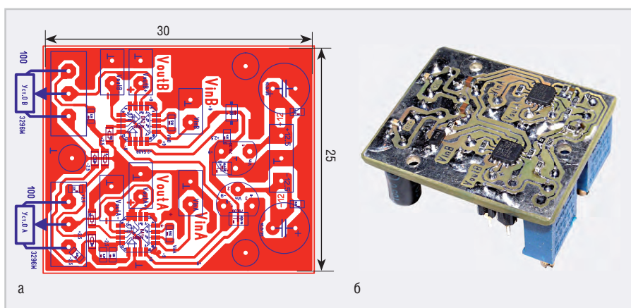
Рис. 16. Предварительный усилитель: а) печатная плата; б) фото со стороны проводников
