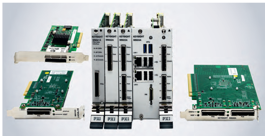
Рис. 3. Контроллер PXI и интерфейсные карты
