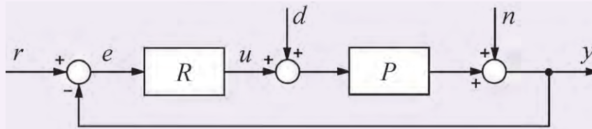
Рис. 3. ПИД-регулятор в системе с шумом n и внешними возмущениями d
