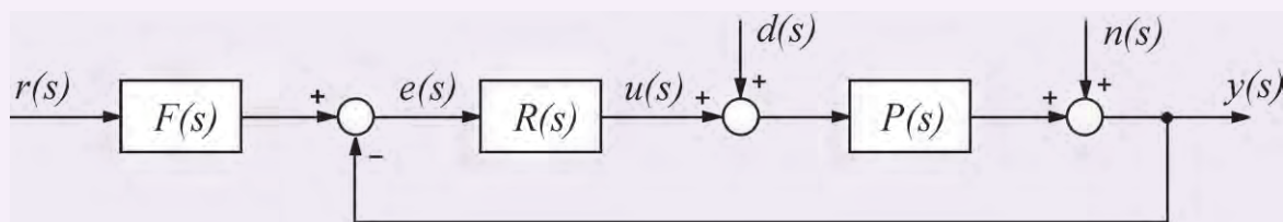
Рис. 10. Выделение блока F(s) в структуре ПИД-регулятора
