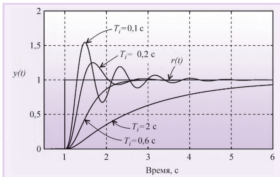
Рис. 5. Реакция на скачок r(t) замкнутой системы 2-го порядка (5) с И-регулятором при T_i = 0,1 с и разных T_i
