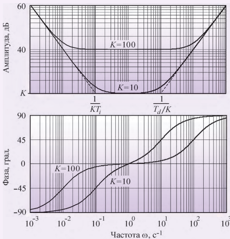
Рис. 2. АЧХ и ФЧХ ПИД-регулятора при T_i = 1 с, T_d = 1 с, K = 10 и K = 100
