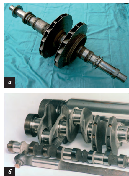
Рис. 2. Вал турбодетандера с восстановленными опорными шейками (а) и восстановленные детали автомобиля (б)
