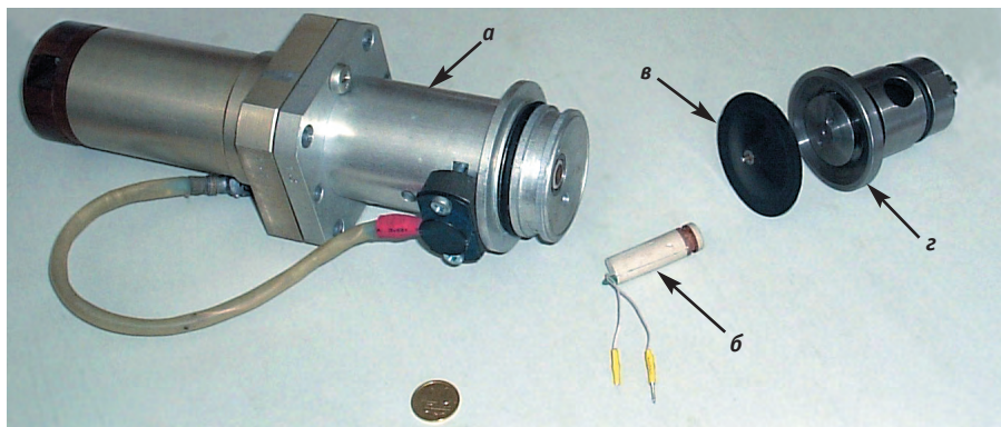
Рис. 5. Унифицированный узел управления: электромагнитный клапан (а), датчик срабатывания (б), мембрана (в), газовый исполнительный клапан (г)
