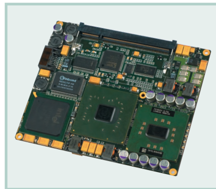
Рис. 3. Внешний вид одноплатного компьютерного модуля CPC2000 фирмы Fastwel (формат XTХ, процессор Intel Core Duo)
