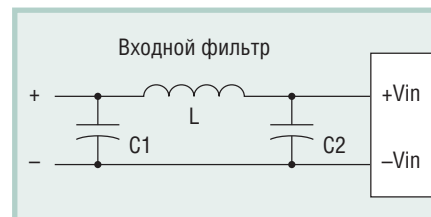
Рис. 2. Схема включения внешнего входного фильтра для преобразователей серии JCA
