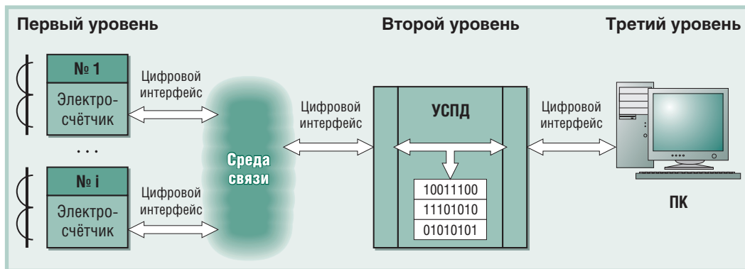
Рис. 2. Типовая структурная схема цифровой АСКУЭ
