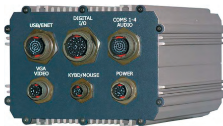
Рис. 4. Компьютер RMB в исполнении MIL-CORE™
