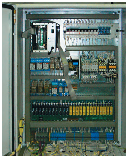
Рис. 4. Шкаф управления
