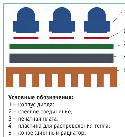
Рис. 3. Схема монтажа элементов светодиодной подсветки
