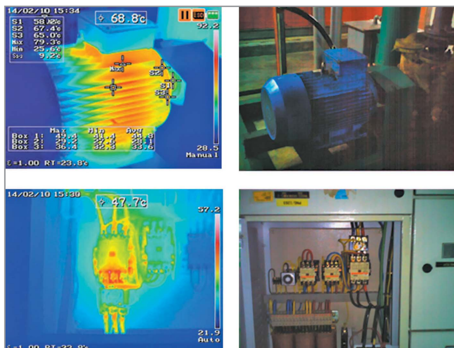
Рис. 1. Тепловые изображения (термограммы) и визуальные изображения электрических систем
