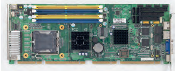
Рис. 4. Процессорная плата стандарта PICMG 1.3 Advantech PCE-5120
