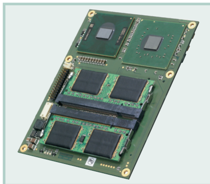
Рис. 2. Внешний вид одноплатного компьютерного модуля Toucan фирмы Lippert (формат COM Express, процессор Intel Core Duo)
