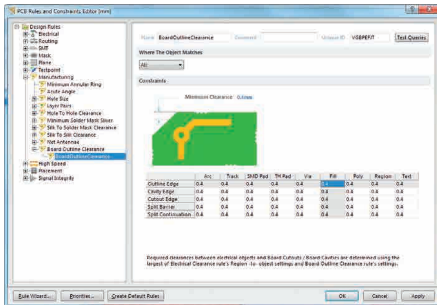
Рис. 36. Управление отступом полигональных объектов от краёв печатной платы
