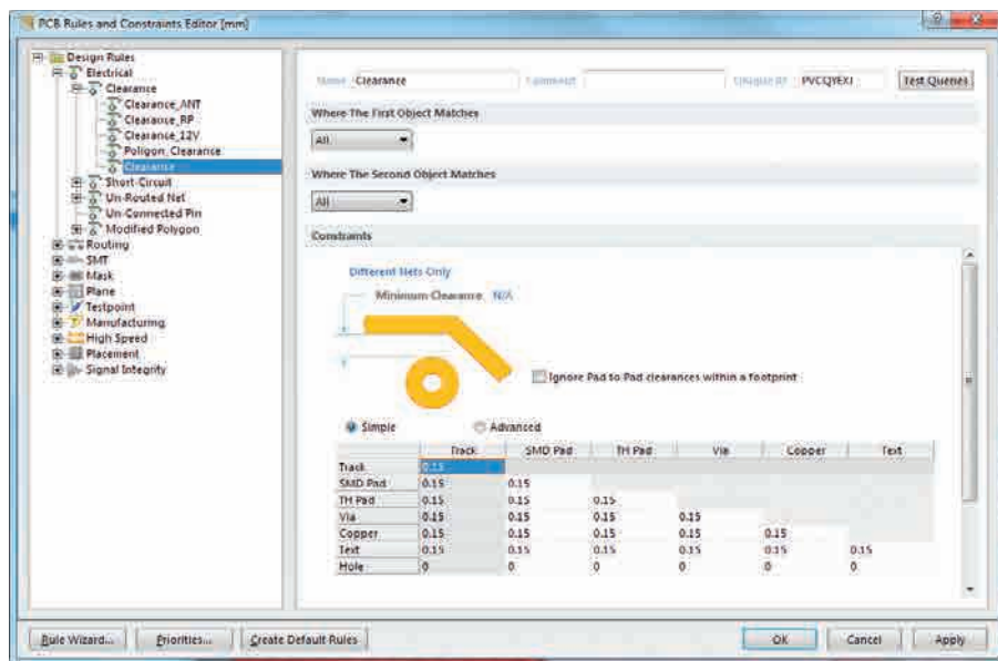
Рис. 34. Управление зазорами полигональных объектов с помощью правила Clearance
