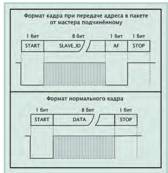
Рис. 7. Форматы кадров FBUS
