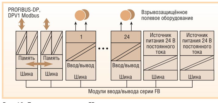
Рис. 10. Подстанция системы FB с резервированными коммуникационным модулем и модулем питания
