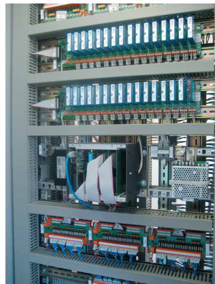
Рис. 5. Контроллер MicroPC установлен в каждом шкафу САУ ГСП
