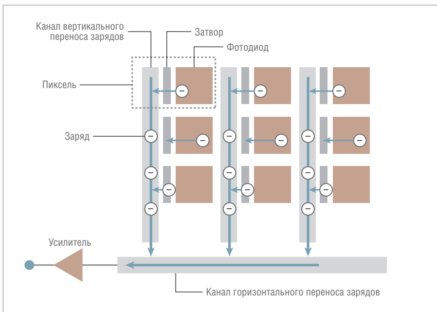
Рис. 1. Структура ССD-матрицы
