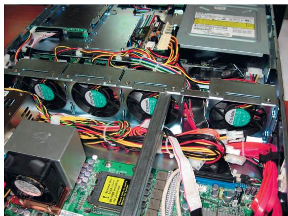
Рис. 3. Размещение жгутов проводов внутри промышленного сервера
