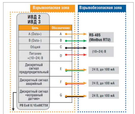
Рис. 5. Схема подключения датчиков с дискретным выходом
