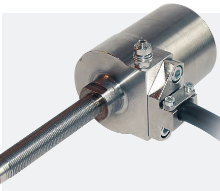
Рис. 1. Цифровой вибродатчик ИВД-2
