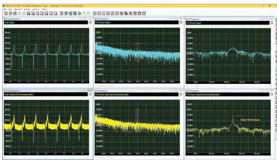
Рис. 5. Добавление интерферирующего сигнала 50 Гц к холтеровскому сигналу канала 1
