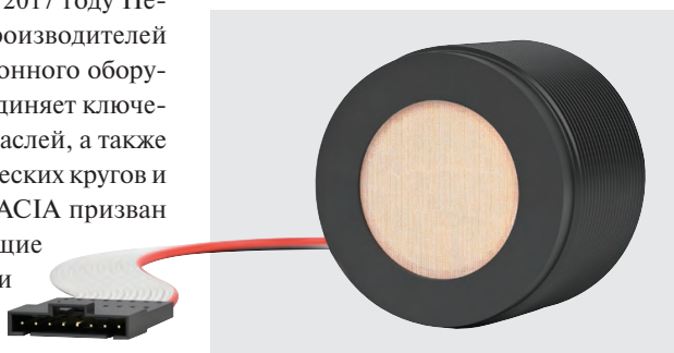
Рис. 3. Ультразвуковой датчик P+F UCC*-50GK для беспроводных систем контроля
