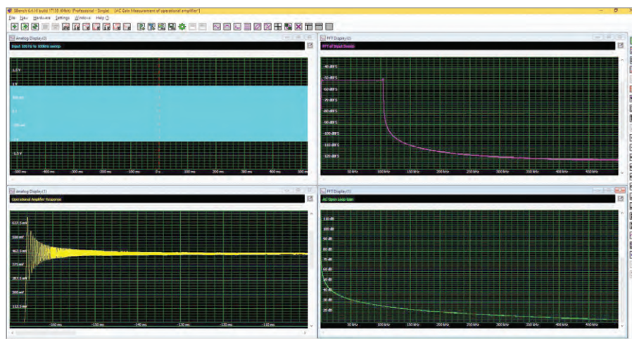
Рис. 3. Генерация сигнала (вверху слева), проверка частотного диапазона входного сигнала (вверху справа), получение выходного сигнала (внизу слева), построение частотной характеристики (внизу справа)
