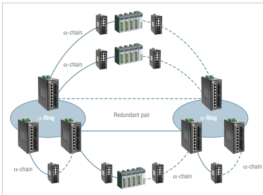
Рис. 11. Вариант использования нескольких протоколов резервирования от EtherWAN
