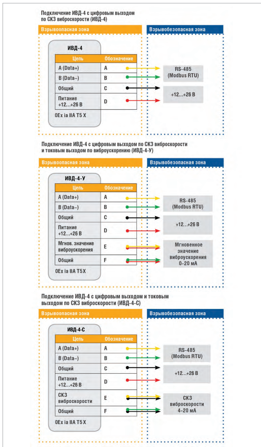
Рис. 9. Схемы подключения датчиков ИВД-4
