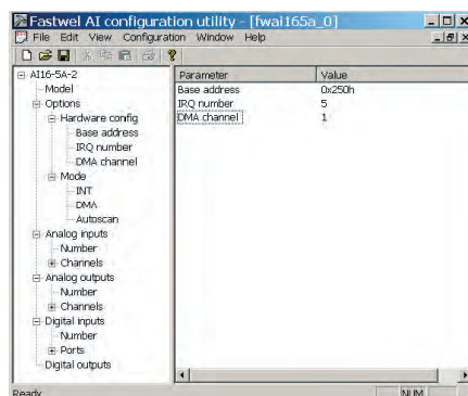
Рис. 3. FWAI CFG устанавливает параметры модуля ввода-вывода и сохраняет настройки в файл, который читается аппаратным драйвером при старте операционной системы
