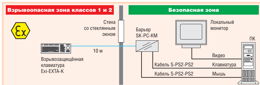
Рис. 15. Подключение клавиатур серии TASTEX к системе на основе ПК через барьер искробезопасности SK-PC-KM: система установлена во взрывобезопасной зоне, отделенной от взрывоопасной зоны стеной со стеклянным окном
