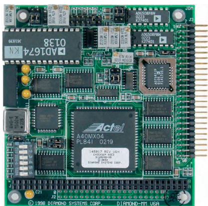
Рис. 2. Плата ввода-вывода DMM-NA-XT
