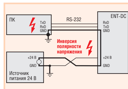
Рис. 11. Изменение полярности напряжения источника питания — причина выхода из строя ПК и ENT-DC
