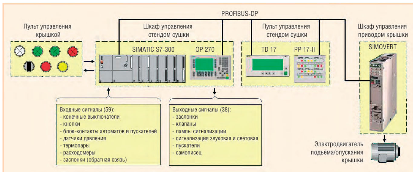
Рис. 3. Структурная схема системы управления станком сушки сталеразливочных ковшей
