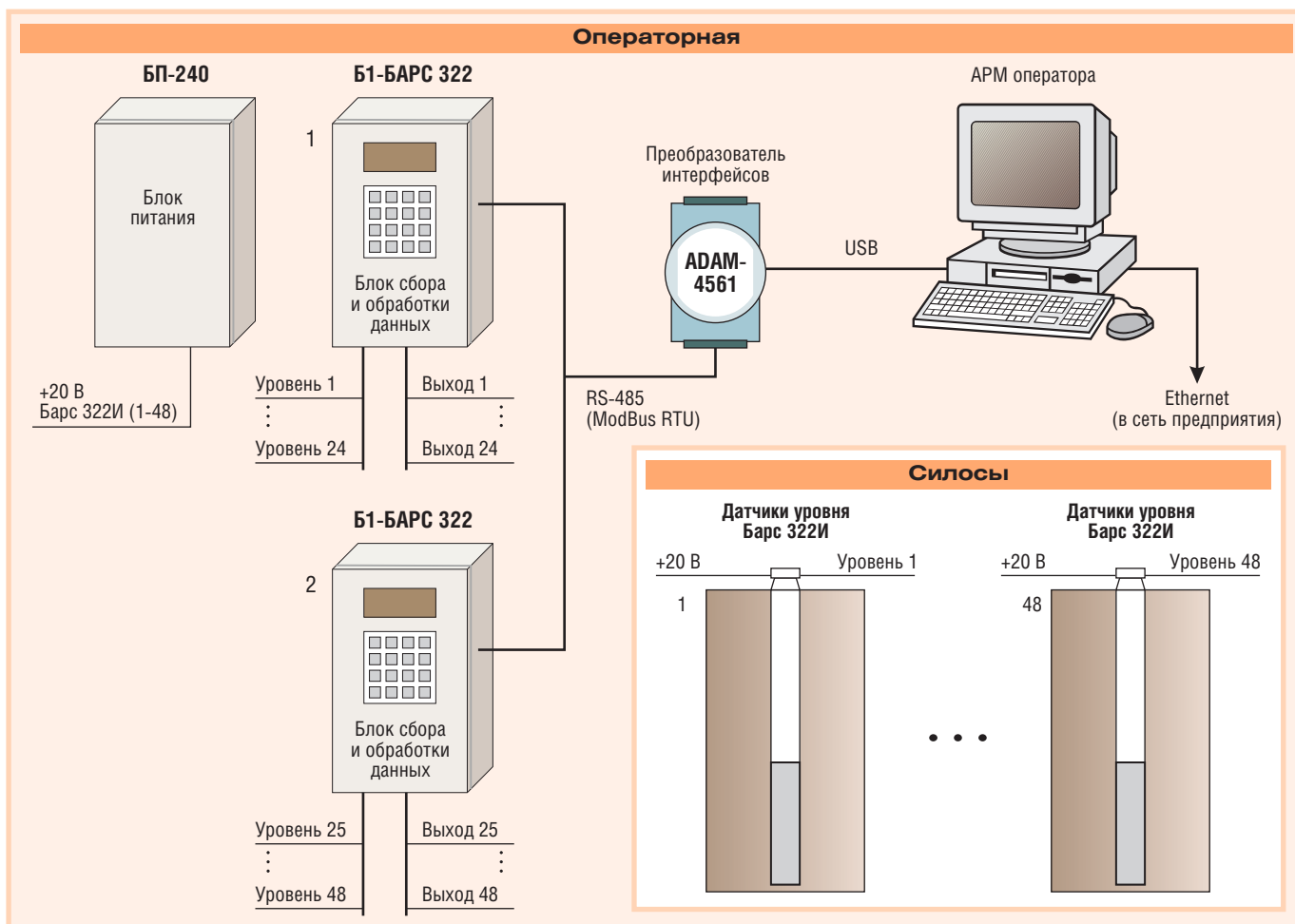
Рис. 4. Структурная схема АСК «Цемент-Завод»
