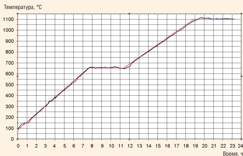
Рис. 9. График сушки сталеразливочного ковша в автоматическом режиме
