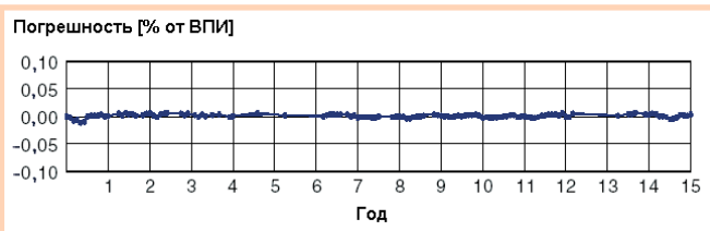
Рис. 3. Реальная погрешность показаний тестовых датчиков в течение 15 лет
