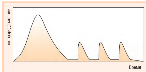
Рис. 14. Типовая форма импульса тока при разряде молнии [3]
