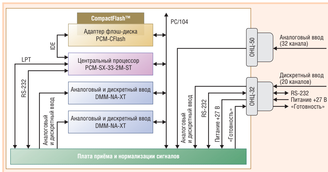
Рис. 3. Блок-схема устройства
