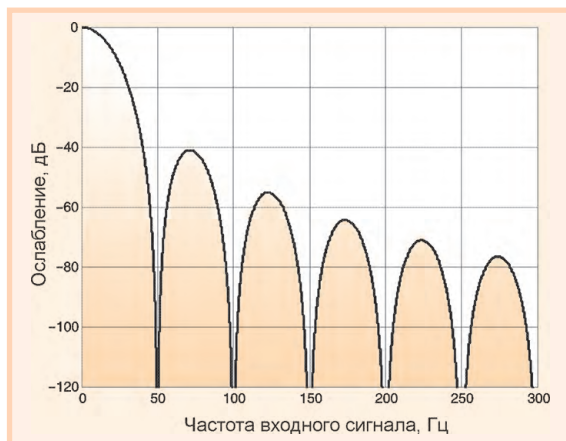
Рис. 9. АЧХ \text{SINC}^3 фильтра, входящего в состав аналоговых модулей NL
