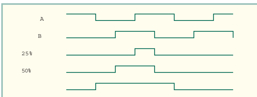
Рис. 16. Обработка квадратурных сигналов
