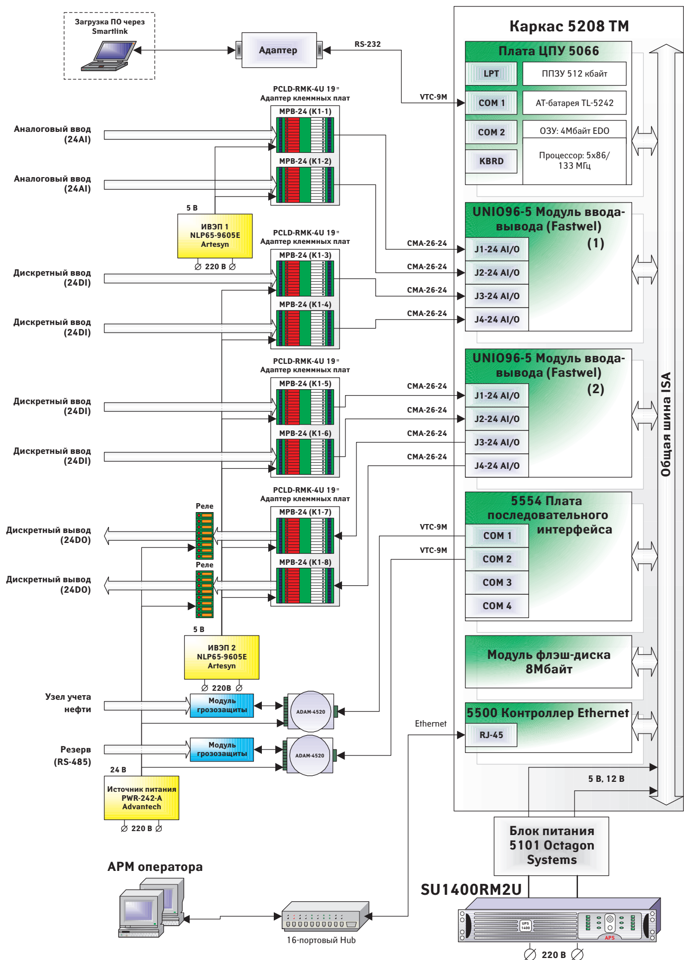
Рис. 7. Контроллер на базе MicroPC
