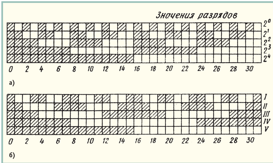
Рис. 2. Примеры кодирующих линейчатых масок: а — двоично-кодированная маска; б — маска в коде Грея
