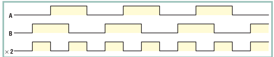
Рис. 8 б. Увеличение разрешающей способности в 2 раза
