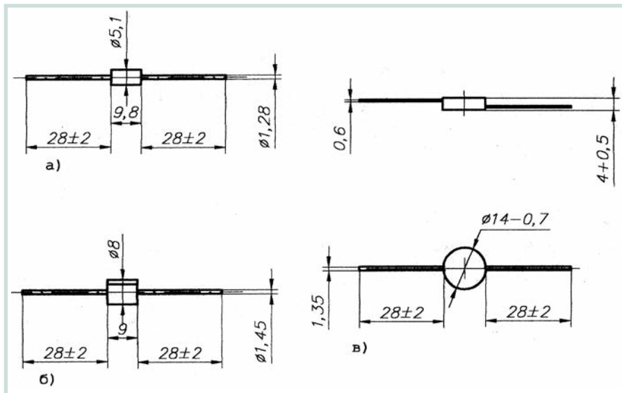
Рис. 7. Корпуса ПОН:
