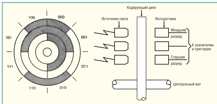
Рис. 5. Кодированный диск для генерации 3-разрядного кода Грея и упрощённая схема абсолютного шифратора углового положения
