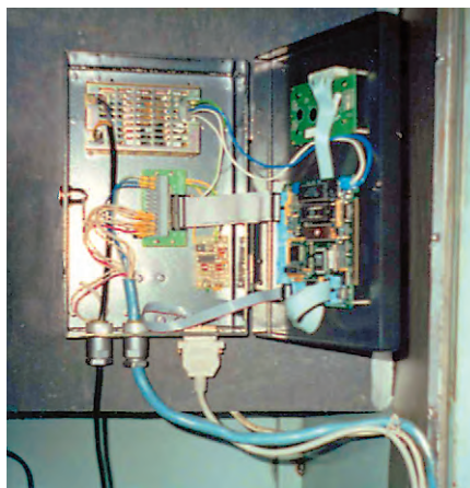
Рис. 2. Внутренняя конструкция вычислителя «ГАММА 055»
