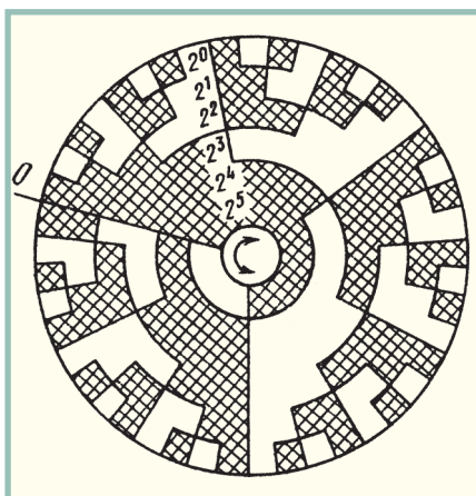
Рис. 3. Кодирующий диск
