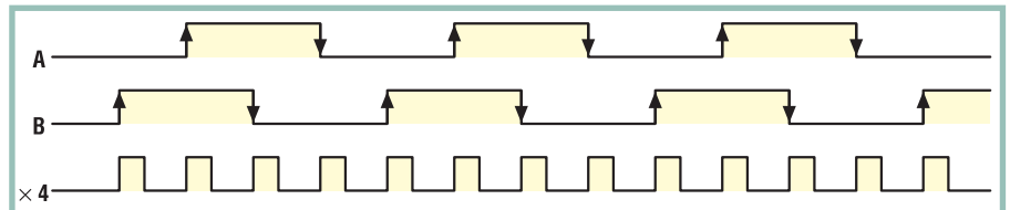
Рис. 8 в. Увеличение разрешающей способности в 4 раза
