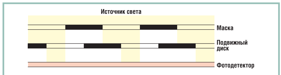
Рис. 9. В традиционном шифраторе приращений свет, до того как он достигнет диска шифратора, проходит через оптическую маску; так как диск вращается, фотодетектор получает не больше половины начальной засветки через каждую прорезь диска
