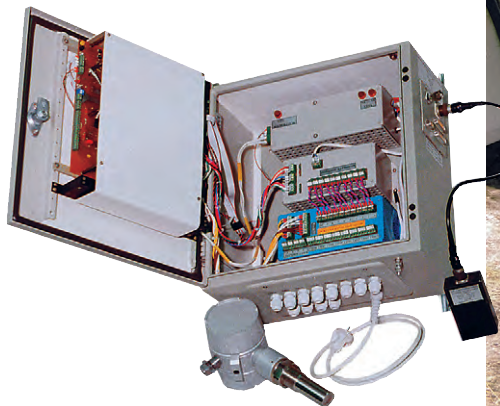
Рис. 9. Комплект аппаратуры ИИС «Поток-3М»
