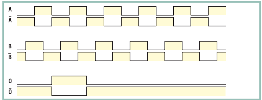
Рис. 8 а. Дифференциальные выходы шифратора
