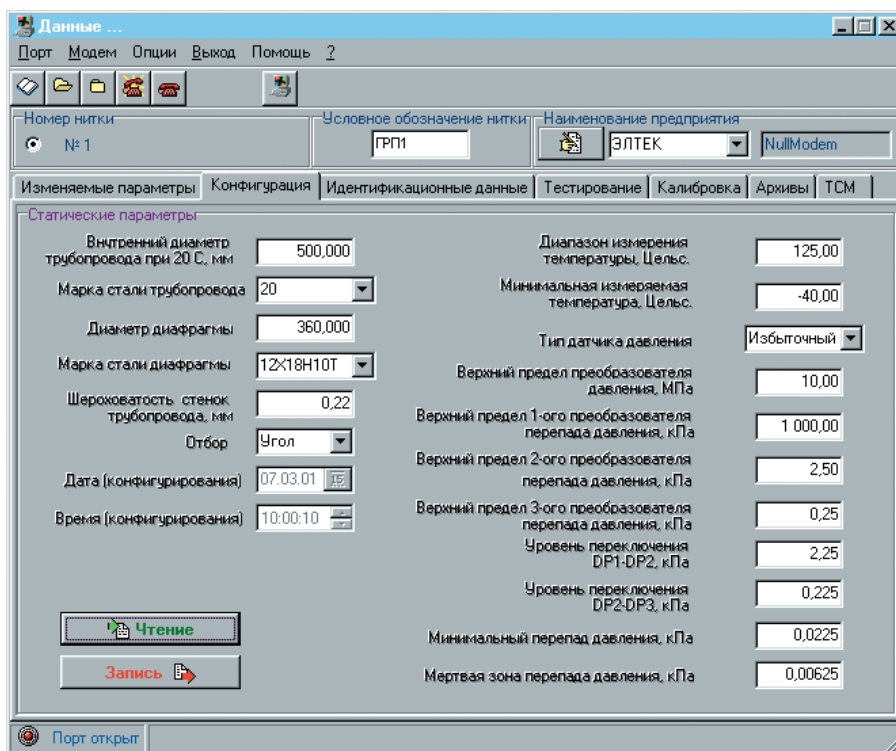
Рис. 5. Окно конфигурирования каналов АЦП вычислителя
