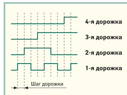
Рис. 6. Число дорожек зависит от разрешающей способности шифратора
