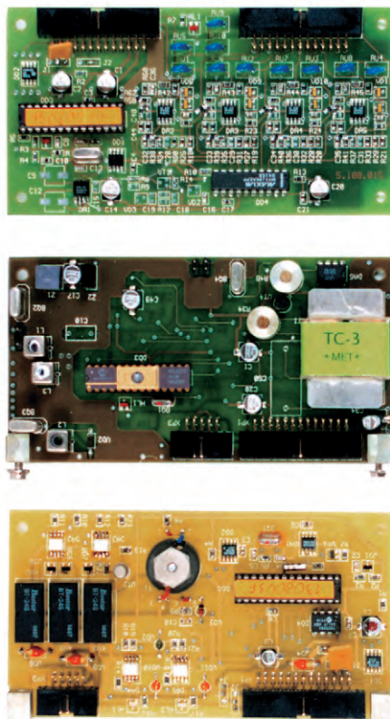
Рис. 8. Функциональные модули ИЗ, МЗ и СЗ (сверху вниз)
