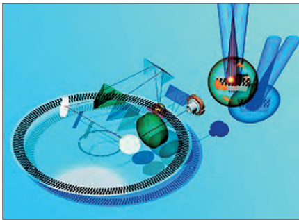
Рис. 11. Направления распространения света в шифраторе приращений
