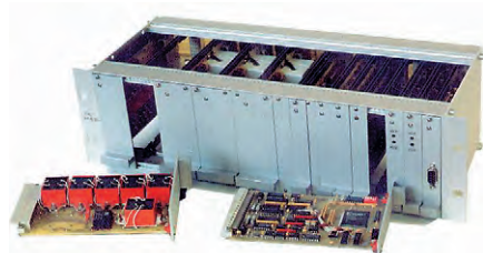
Рис. 5. Блок управления стрелкой (БУС)
