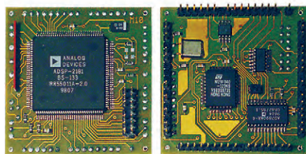
Рис. 8. Модуль аналого-цифровой обработки
