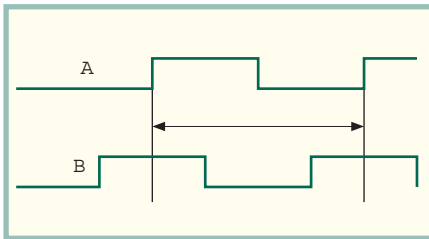
Рис. 15. Определение полного периода двухканального шифратора приращений
