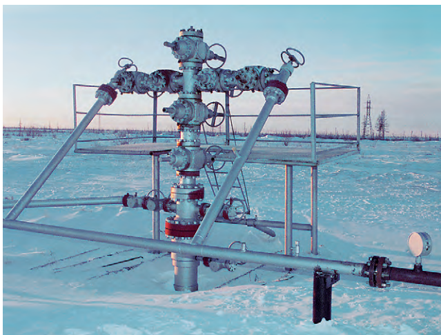
Рис. 1. Эксплуатационная скважина на промысле Нового Уренгоя
