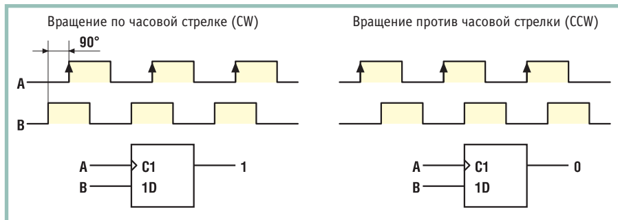
Рис. 7 б. Выходные сигналы двухканального шифратора
