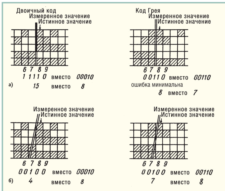
Рис. 4. Иллюстрация неоднозначности считывания кода с маски: а — при граничном положении считывающих элементов; б — при неверной юстировке элементов считывания кода
