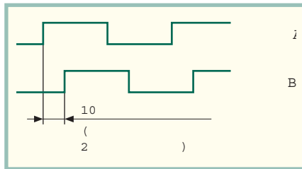
Рис. 13. Два сигнала, поступающих от фотодетектора, сфазированы так, что электронным управляющим устройством может быть обнаружено движение по часовой стрелке или против неё
