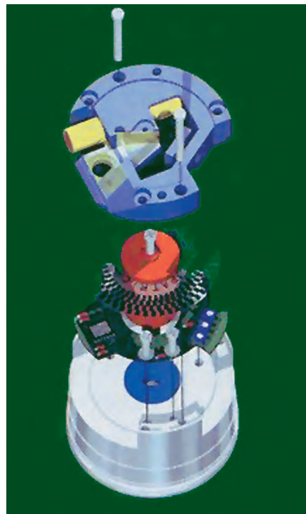
Рис. 10. Для обеспечения стабильности оптической системы все компоненты: светоделительная пластина, отражатели и источник света — установлены на прочном алюминиевом основании
