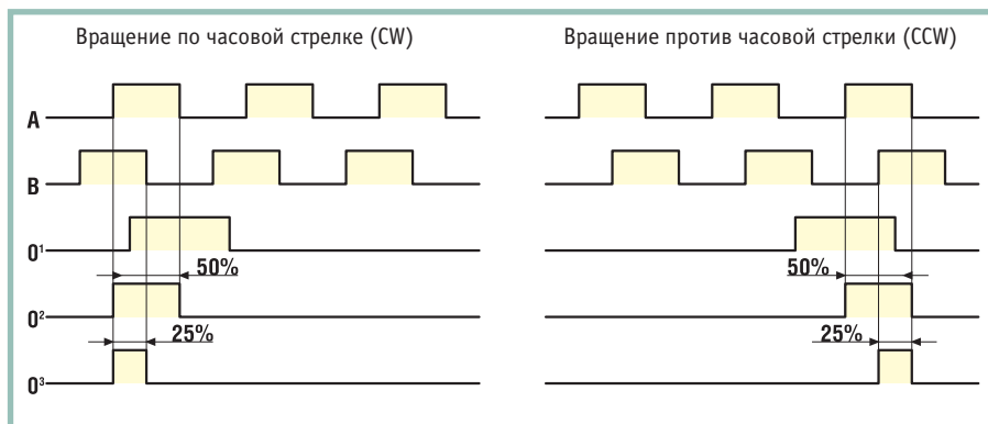
Рис. 7 в. Выходные сигналы и маркеры трёхканального шифратора
