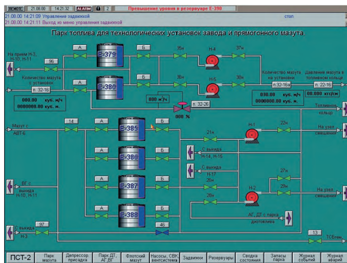
Рис. 10. Мнемосхема парка мазута
