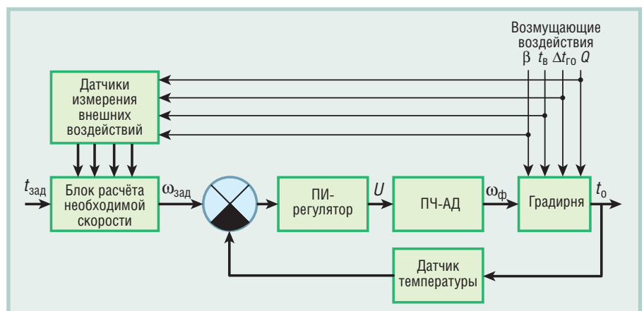
Условные обозначения: t_{зад} , t_o — температура охлажденной воды, заданная и фактическая соответственно; \omega_{зад} , \omega_{ф} — скорость вращения электропривода вентилятора, заданная и фактическая соответственно; \Delta t_{го} — перепад температур горячей/охлажденной воды; t_b — температура окружающего воздуха; \beta — влажность окружающего воздуха; Q — подача насоса; U — питающее напряжение; ПЧ-АД — система частотно-регулируемого электропривода «преобразователь частоты — асинхронный двигатель».
