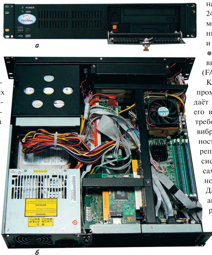
Рис. 2. Внешний вид конструкции шлюза: а — лицевая панель; б — вид сверху со снятой крышкой корпуса
