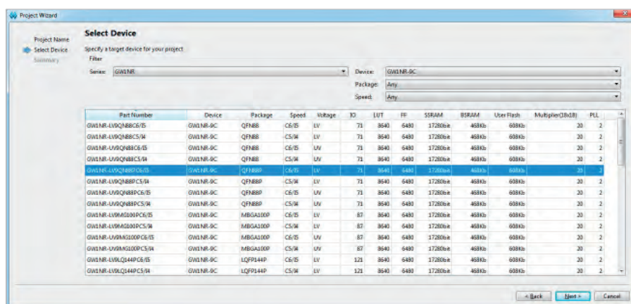
Рис. 4. Окно задания целевой ПЛИС
