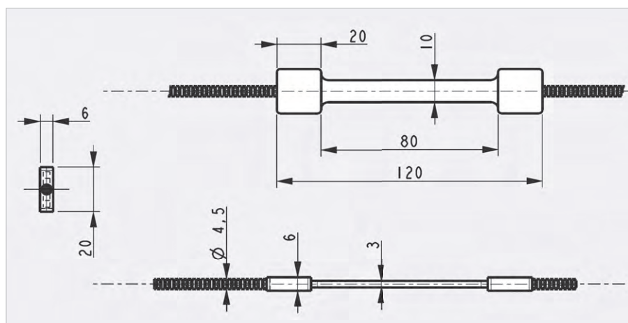
Рис. 5. Форм-фактор волоконно-оптического датчика детонации FT-OBSG-120-HT-FE-1117
