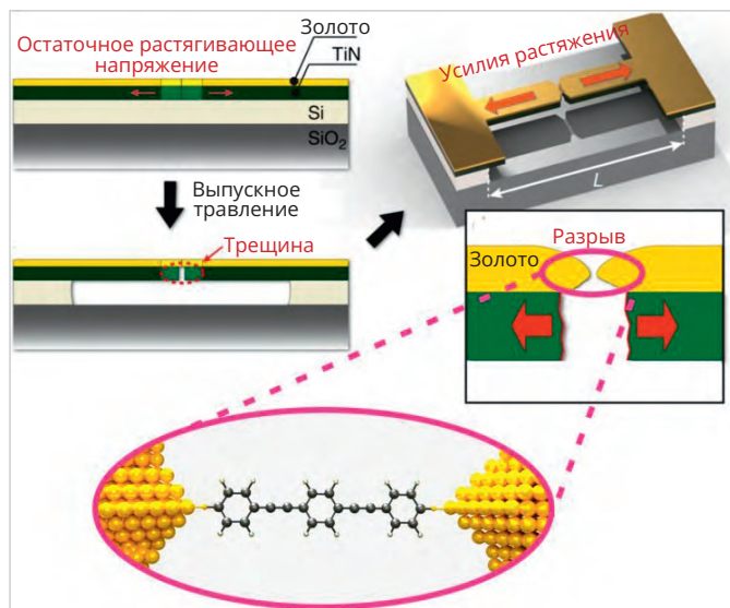
Рис. 5. Схема технологии изготовления металлических электродов для одномолекулярных устройств с помощью технологии [12]
