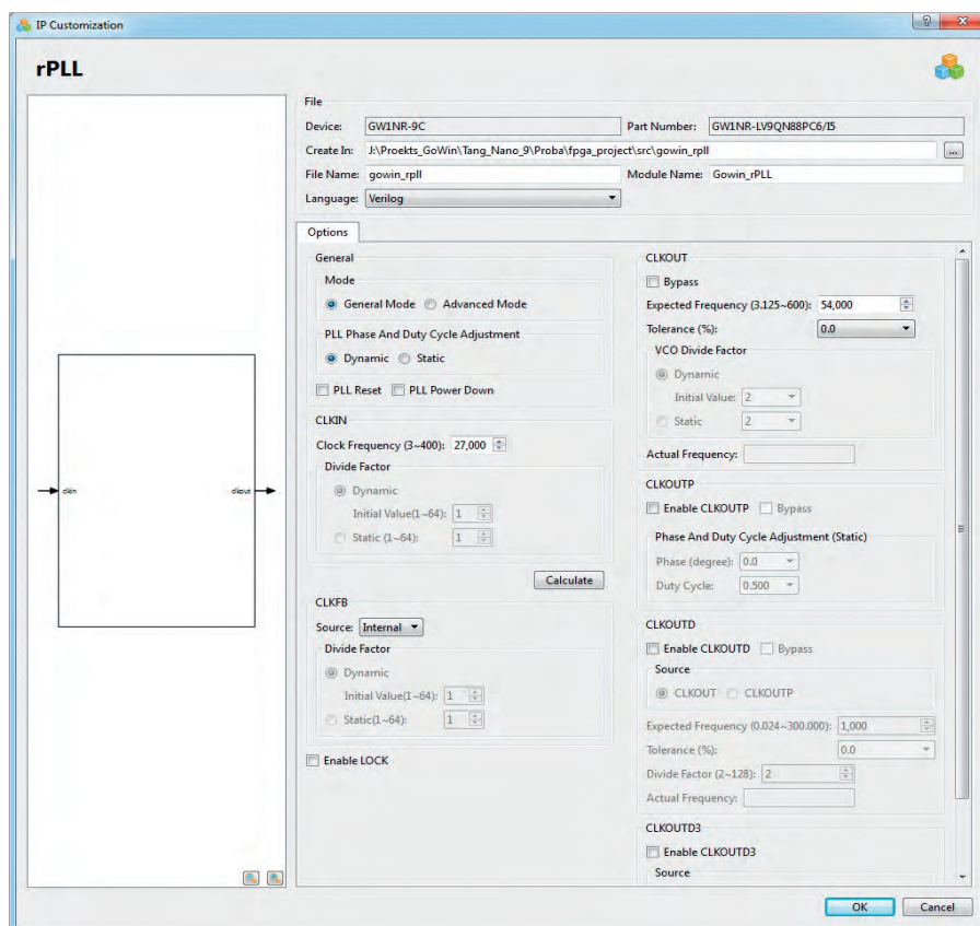
Рис. 16. Окно настройки параметров PLL
