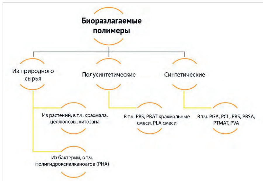
Рис. 5. Классификация биополимеров
