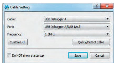
Рис. 22. Окно настройки загрузочного кабеля «Cable Setting»
