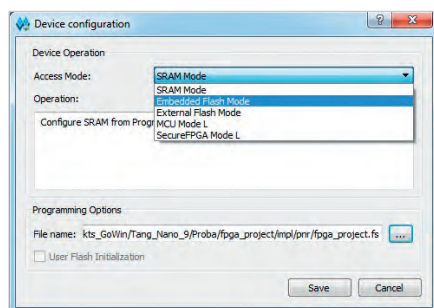
Рис. 23. Окно конфигурирования целевой ПЛИС
