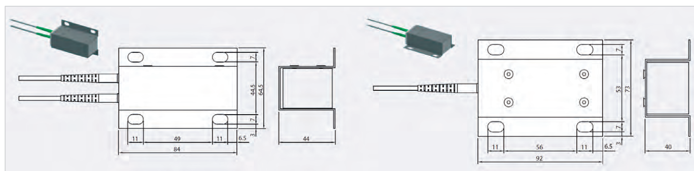
Рис. 6. Форм-фактор волоконно-оптического акселерометра ОБАС-002
