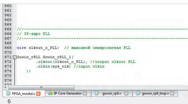
Рис. 17. а) файл шаблона модуля PLL; б) модуль PLL в качестве модуля нижнего уровня в проекте
