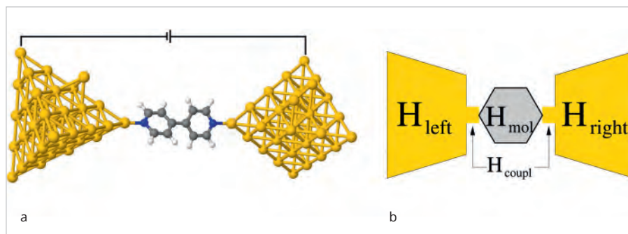
Рис. 10. а. Реальная структурная схема молекулярного мостика между металлическими проводниками и крепящими органическими якорями.
