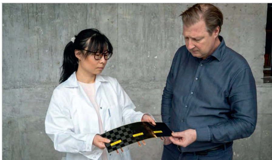
Рис. 16. Последовательно соединённые структурные батареи общим напряжением 8,4 В с модулем продольной упругости 28 ГПа.
