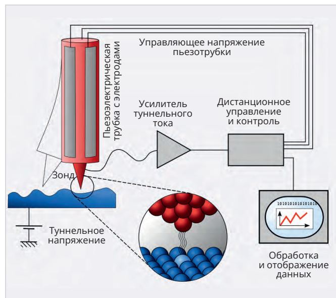
Рис. 6. Схема работы сканирующего туннельного микроскопа [13]
