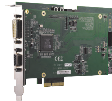
Рис. 11. Плата видеозахвата HDV62, поддерживающая формат Full HD
