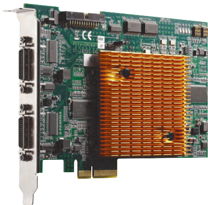
Рис. 6. PCIe-CPL64 – плата видеозахвата с интерфейсом PoCL
