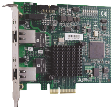
Рис. 8. PoE-плата видеозахвата PCIe-GIЕ62+
