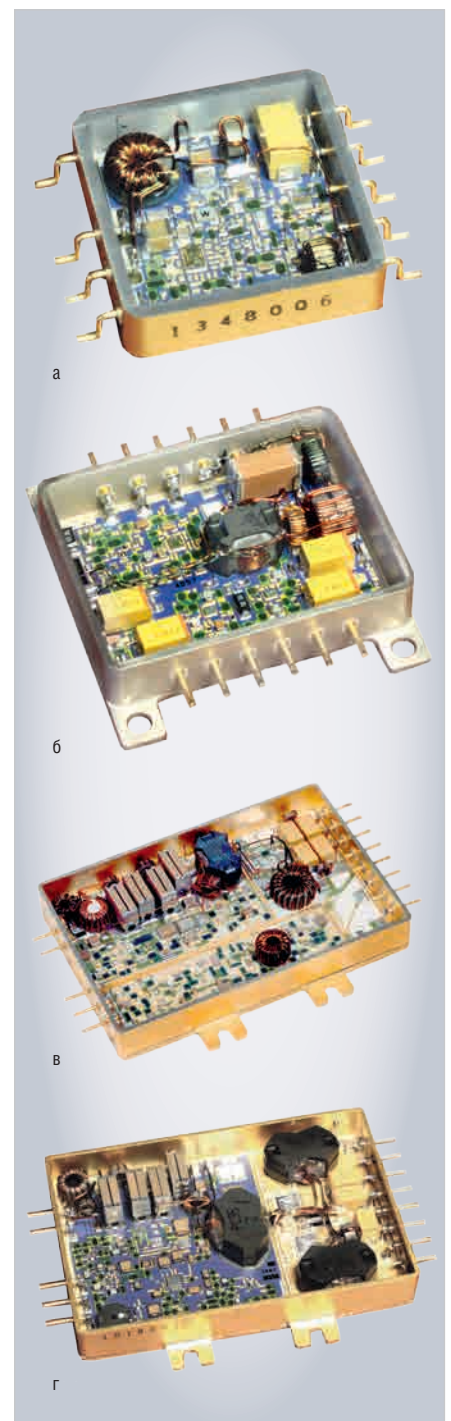
Рис. 3. Радиационно-стойкие модули DC/DC-преобразователей напряжения серий ARE (а), LA (б), M3N (в) и GHN (г)
