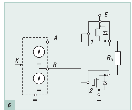
Рис. 10. Резервирование модулей вывода для повышения отказоустойчивости и живучести (а) и для реализации аварийного отключения (б)
