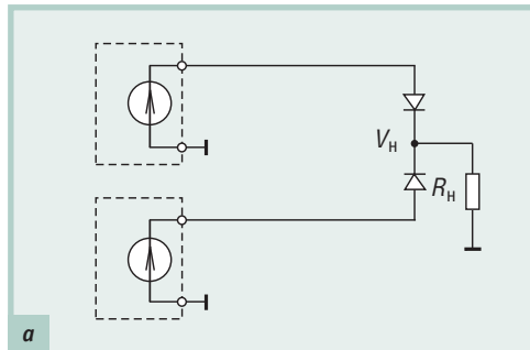
Рис. 9. Соединение дискретных выходов при резервировании (а) и один из вариантов реализации дискретных выходных каскадов (б)
