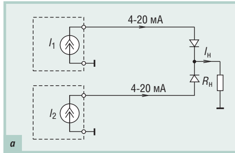
Рис. 8. Резервирование (а) и диагностика (б) линии вывода аналоговых сигналов
