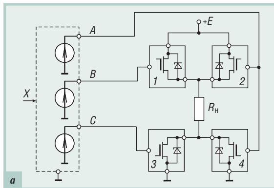
Рис. 10. Резервирование модулей вывода для повышения отказоустойчивости и живучести (а) и для реализации аварийного отключения (б)
