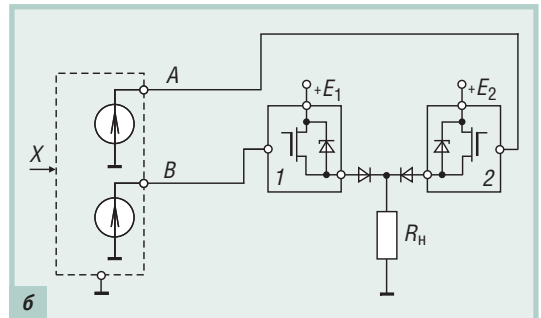
Рис. 9. Соединение дискретных выходов при резервировании (а) и один из вариантов реализации дискретных выходных каскадов (б)
