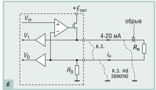
Рис. 8. Резервирование (а) и диагностика (б) линии вывода аналоговых сигналов
