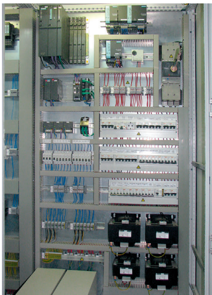
Рис. 6. Шкаф контроллера
