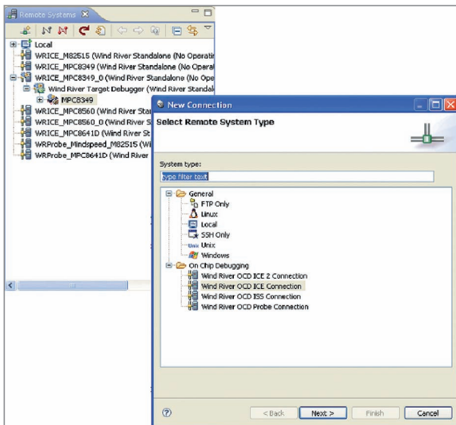
Рис. 9. Администратор соединений упрощает подключение к нескольким ядрам одновременно и поддерживает множество типов соединений
