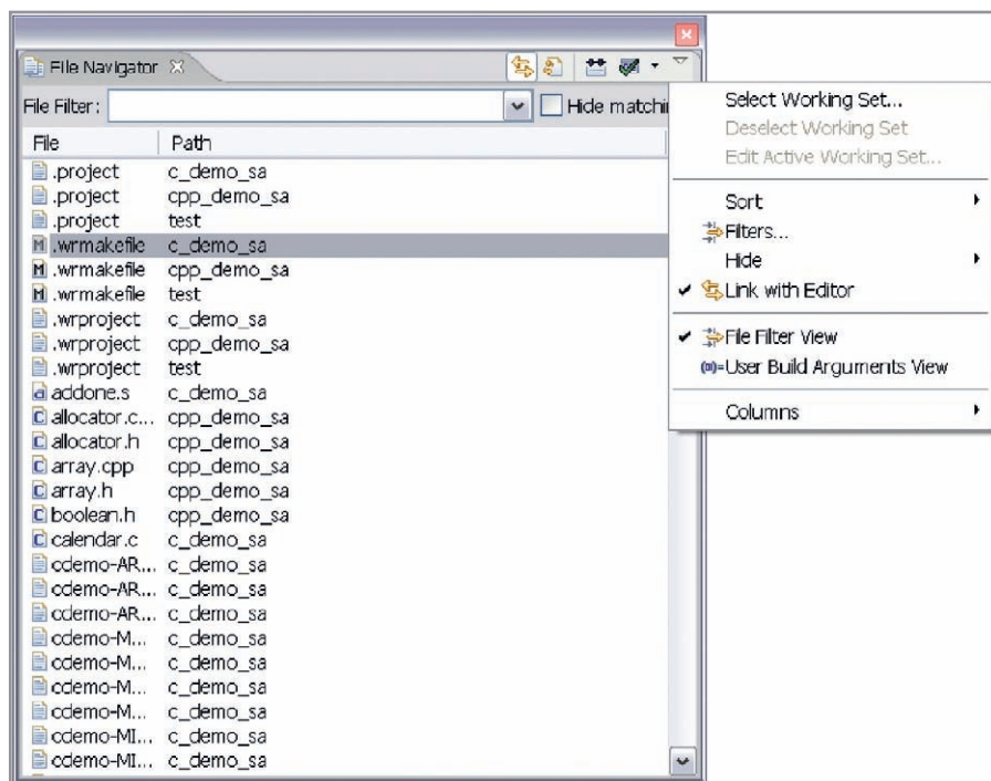
Рис. 5. Навигатор Workbench позволяет быстро искать идентификаторы
