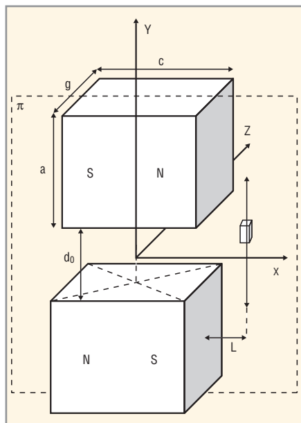
Рис. 2. Магнитная система из двух магнитов типа «магнитный репер»
