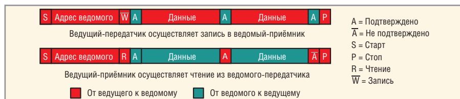
Рис. 3. Переключение между режимами передачи и приема во время пересылки данных
