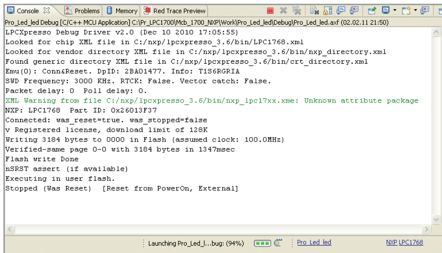
Рис. 12. Информация о действиях, производимых LPCXpresso IDE и отладчиком LPC-Link над приложением и целевым МК при переходе в режим отладки
