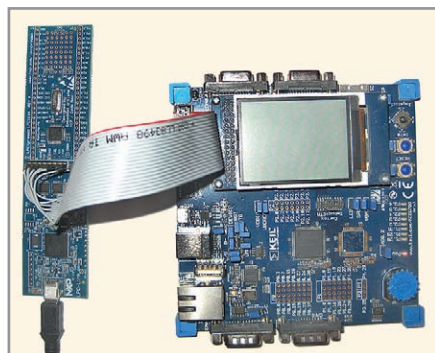
Рис. 11. Подключение демонстрационной платы LPCXpresso к отладочной плате MCB1760 через JTAG
