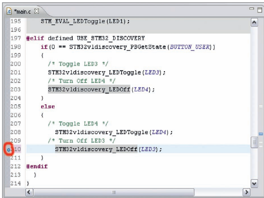
Рис. 13. Установка точки останова
