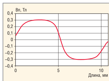
Рис. 4. Распределение нормальной составляющей индукции магнитного поля B_n магнитной системы из двух магнитов при a = c = 5,0 мм; d_0 = 0,0 мм; \Delta = 0,1 мм и L = 0,5 мм; магниты марки \text{SmCo}_5 20MG0e
