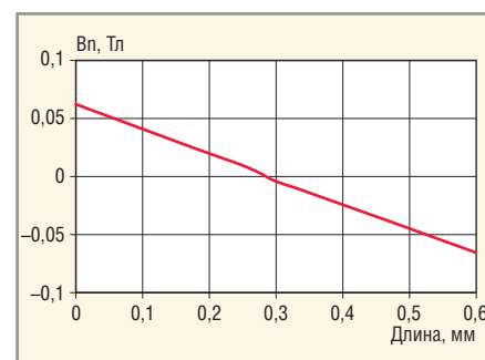
Рис. 5. Распределение нормальной составляющей индукции магнитного поля B_n репера вблизи смены полюсов магнитов при a = c = 5,0 мм; d_0 = 0,0 мм; \Delta = 0,1 мм и L = 1,0 мм; магниты марки \text{SmCo}_5 20MG0e
