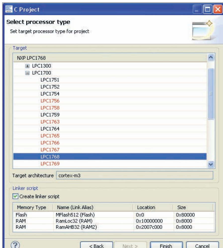
Рис. 7. Диалоговое окно выбора МК целевой системы проекта Select processor type
