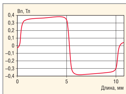
Рис. 3. Распределение нормальной составляющей индукции магнитного поля B_n магнитной системы из двух магнитов при a = c = 5,0 мм; d_0 = 0,0 мм; \Delta = 0,1 мм и L = 0,0 мм; магниты марки \text{SmCo}_5 20MG0e
