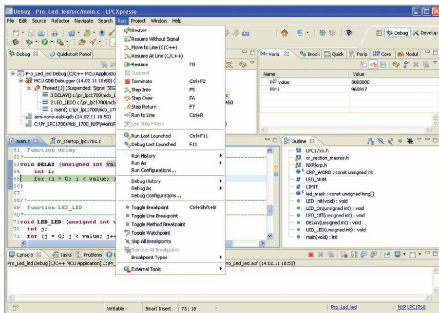
Рис. 13. Главное окно перспективы Debug в режиме отладки
