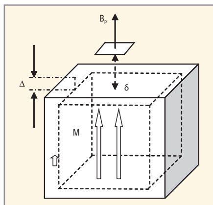
Рис. 1. Модель магнита с учётом дефектной поверхности
