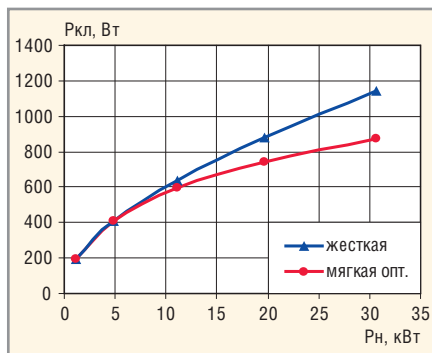
Рис. 4. Зависимость суммарной мощности потерь P_{\text{кл}} в ключевых элементах инвертора от выходной мощности нагрузки P_n при жёсткой и мягкой коммутации при слежении за пороговым током
