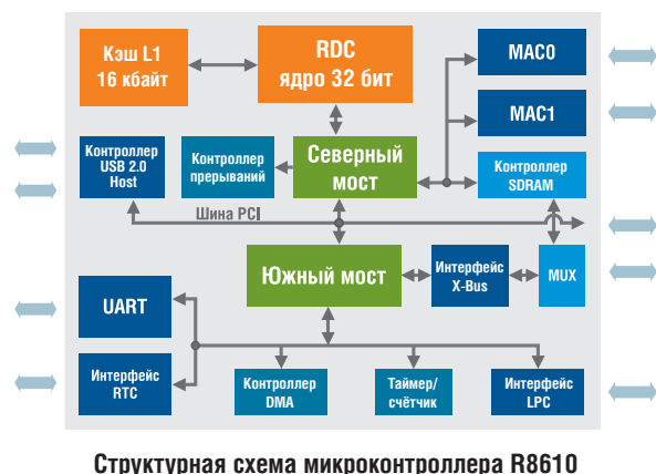
Структурная схема микроконтроллера R8610
