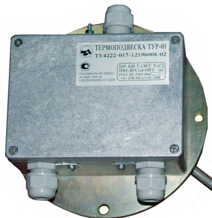
Рис. 4. Термоподвеска ТУР-01
