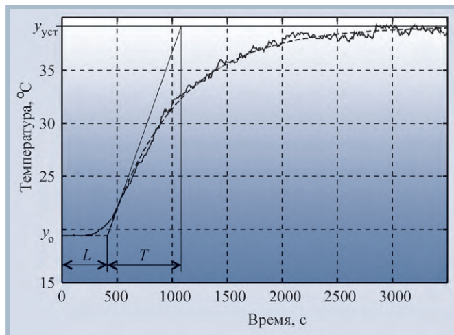
Рис. 24. Температура трубы отопления здания после включения клапана подачи теплоносителя (аппроксимация моделью первого порядка)
