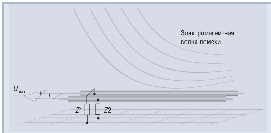
Рис. 5. Воздействие электромагнитной волны помехи на витую пару
