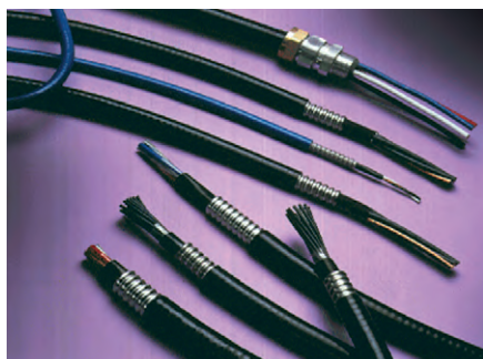
Рис. 18. Бронированные кабели
