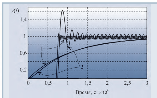
Рис. 35. Сравнение различий между переходными характеристиками и колебаниями в двух системах второго порядка с параметрами T_1 = 10,9 , T_2 = 0,1 , L = 0,02 (кривые 1) и T_1 = 10 , T_2 = 1 , L = 0,02 (кривые 2)
