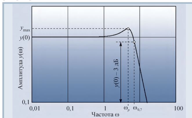
Рис. 20. Критерии качества регулирования в частотной области
