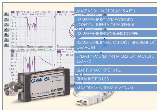
Рис. 2. Векторные рефлектометры
