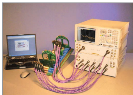
Рис. 2. Измерительный комплекс Agilent U3025AE10
