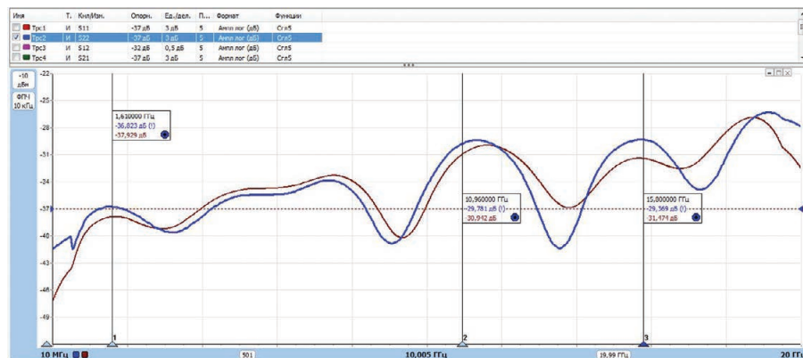
Рис. 14. Графики возвратных потерь коаксиального аттенюатора с ослаблением 30 дБ (тракт 3,5 мм)
