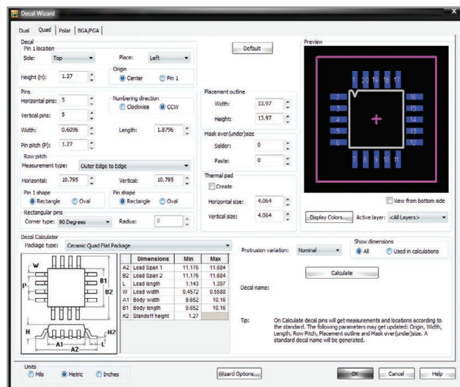
Рис. 6. Вкладка Quad мастера PM Decal Wizard
