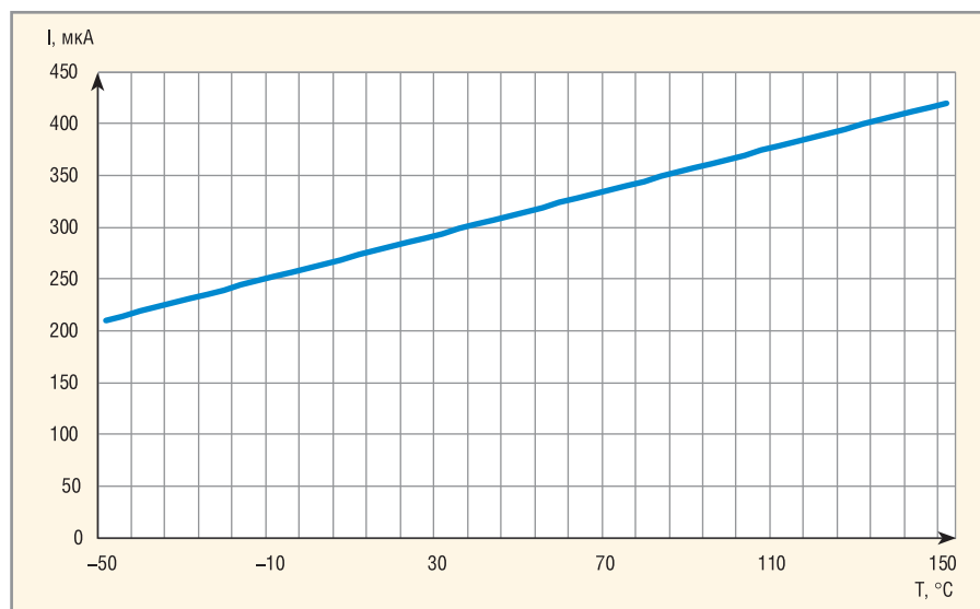
Рис. 2. Зависимость выходного тока микросхемы 1019ЧТЗС от температуры
