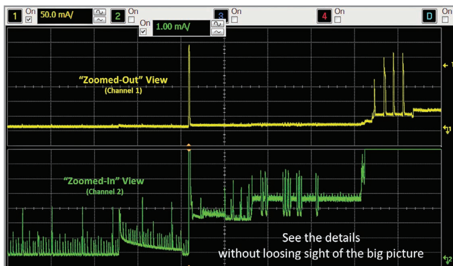
Рис. 2. Осциллограммы тока мобильного телефона, измеренные с помощью пробника N2820A.
