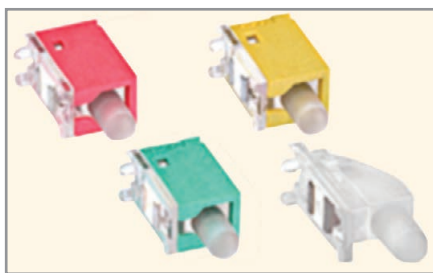
Рис. 6. Светопроводниковые компоненты M-PIPE
