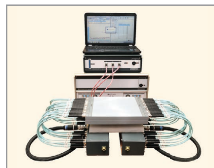
Рис. 8. Внешний вид комплекса К2М-102, скоммутированного для калибровки
