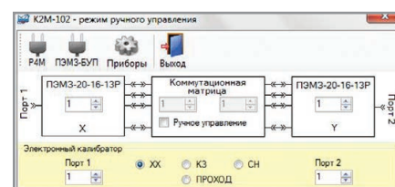
Рис. 10. Окно работы для ручного режима
