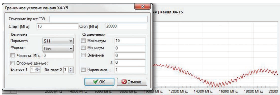
Рис. 13. Окно установки граничных условий для отбраковки измеряемых устройств
