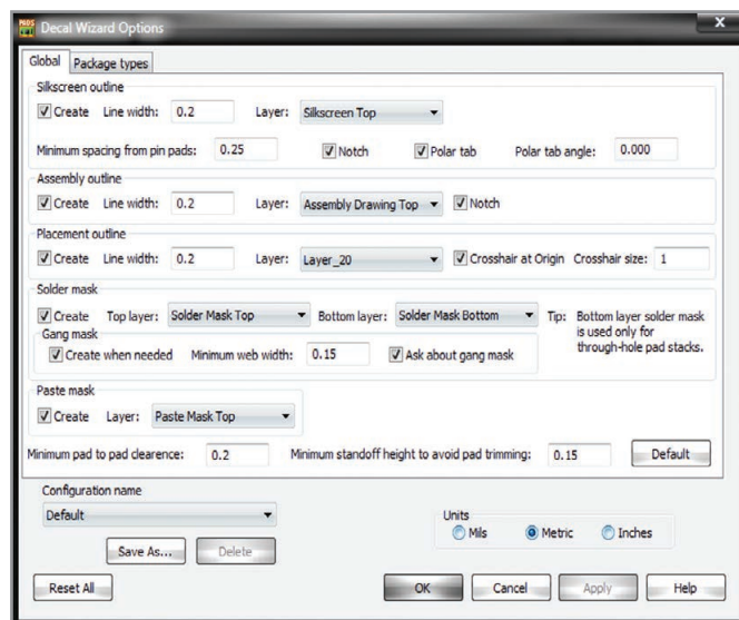
Рис. 4. Окно настроек мастера ПМ Decal Wizard Options
