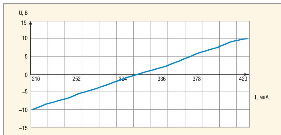
Рис. 5. Зависимость выходного напряжения модели от входного тока
