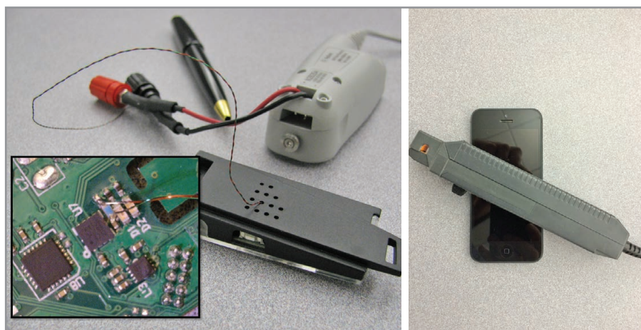
Рис. 3. Токовые клещи (слева) и токовый пробник с шунтом (справа)
