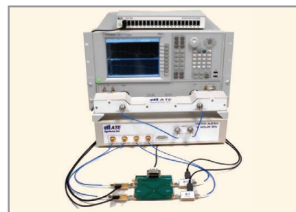
Рис. 4. Измерительный комплекс на основе расширителя портов от ATE Systems
