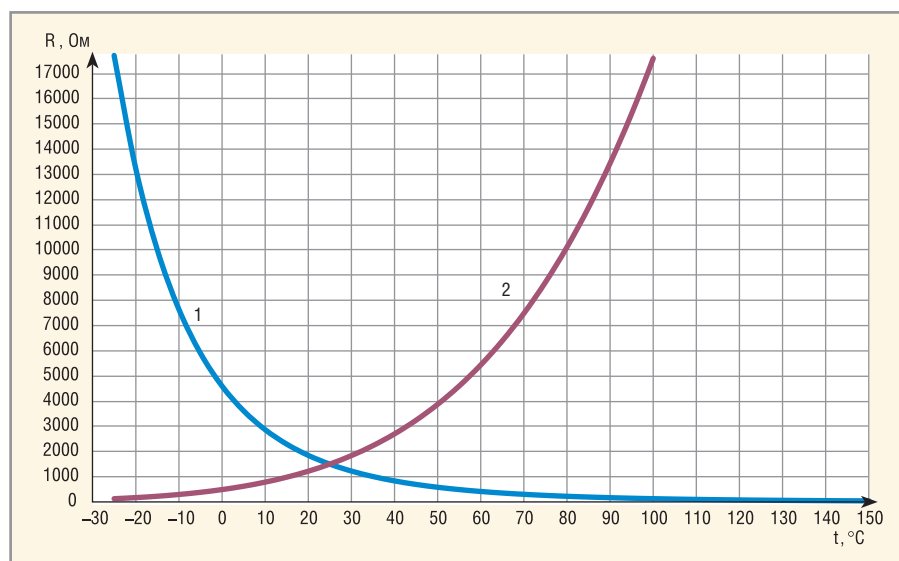
Рис. 1. Типовые графики температурной зависимости для различных терморезисторов: 1 – типа СТ, 2 – типа ТР
