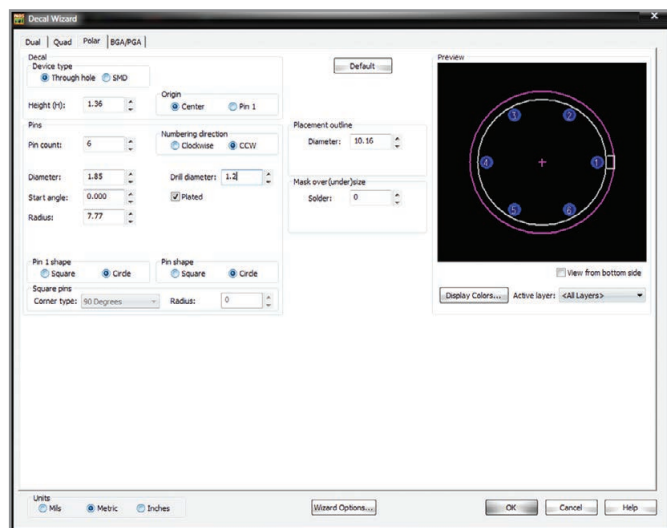
Рис. 7. Создание ПМ компонента со штыревыми выводами на вкладке Polar мастера PM Decal Wizard
