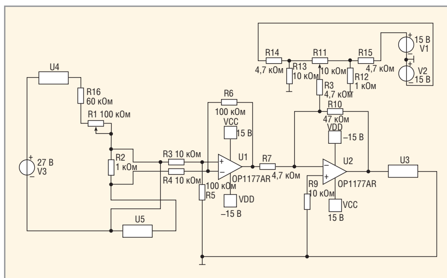
Рис. 4. Схема моделирования обработки выходного сигнала ИС 1019CT3C
