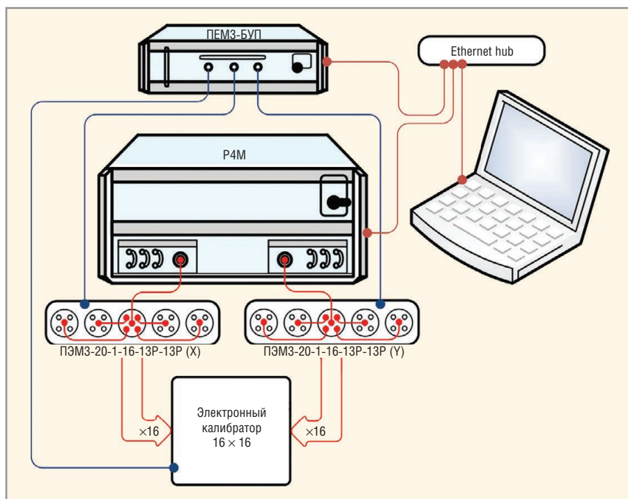
Рис. 5. Структурная схема комплекса K2M-102
