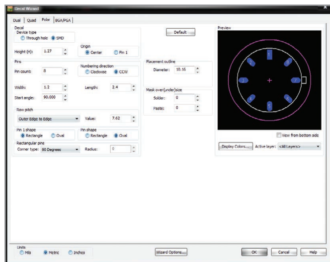
Рис. 8. Создание ПМ компонента с планарными выводами на вкладке Polar мастера PM Decal Wizard
