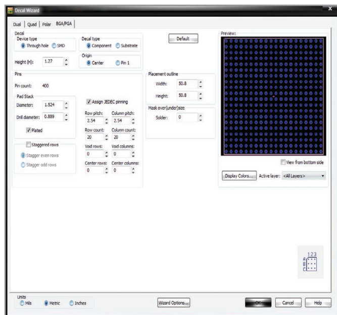
Рис. 9. Вкладка BGA/PGA мастера ПМ Decal Wizard
