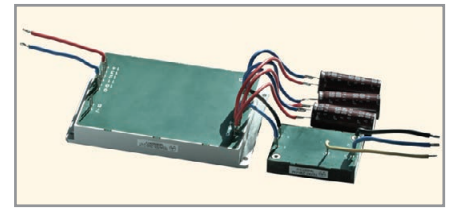
Рис. 4. Пример способа построения AC/DC-преобразователя с выносными конденсаторами
