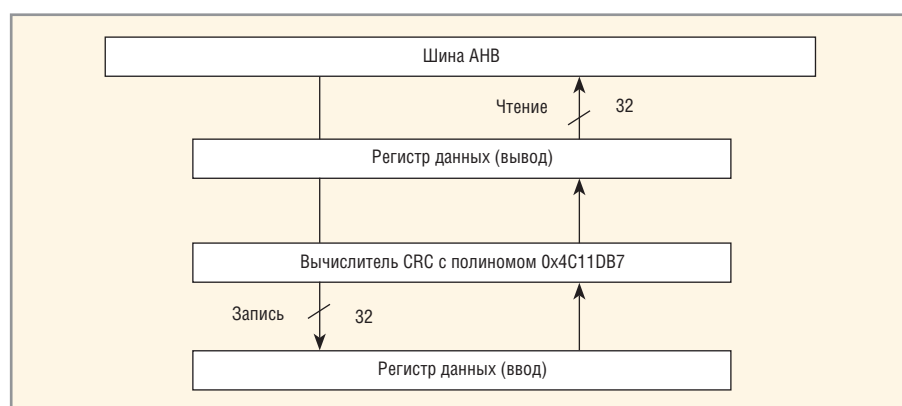
Блок-схема работы блока вычисления CRC
