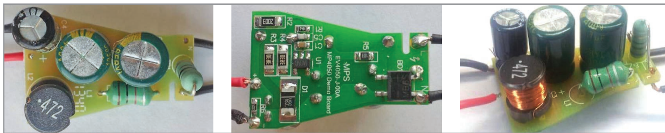
Рис. 2. Внешний вид светодиодного драйвера на базе микросхемы MP4050GJ (габаритные размеры 29 × 19 × 18 мм)
