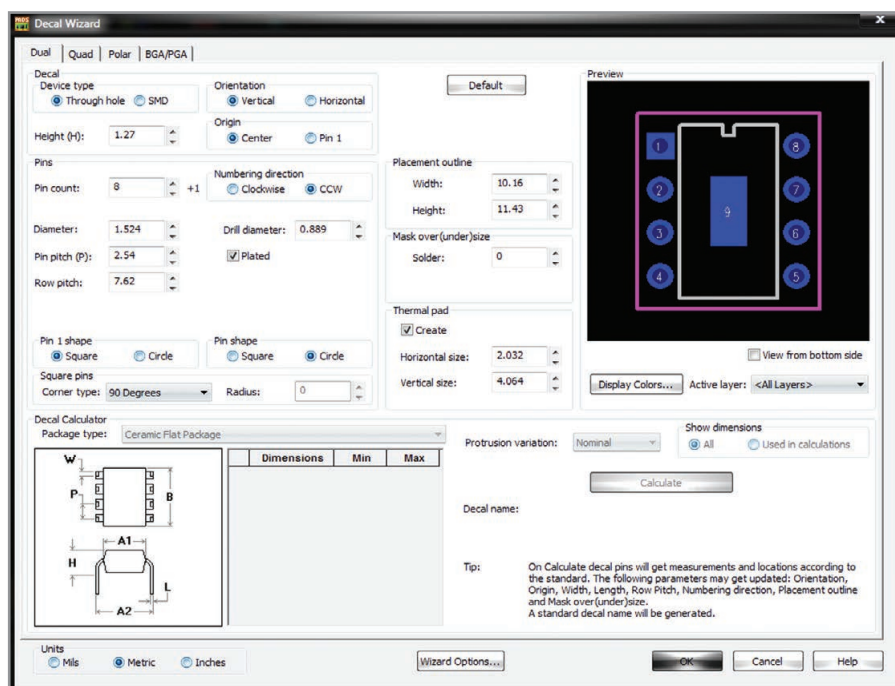
Рис. 2. Создание ПМ компонента со штыревыми выводами на вкладке Dual мастера ПМ Decal Wizard
