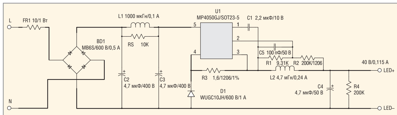
Рис. 1. Принципиальная схема светодиодного драйвера на базе микросхемы MP4050 от компании MPS
