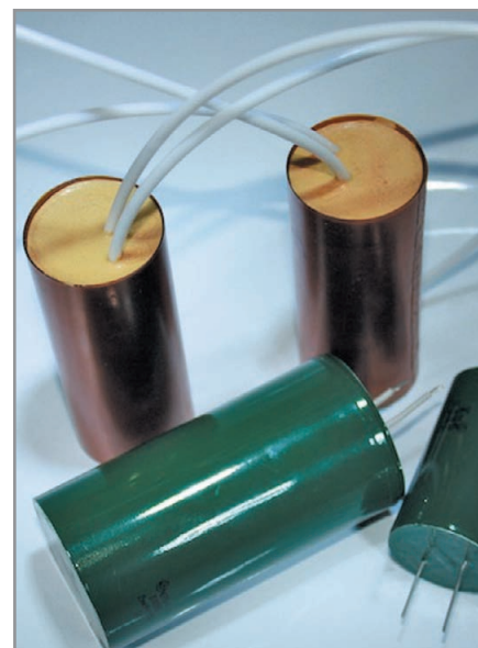
Высокотемпературный конденсатор К73-47
