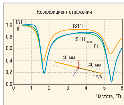
Рис. 3. Частотная характеристика вибраторной антенны, рассчитанная с учётом влияния частот антенны ( |S_{11\_корр}| ) и без учёта их влияния ( |S_{11}| ), а также коэффициент отражения \Gamma_1 , рассчитанный в однопортовой схеме
