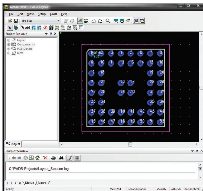
Рис. 10. Окно редактора Decal Editor
