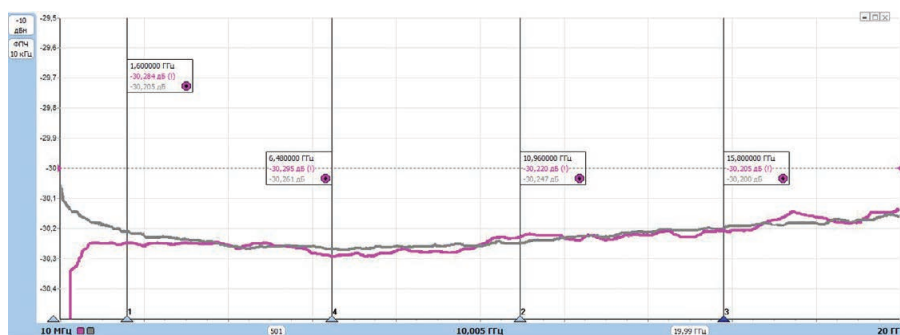
Рис. 15. Графики АЧХ коаксиального аттенюатора с ослаблением 30 дБ (тракт 3,5 мм)
