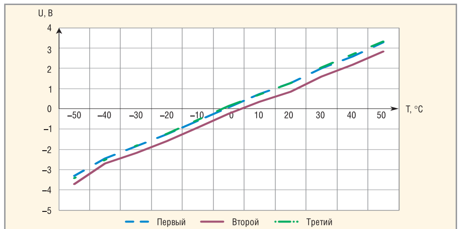
Рис. 9. Результаты натуральных испытаний трёх образцов микросхемы 1019ЧТЗС
