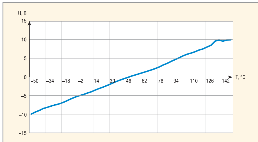
Рис. 6. Имитация зависимости выходного напряжения схемы моделирования от температуры
