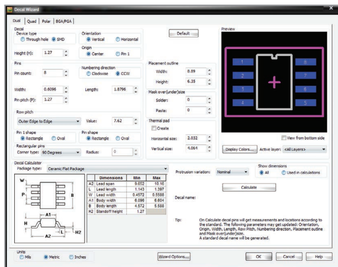
Рис. 5. Создание ПМ компонента с планарными выводами на вкладке Dual мастера PM Decal Wizard
