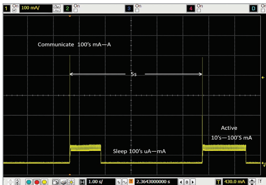
Рис. 1. Профиль тока типичного устройства с батарейным питанием (мобильный телефон в режиме ожидания и в режиме связи)
