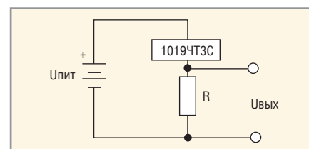
Рис. 3. Схема делителя напряжения – преобразователя тока в напряжение
