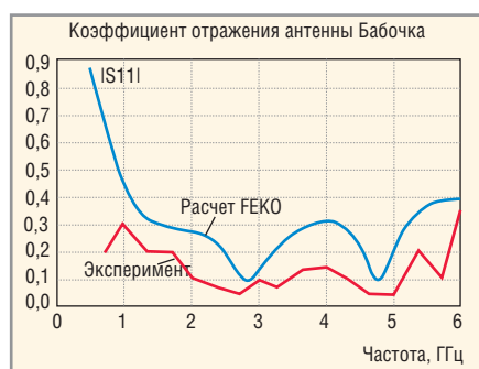
Рис. 6. Коэффициент отражения со стороны входного разъёма антенны «бабочка», отдельные вибраторы которой запитываются с помощью ИС
