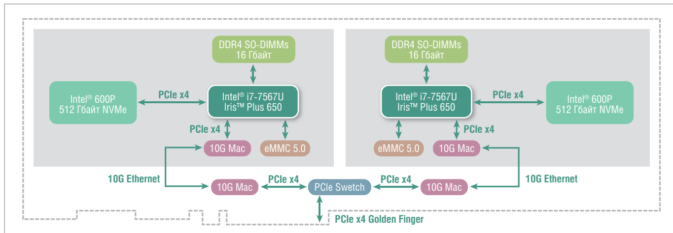
Рис. 2. Структура Mustang-200
