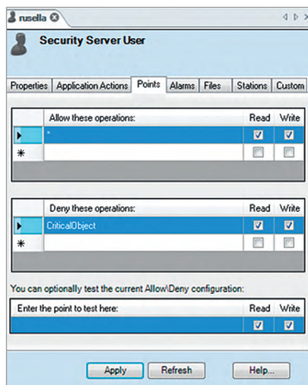
Рис. 3. Запрет доступа на чтение и запись точки CriticalObject
