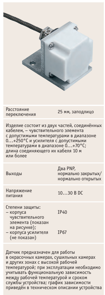
Рис. 16. Индуктивный датчик NCN25-F35-A2-250-V1 для рабочих зон с высокой температурой обнаруживает металлический объект в рабочей зоне датчика
