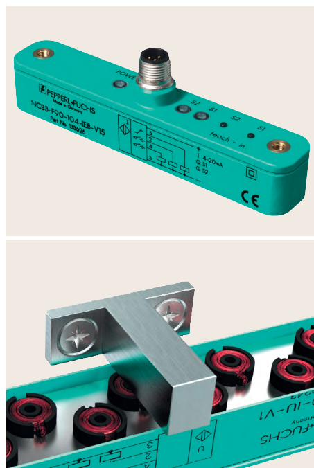
Индуктивный датчик серии PMI определяет крайние и промежуточные положения управляемой заслонки на трубопроводе
