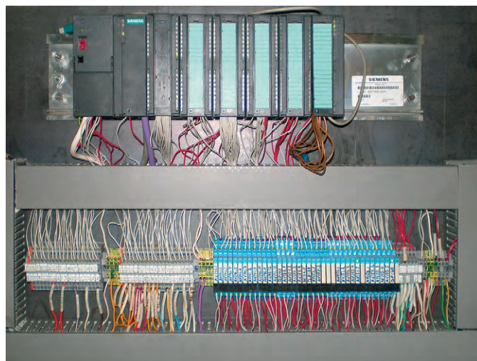
Рис. 4. Периферийная панель управления с модулями ввода-вывода для 4-й линии приготовления маргарина
