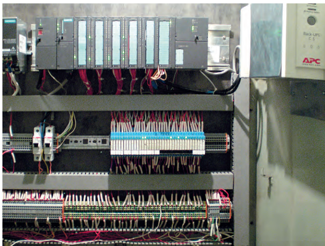
Рис. 3. Центральная панель управления с модулями ввода-вывода для 3-й линии приготовления маргарина
