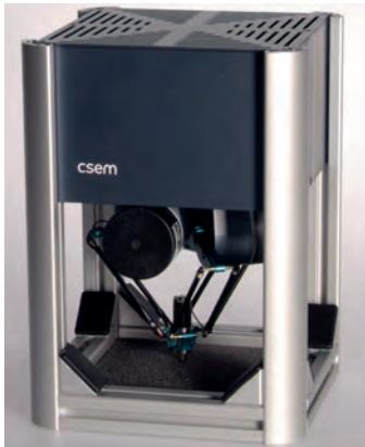
Рис. 5. Робот PocketDelta компании CSEM предназначен для сборки сложных миниатюрных устройств и построен на основе QNX
