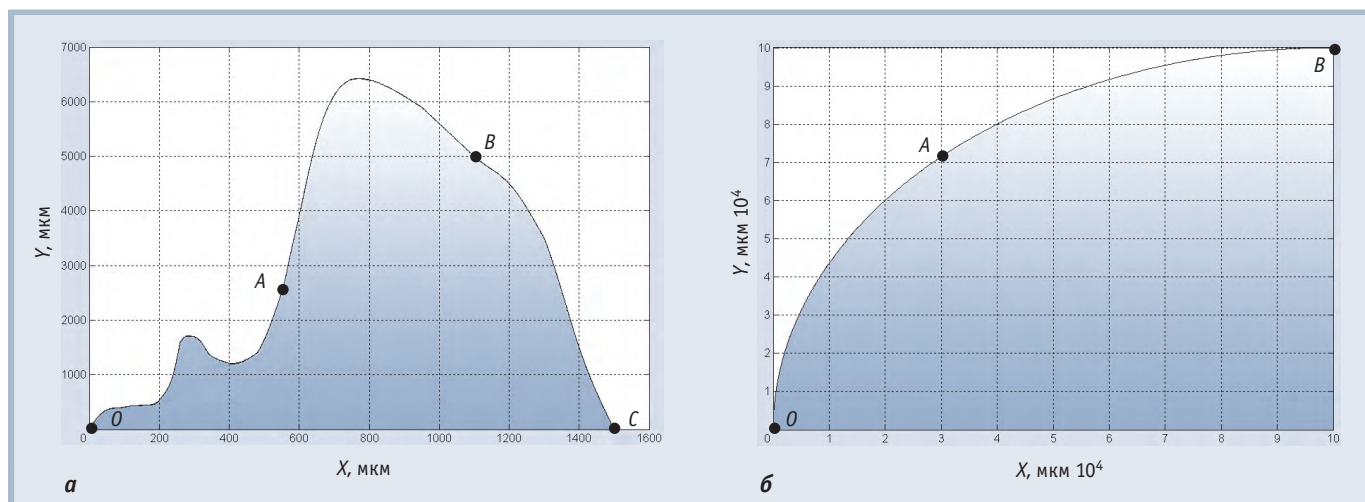
Рис. 8. Примеры графиков заданной и отработанной траекторий на плоскости XY (в обоих примерах – a и b – заданная и отработанная траектории практически совпадают)
