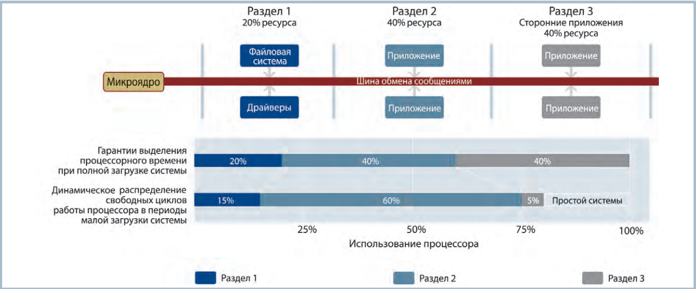
Рис. 4. Распределение процессорных ресурсов при использовании технологии адаптивной декомпозиции
