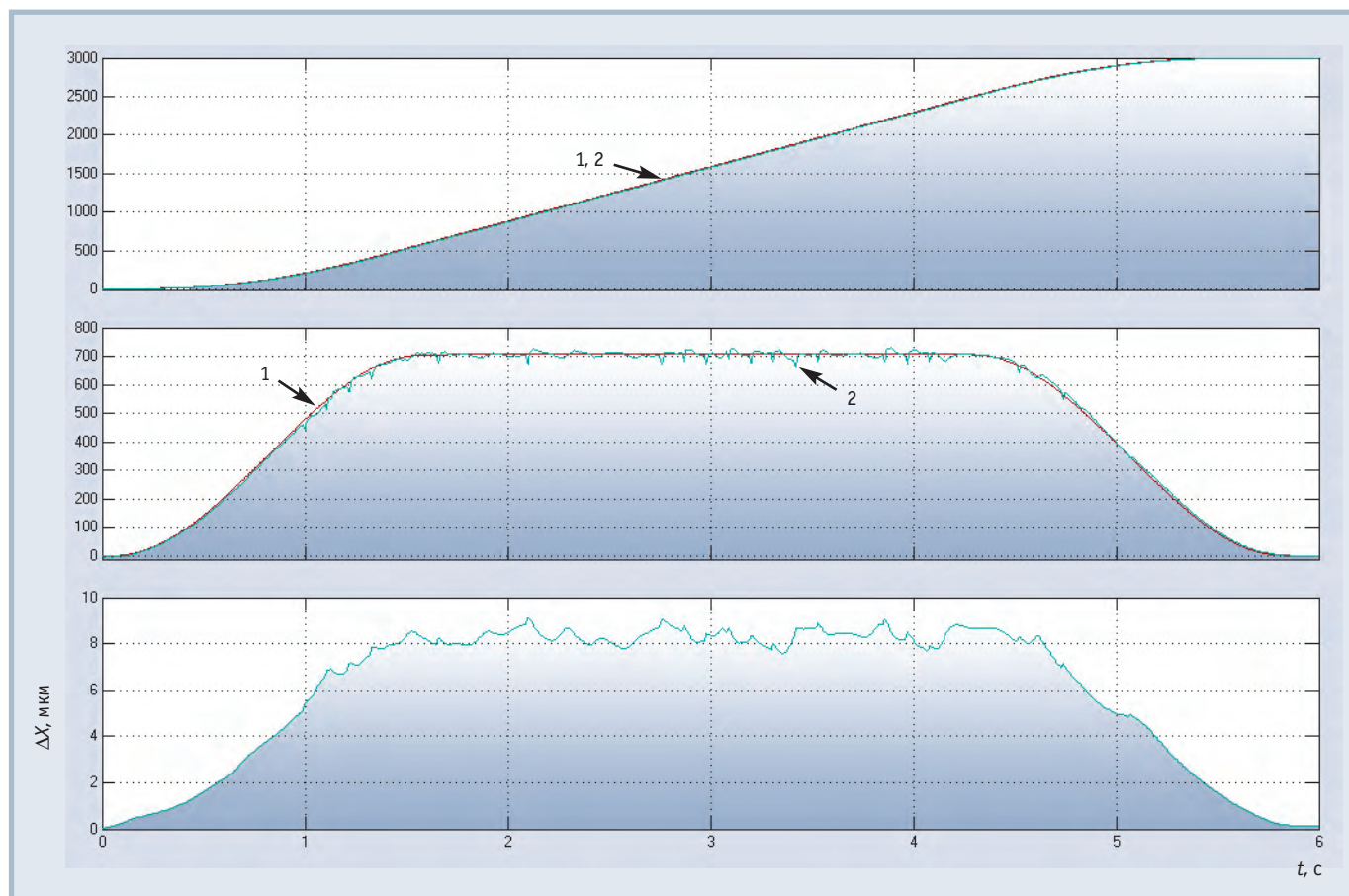
Рис. 11. Пример отработки прямолинейной траектории движения по оси X при наличии цифровой коррекции:
