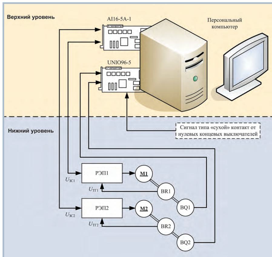
Рис. 2. Двухкоординатный стол
