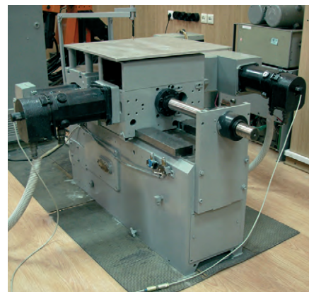
Рис. 2. Двухкоординатный стол
