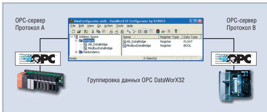
Рис. 3. Реализация функции группировки данных OPC в DataWorX
