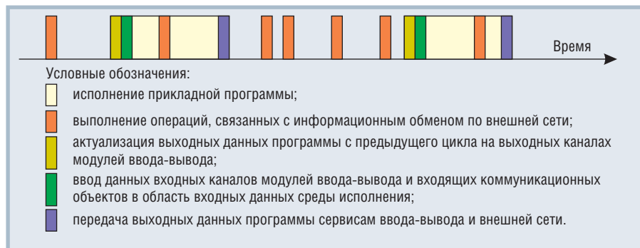
Рис. 2. Циклограмма исполнения прикладной программы
