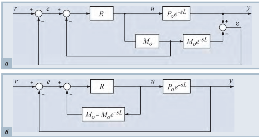
Рис. 26. Модификации системы управления с предиктором Смита
