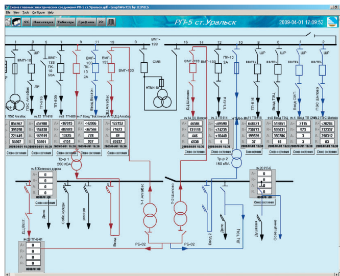
Рис. 5. Мнемосхема диспетчера АСКУЭ
