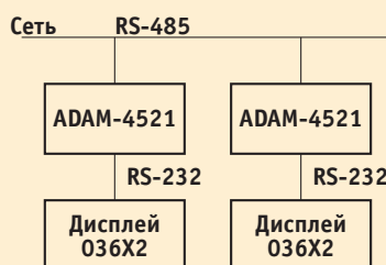
Рис. 13. Включение дисплеев серии 036X2 в сеть RS-485 через модули ADAM-4521
