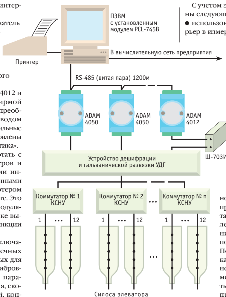
Рис. 1. Структурная схема автоматизированной системы контроля температур
