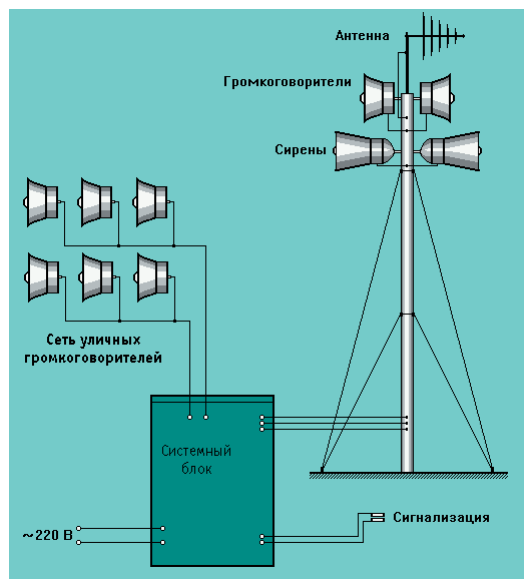
Рис. 4. Внешние подключения системного блока поста оповещения
