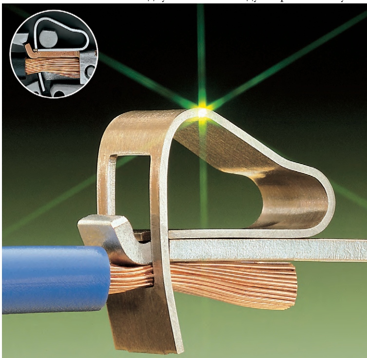
Рис. 6. Основной узел клеммного соединителя Cage Clamp фирмы Wago. До гениальности просто
