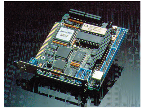
Рис. 2. Платы MicroPC готовы к работе в любом офисном или промышленном компьютере с шиной ISA
