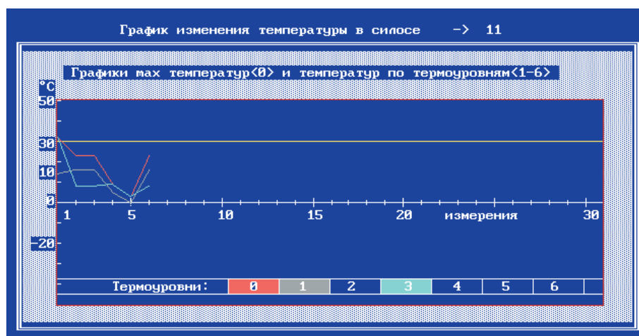
Рис. 4. График изменения температуры в силосе
