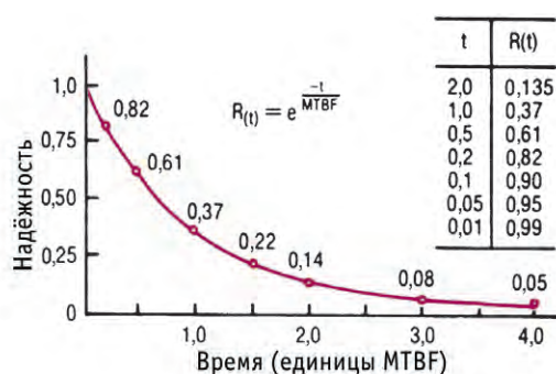
Рис. 8. Зависимость надёжности от времени эксплуатации изделия
