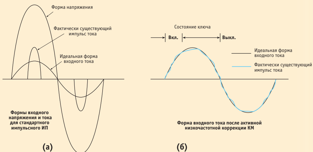
Рис. 4. Нескорректированная форма импульсов входного тока ИП (а). Псевдосинусоидальный входной ток, полученный с помощью активной низкочастотной схемы коррекции КМ (б)
