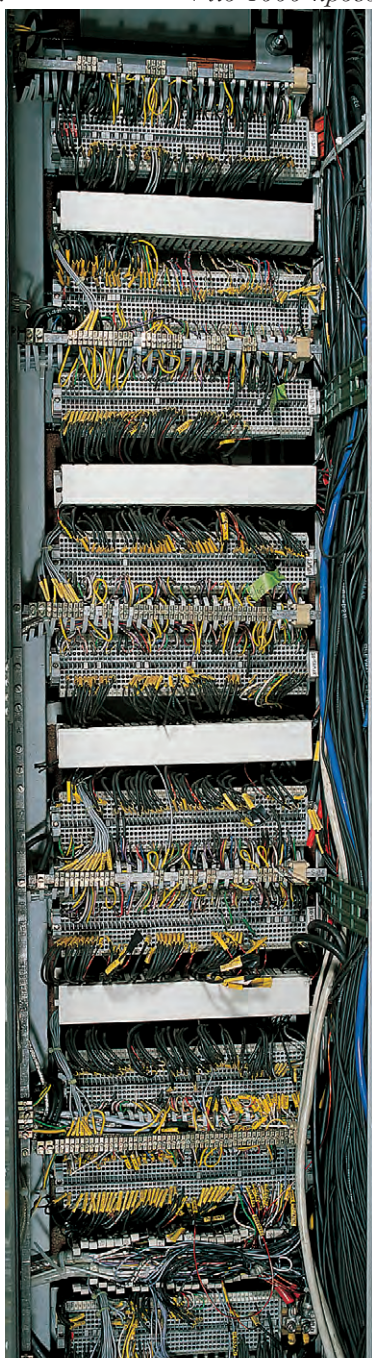
Типичный шкаф управления на железной дороге с клеммами Wago фронтального электро монтажа
