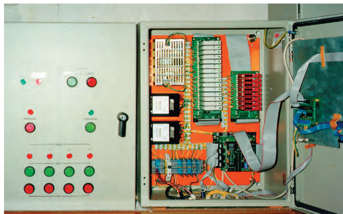
Размещение составных частей блока управления системы ЛСУ КНС на шасси шкафа
