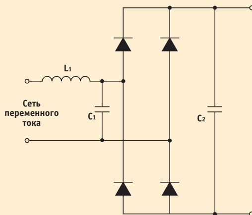
Рис. 1. В типичной пассивной схеме коррекции коэффициента мощности для получения формы входного тока с низкими искажениями применяются конденсатор С1, дроссель L1
