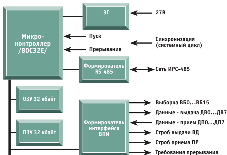
Рис. 3. Структурная схема встраиваемого периферийного контроллера
