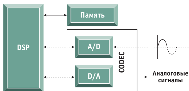
Рис. 1. Общая структура DSP-системы
