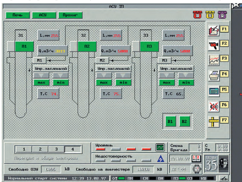
Рис. 6. Мнемосхема газоочистки
