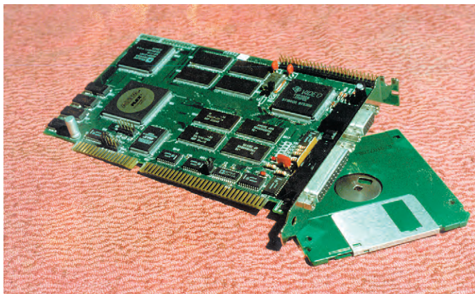
Рис. 3. Внешний вид контроллера «МИКСТ»
