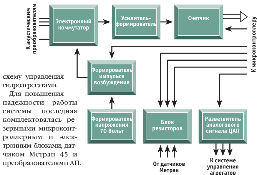
Рис. 3. Функциональная схема электронного блока
