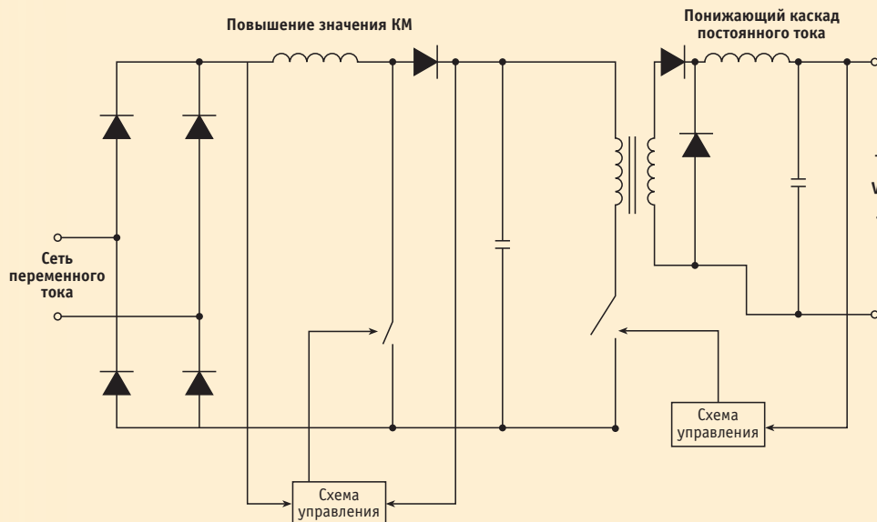
Рис. 2. В этом двухкаскадном источнике для осуществления активной коррекции коэффициента мощности применяется повышающий импульсный регулятор
