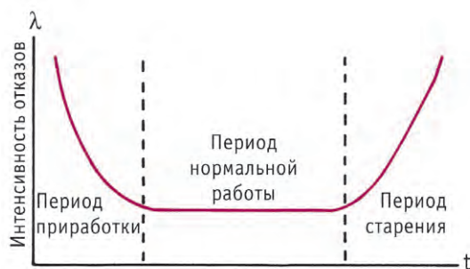
Рис. 7. Типичная зависимость интенсивности отказов от времени
