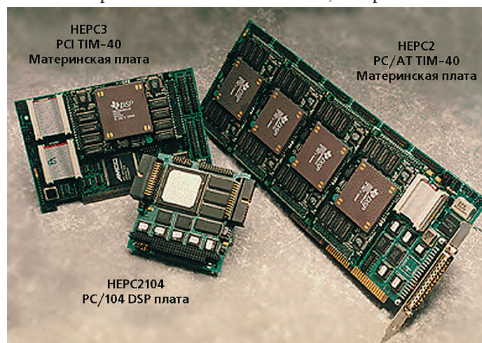
Платы HEPC2 и HEPC3 (Hunt Engineering)
