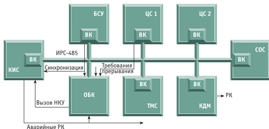
Рис. 1. Пример использования ОБК и ВК в составе бортового вычислительного комплекса КА КИС — командно-измерительная система; ТМС — телеметрическая система; КДМ — дополнительная командно-диагностическая матрица; СОС — система орбитальной стабилизации; ЦС1, ЦС2 — целевые системы; БСУ — бортовое синхронизирующее устройство; НКУ — наземный комплекс управления; РК — разовые команды.
