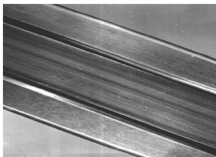
Рис. 1а. Вид поврежденной беговой дорожки наружной обоймы роликоподшипника. Наиболее ранняя стадия: появление рисок
