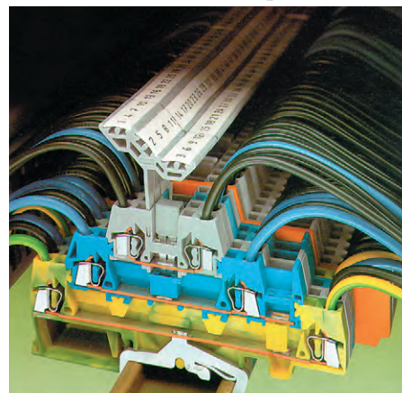
Рис. 3. Многоярусные клеммы значительно экономят монтажное пространство
