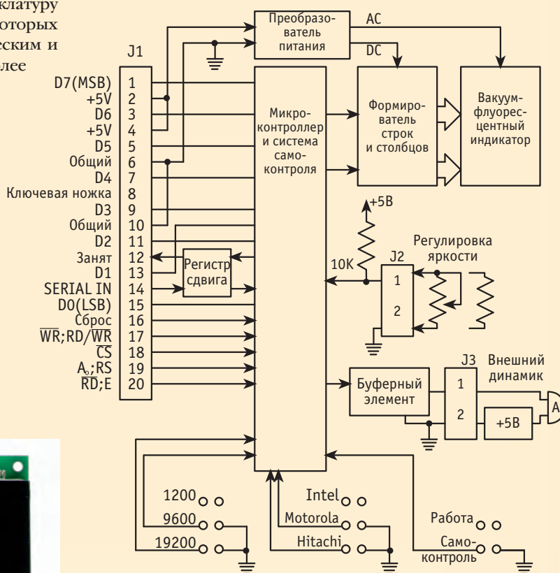
Рис 3. Вакуум-флуоресцентный дисплей Century. Схема электрическая функциональная
