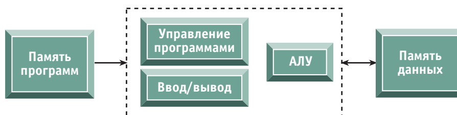
Рис. 2б. Гарвардская архитектура
