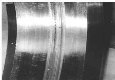
Рис. 1б. Вид поврежденной беговой дорожки наружной обоймы роликоподшипника. Минимальная стадия: появление отдельных участков с микроповреждениями
