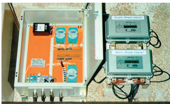
Внешний вид блока ввода аналоговых сигналов
