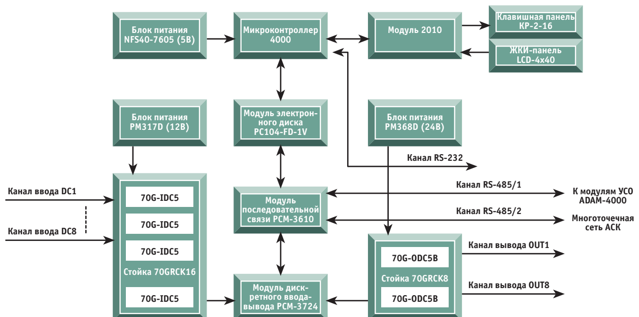
Рис. 3. Структурная схема ЛСУ КНС
