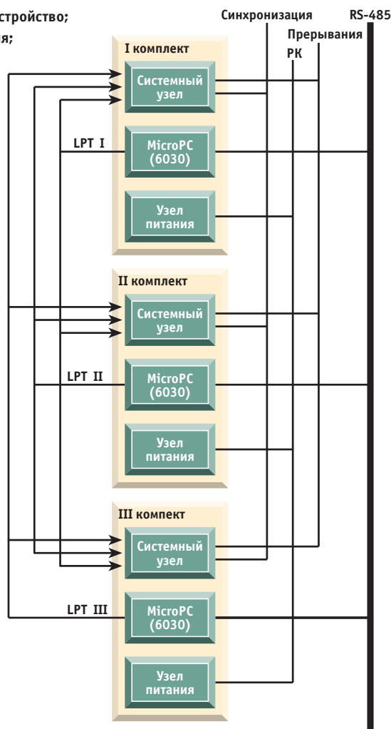
Рис. 2. Структурная схема отказоустойчивого бортового компьютера (ОБК)
