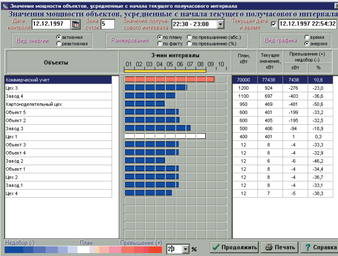
Рис. 11. Значения мощности объектов, усредненные с начала текущего полукасового интервала (объекты проранжированы по плановым значениям полукасовой мощности)
