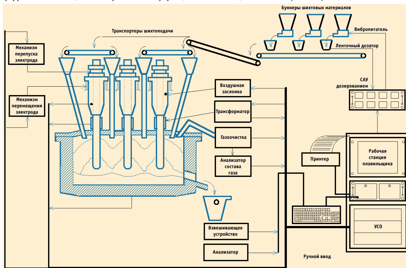
Рис. 1. Структурная схема АСУ ТП выплавки сплавов на основе кремния
