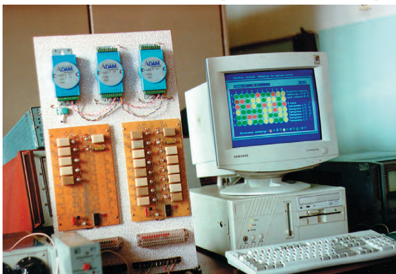
Рис. 2. Стенд для отработки технических решений системы контроля температур
