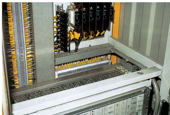
Первый опыт применения клемм WAGO в пассажирских вагонах. Проходные клеммы до 2,5 мм 2 , стандартный электро-монтаж
