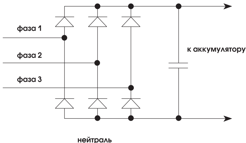
Рис. 9. Выпрямитель трехфазного источника бесперебойного питания
