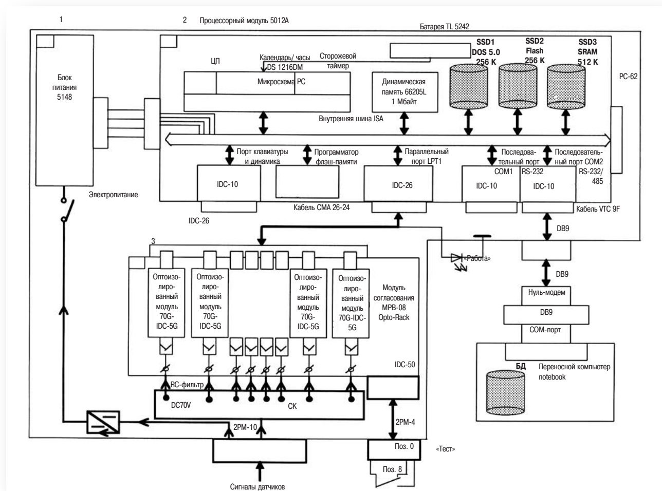
Рис. 1. Функциональная схема бортового регистратора
