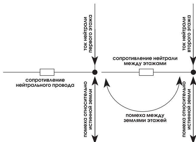
Рис. 7. «Заземление» компьютерной сети с помощью нейтрального провода
