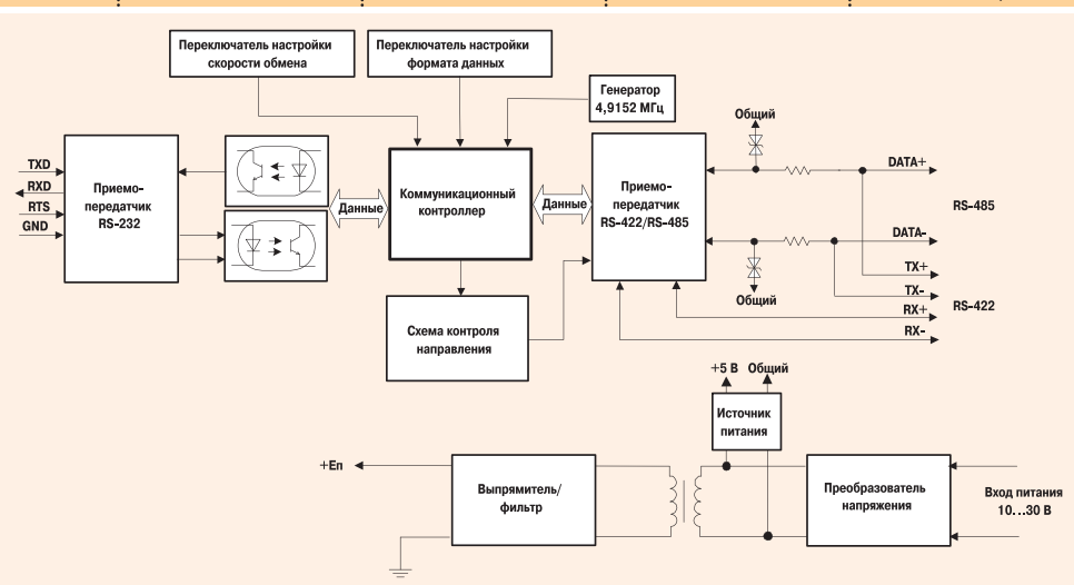
Рис. 8. Структурная схема модуля ADAM-4520
