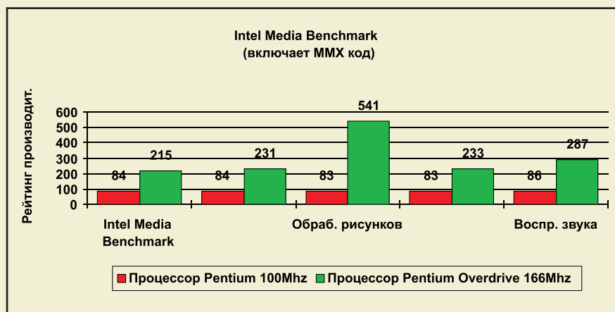
Рис. 1. Результаты теста Intel Media Benchmark для систем с процессором Pentium/100 МГц и после его замены на Pentium OverDrive с технологией MMX и тактовой частотой 166 МГц
