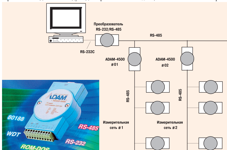
Рис. 13. Вариант применения модуля ADAM-4500
