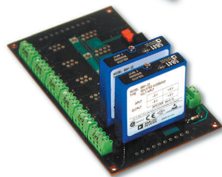
Рис. 5. Модули УСО фирм Grayhill и Analog Devices, используемые в контроллерах
