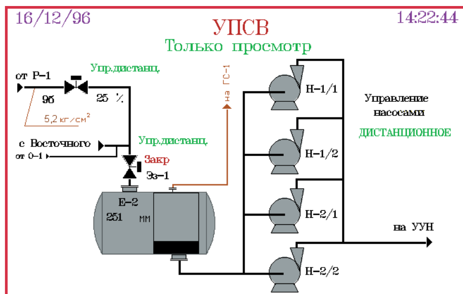
Рис. 4. Пример мнемосхемы
