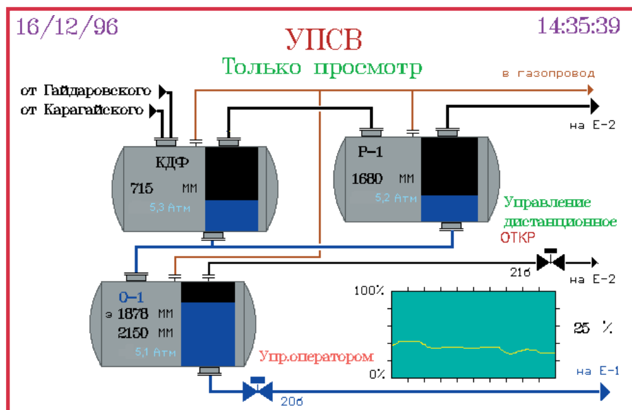
Рис. 3. Пример мнемосхемы
