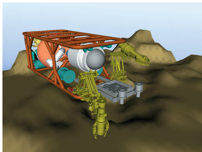
Рис. 2. Трехмерная геометрическая модель подводного аппарата
