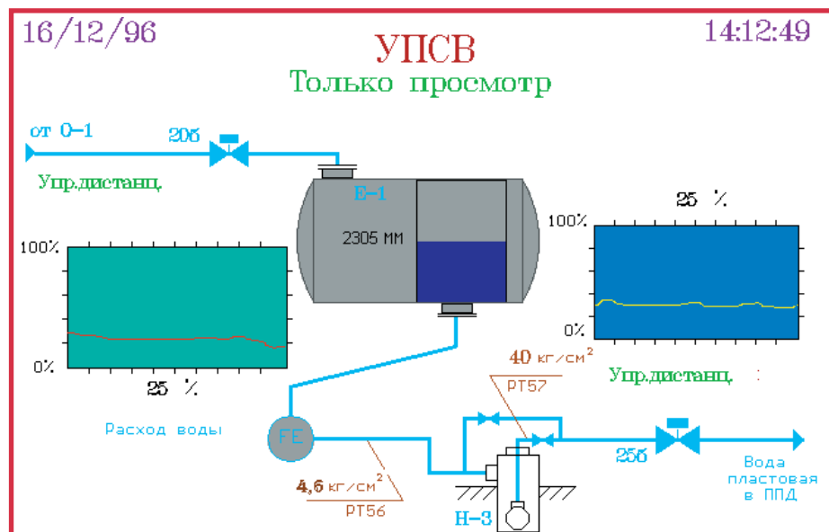
Рис. 5. Пример мнемосхемы
