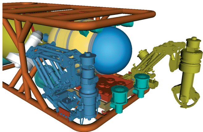
Рис. 2. Геометрическая модель подводного аппарата «АКБА-ЧС»
