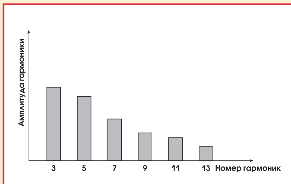
Рис. 5. Спектр тока импульсного блока питания
