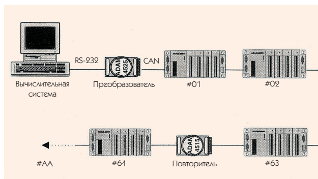
Рис. 17. Структура распределенной системы сбора данных и управления на базе контроллеров ADAM-5000/CAN
