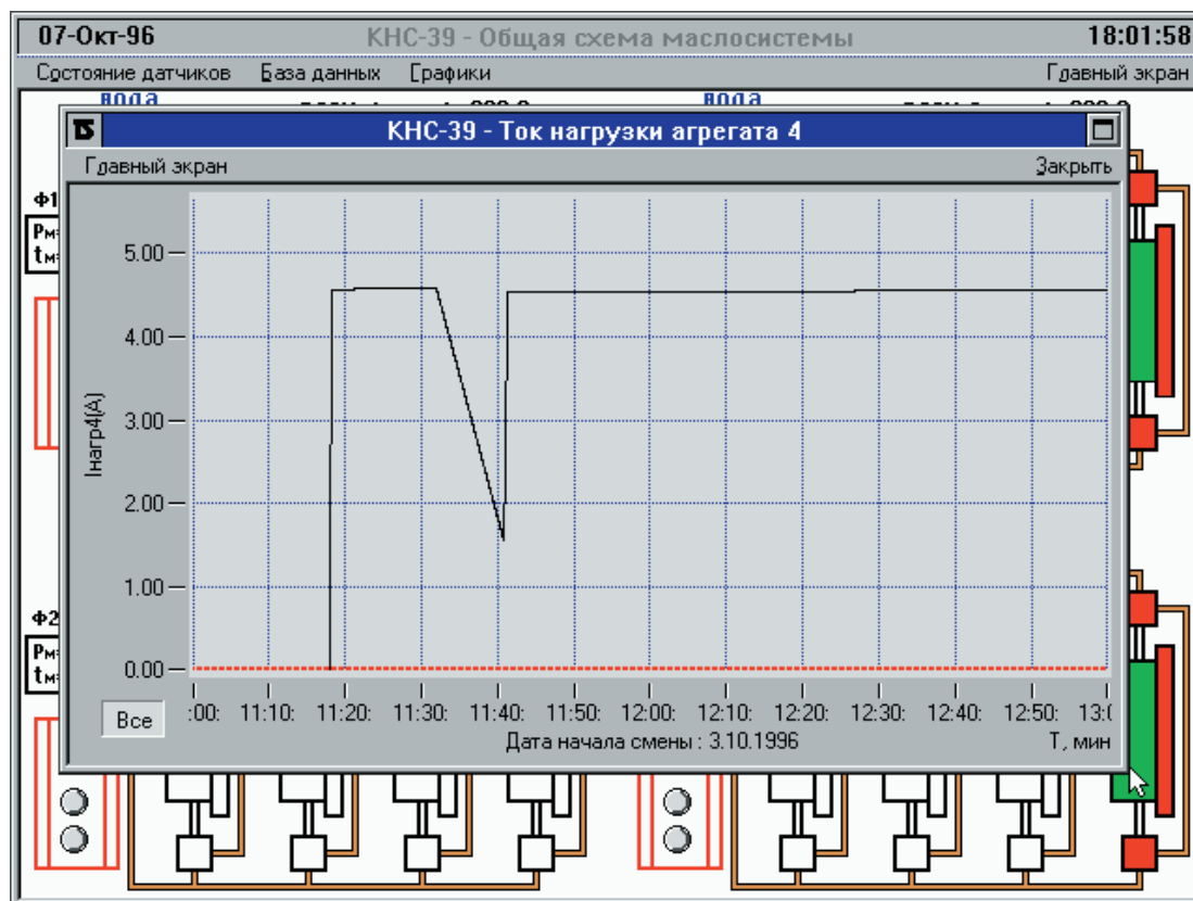
Рис. 8. График аналогового сигнала объекта
