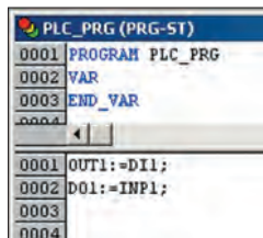
Рис. 7. Текст программы для ПЛК FASTWEL I/O
