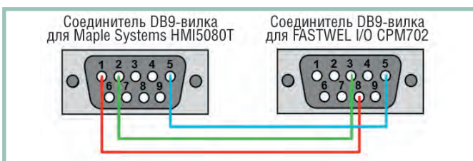
Рис. 2. Схема подключения контактов со стороны соединительного кабеля для CPM702
