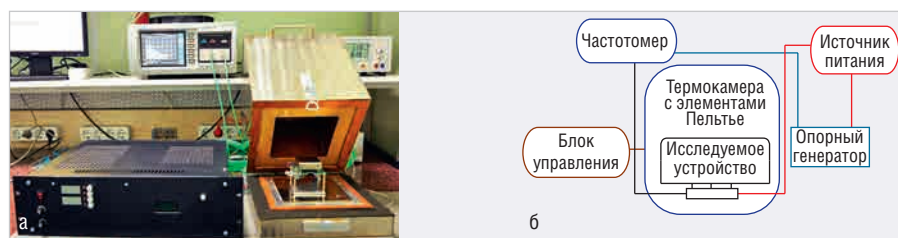
Рис. 7. Стенд для испытаний с температурной камерой на элементах Пельтье: а) общий вид; б) структурная схема
