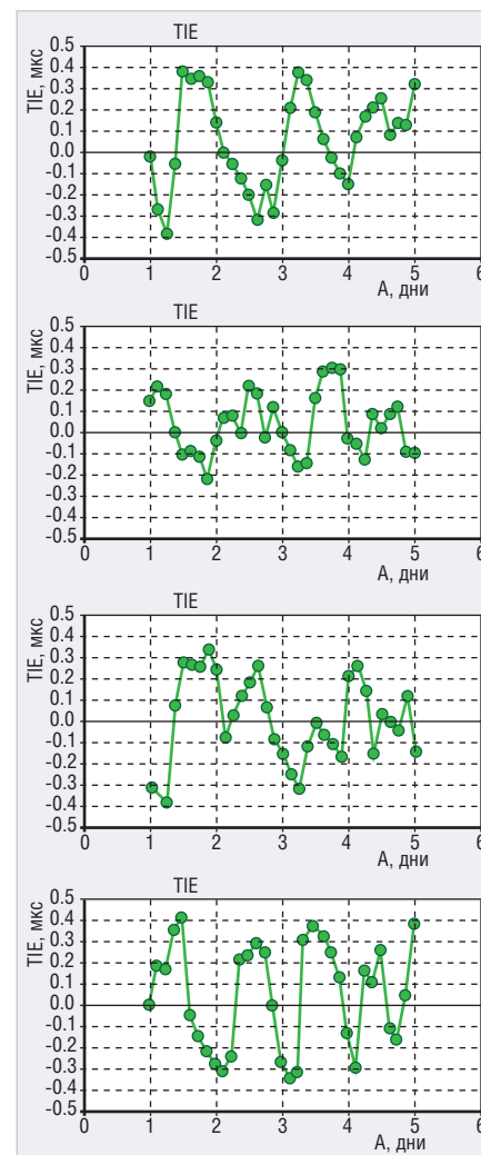
Рис. 8. Результаты измерения временной ошибки за 24 ч для прецизионных кварцевых генераторов GK360 при изменении температуры окружающей среды в пределах 5°C в течение суток
