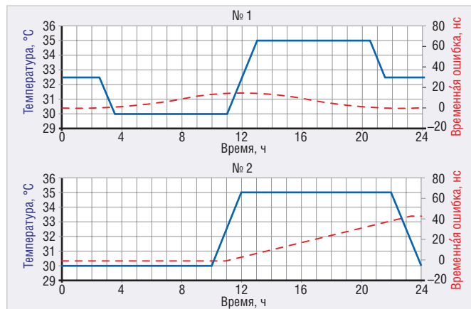
Рис. 2. Сравнение профилей изменения температуры
