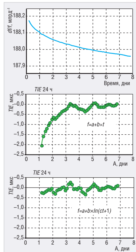
Рис. 4. Оценка временной ошибки с линейной (в центре) и логарифмической (внизу) функциями аппроксимации для одного и того же кварцевого генератора
