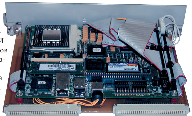
Рис. 7. Блок компьютера PC-680 Octagon Systems
