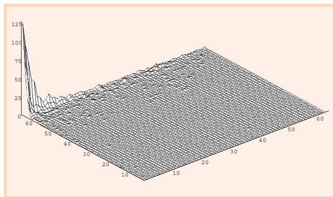
Рис. 14. Двухмерное распределение энергия-соотношение компонентов сцинтилляционной вспышки в спокойной обстановке
