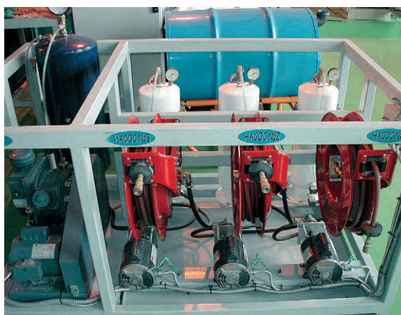
Рис. 9. Маслораздаточная станция
