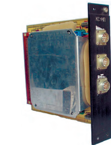
Рис. 5. Технологический образец модуля КС-МП в сборе, с установленной верхней фиксирующей крышкой
