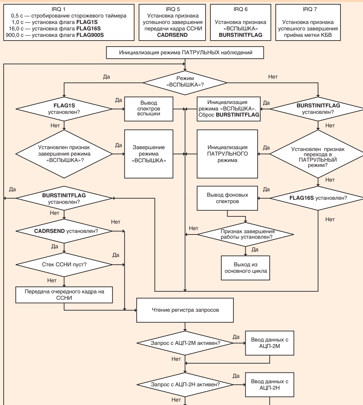
Рис. 8. Блок-схема основного цикла работы системы
