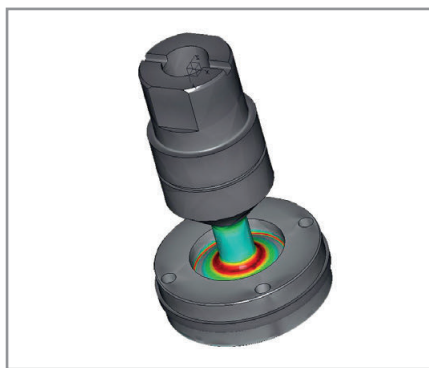
Рис. 15. Датчик контроля прикладываемого пилотом усилия – монтаж в джойстик
