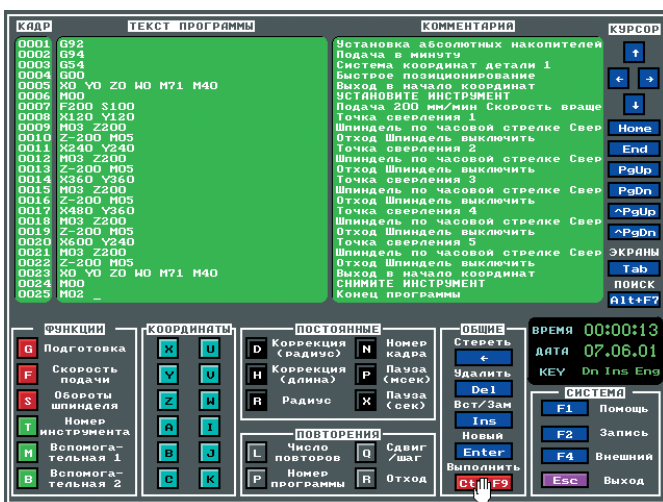
Рис. 5. Экран пользователя для подрежима Изменить режим Подготовка программ
