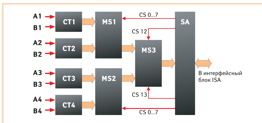
Рис. 2. Устройство для измерения температуры, реализованное на базе изделий фирмы Fastwel и модулей UCO Grayhill
