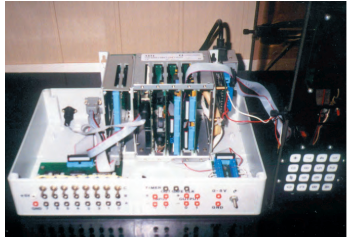
Рис. 5. Внешний вид микропроцессорного тренажёра
