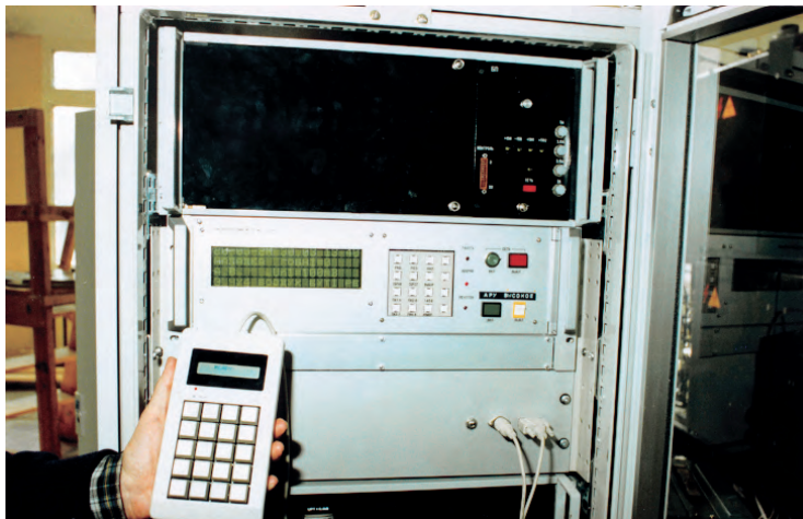
Рис. 5. Блок управления с пультом технолога-обогапителя
