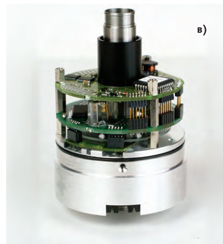
в) Верхняя плата включает в себя EEPROM для хранения программы, выходные схемы, цепи питания
