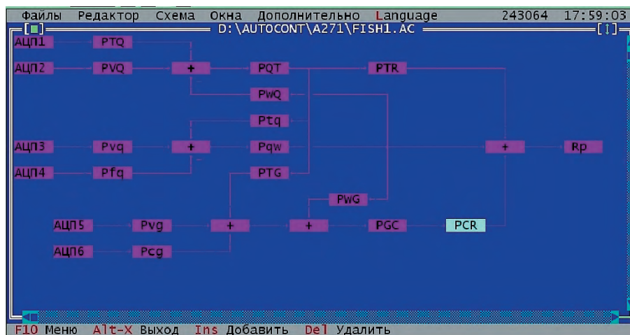
Рис. 3. Внешний вид окна программы с фрагментом модели тестируемого технологического процесса (AutoCont)
