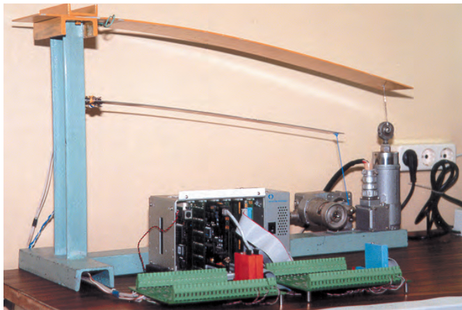
Стенд моделирования и исследования контуров регулирования АСУ ТП
