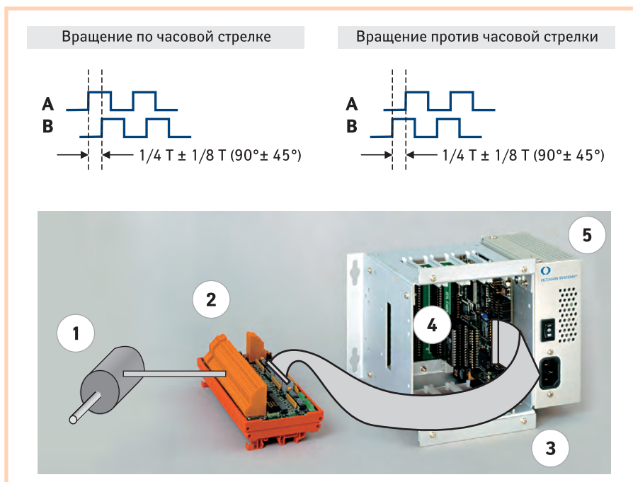
Рис. 3. Заказная схема подсчёта импульсов от четырёх шифраторов типа Omron E6A
