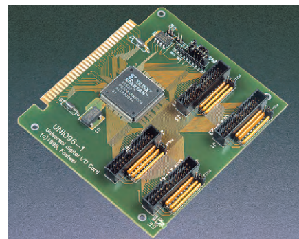
Внешний вид многофункциональной платы дискретного ввода-вывода UNIO96/48 фирмы Fastwel
