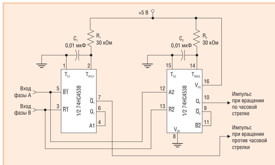
Рис. 5. Схема, построенная на основе сдвоенного одновибратора, представляет собой простой декодер квадратурных сигналов. Постоянные времени цепочек R_1C_1 и R_2C_2 задают длительность выходных сигналов, которые должны быть короче самого короткого квадратурного сигнала
