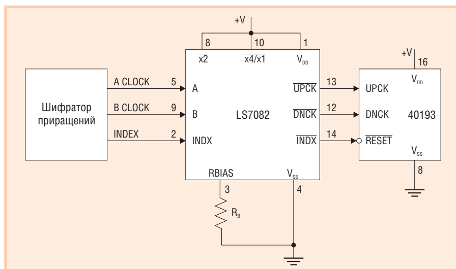
Рис. 6. Типовая схема подключения в режиме x4
