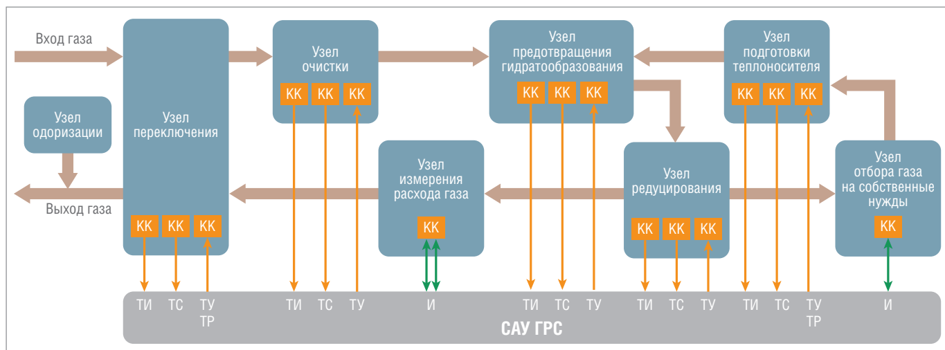
Рис. 1. Структура системы автоматизации централизованного типа
