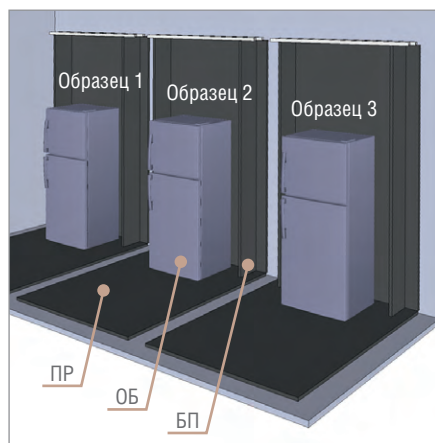
Условные обозначения: ПР – платформа; ОБ – образец; БП – перегородка.
