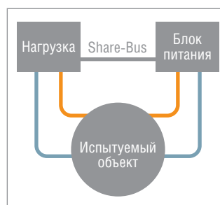
Рис. 16. Подключение источника, испытуемого объекта и нагрузки по двухквадрантной схеме
