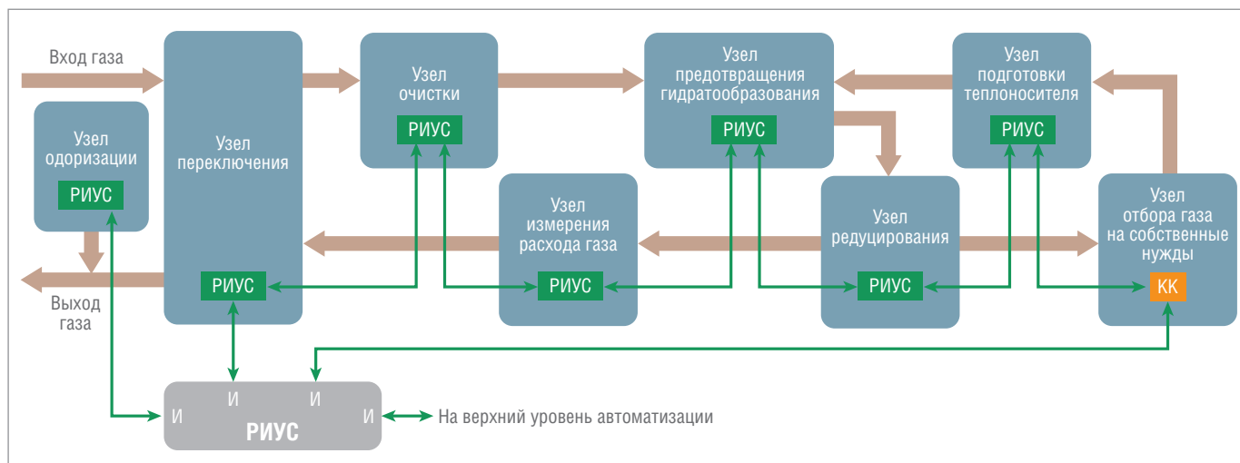
Рис. 2. Структура системы автоматизации распределённого типа
