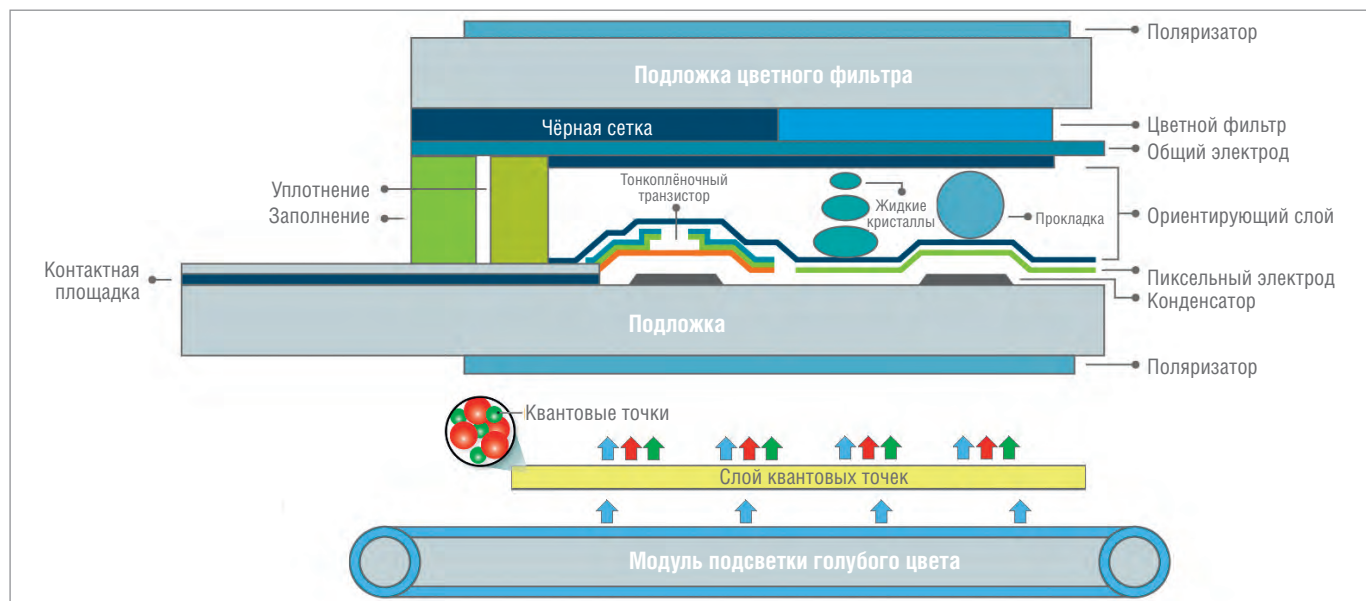
Рис. 9. Структура QD-дисплея
