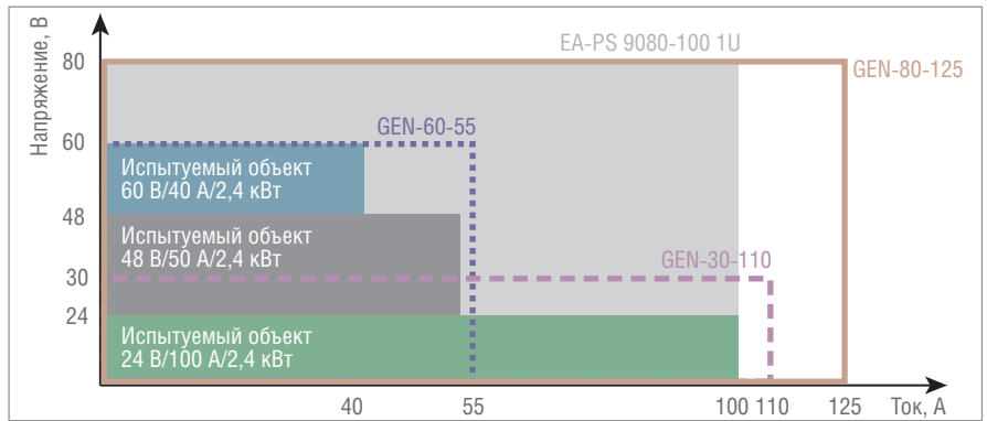
Рис. 6. Иллюстрация преимущества источников с технологией авторанжирования
