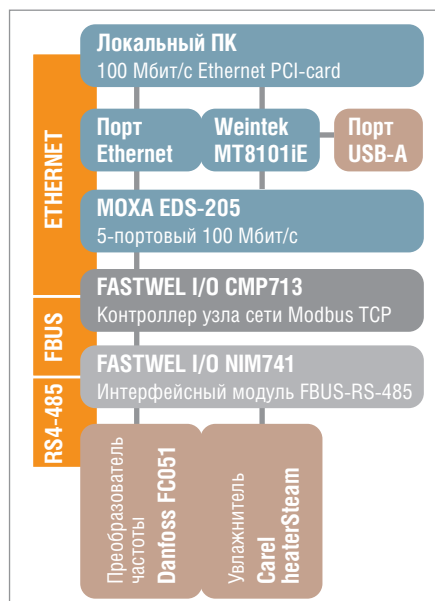
Рис. 6. Организация сети
