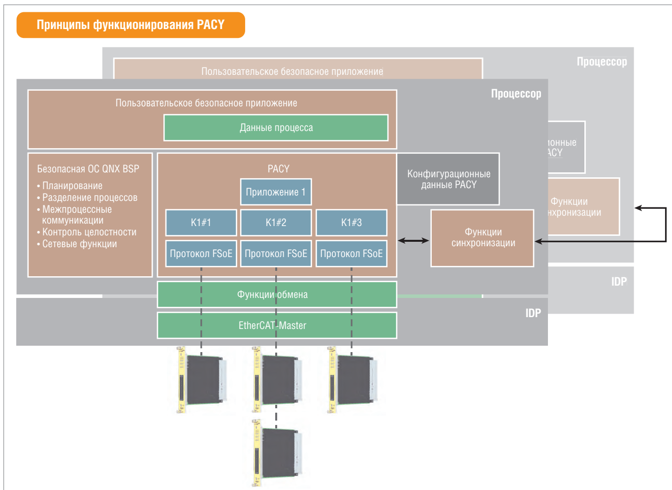
Рис. 3. Структура безопасного ввода/вывода РАСУ
