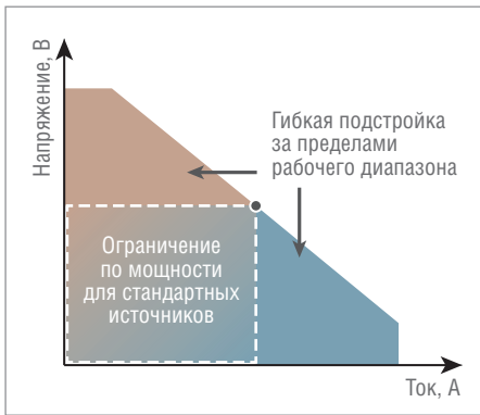
Рис. 5. Авторанжирование рабочих диапазонов
