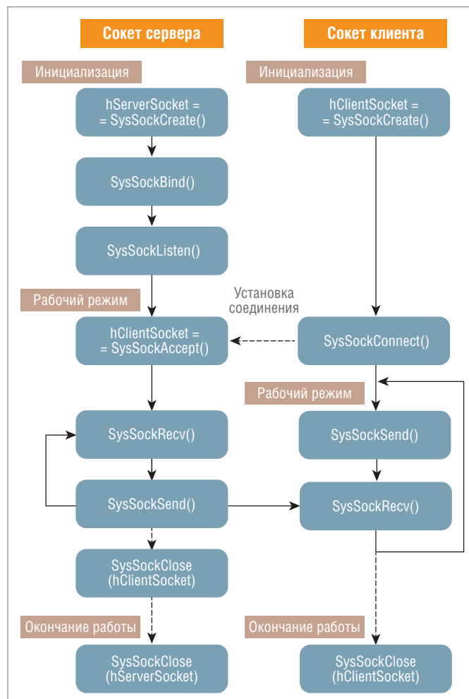
Рис. 6. Работа простых клиентского (справа) и серверного (слева) TCP-сокетов
