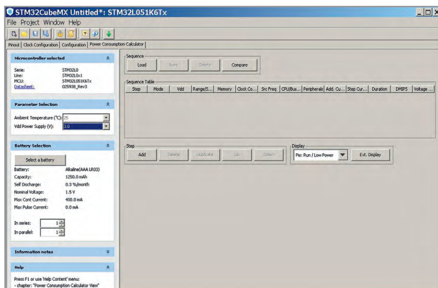
Рис. 7. Закладка «Power Consumption Calculator»
