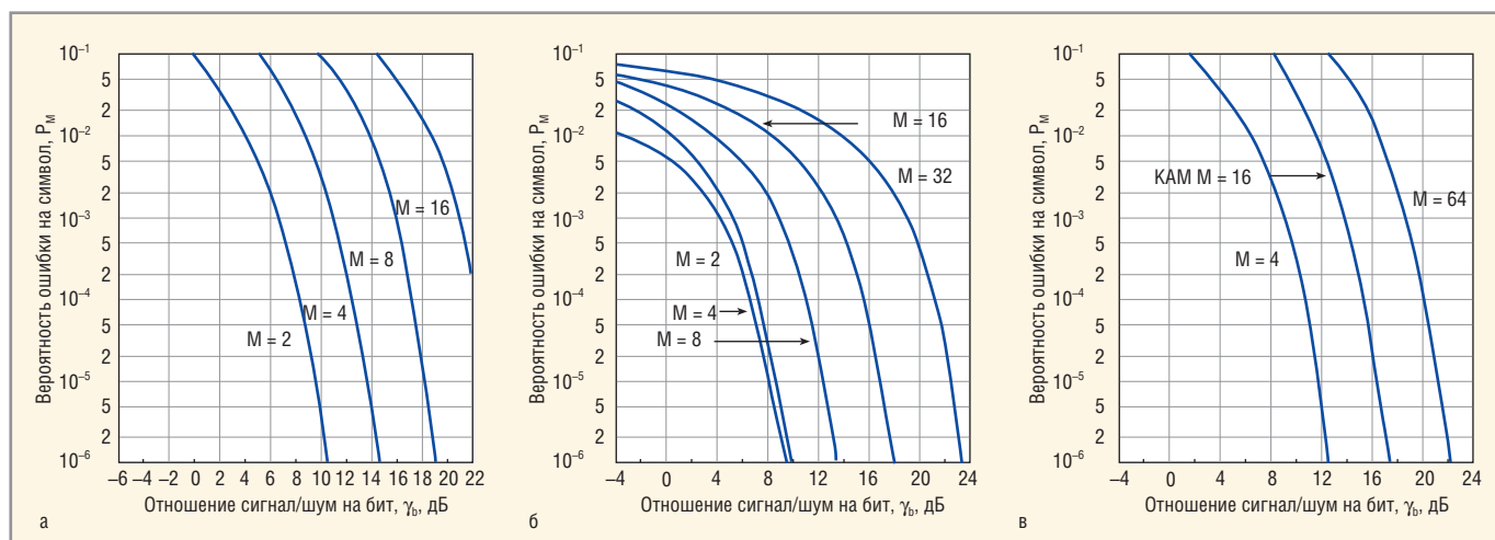
Рис. 2. Вероятность ошибки на символ при [2]: а – М-АМ; б – М-ФМ; в – М-КАМ
