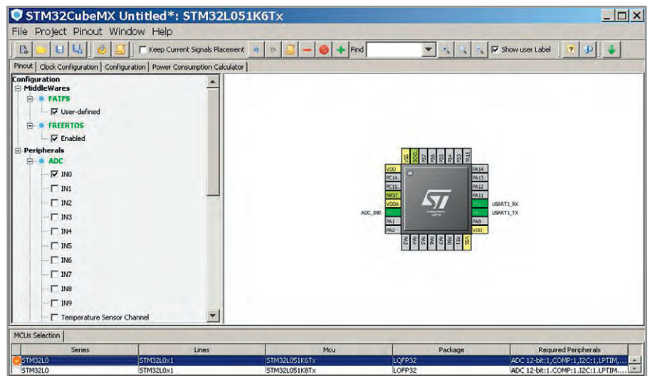
Рис. 3. Периферийные устройства микроконтроллера и аппаратные блоки в развёрнутом виде
