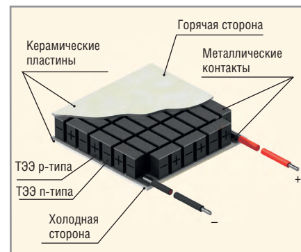
Рис. 3. Термоэлектрический генераторный модуль в разрезе
