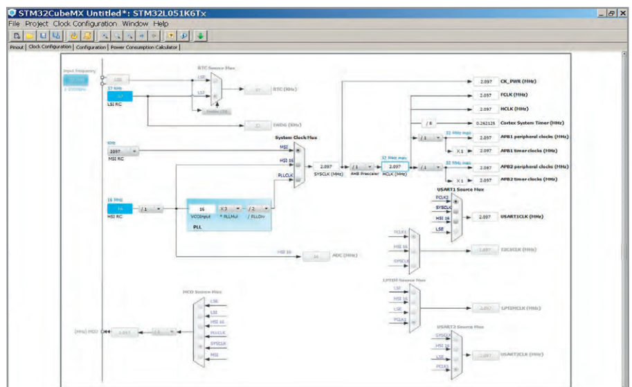
Рис. 4. Закладка «Clock Configuration»
