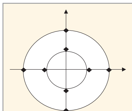
Рис. 3. Двухуровневая квадратурная амплитудно-инверсная модуляция (2-QAM)
