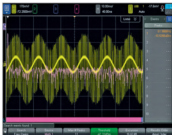
Рис. 7. БПФ сигнала USB с наведённым низкочастотным шумом
