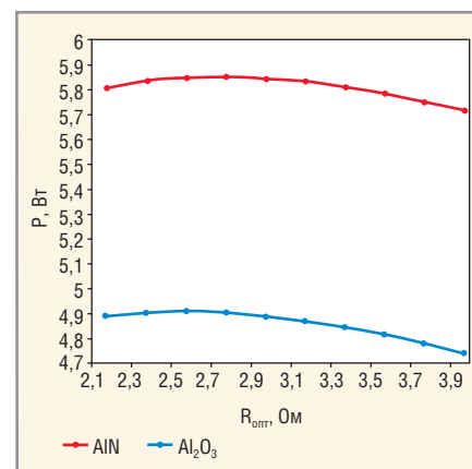
Рис. 7. Сравнительные испытания ТГМ-199-1,4-0,8
