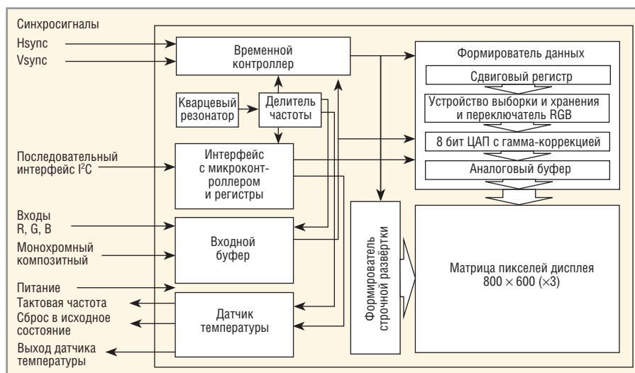
Рис. 3. Функциональная схема микродисплея
