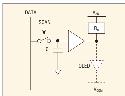
Рис. 9. Функциональная схема субпиксельной ячейки
