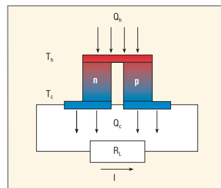
Рис. 2. Термопара с тепловым потоком Q и внешней электрической нагрузкой R_L
