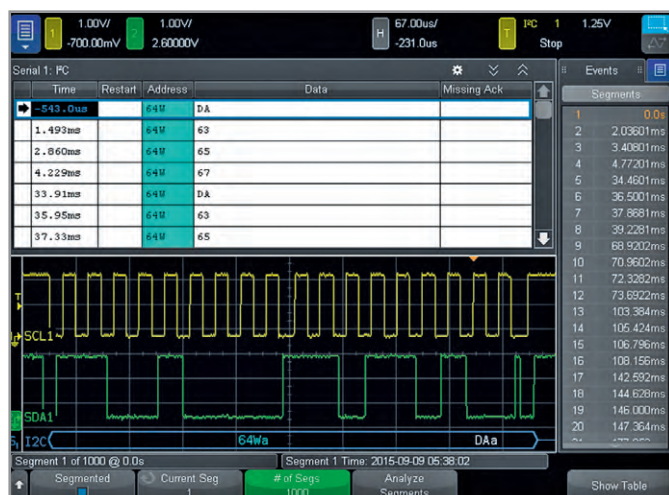
Рис. 3. Декодирование данных последовательной шины в режиме сегментированной памяти
