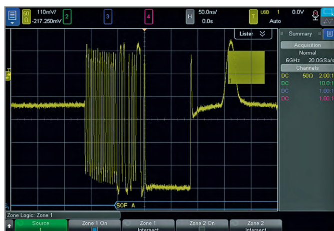
Рис. 5. Локализация наведённой помехи с помощью запуска по выделенной области
