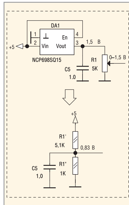
Рис. 8. Замена стабилизатора и переменного резистора делителем напряжения
