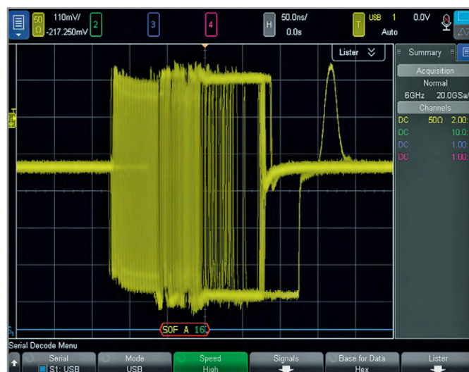
Рис. 4. Сигнал USB с наведённой помехой
