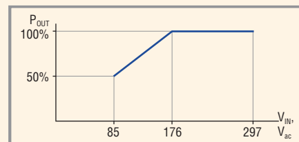
Рис. 2. Ограничение мощности от величины входного напряжения
