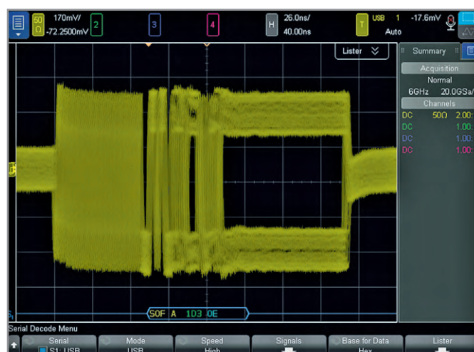
Рис. 6. Сигнал USB с низкочастотным шумом
