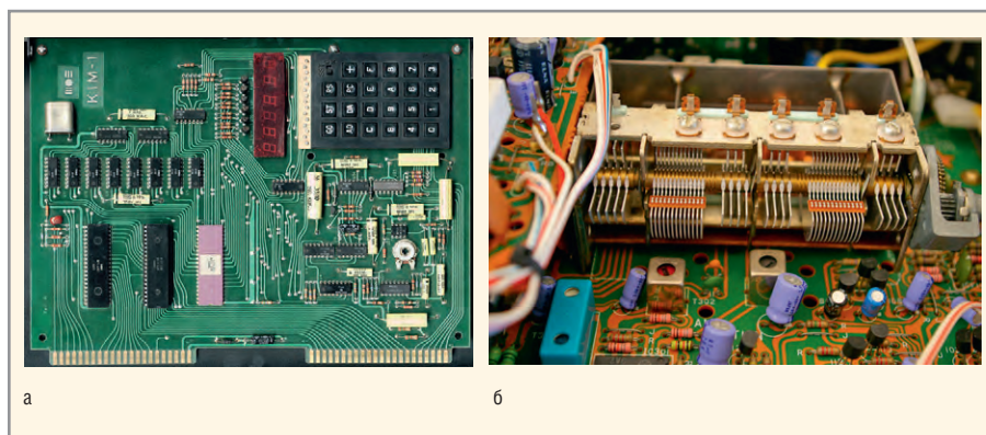
Рис. 1. Внешний вид печатных плат одноплатного компьютера KIM-1 (а) и радиоприёмника Yamaha CR-1040 (б)
