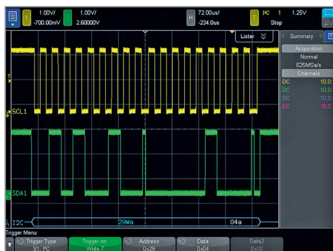
Рис. 2. Запуск по сигналам шины I 2 C и автоматическое декодирование данных
