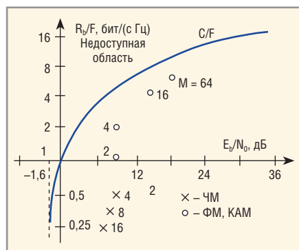
Рис. 1. Сравнение М-ЧМ, М-ФМ и М-КАМ
