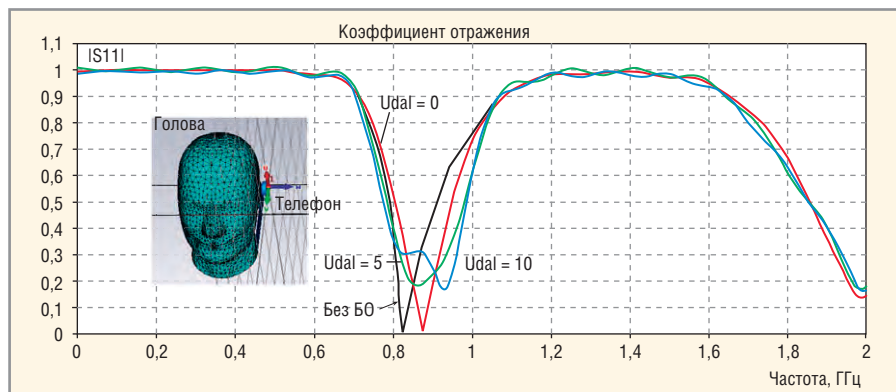
Рис. 4. Рассогласование антенны сотового телефона при изменении удаления от БО
