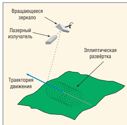
Рис. 4. Сканирующая система с вращающимся зеркалом
