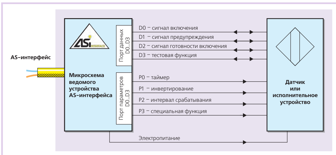
Рис. 11. Схема датчика или исполнительного устройства с интегрированным AS-интерфейсом
