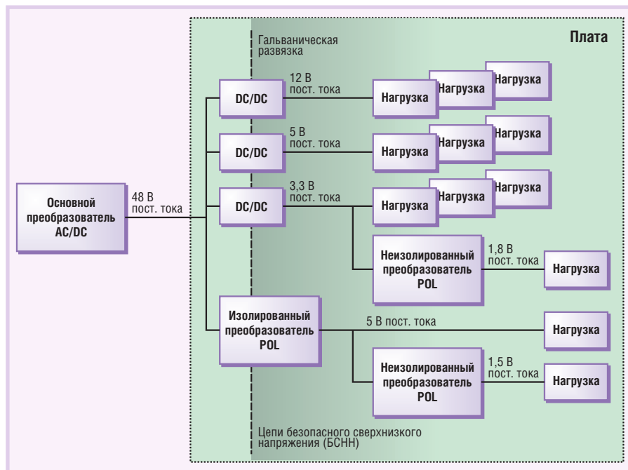
Рис. 1. Распределённая система электропитания с однократным преобразованием
