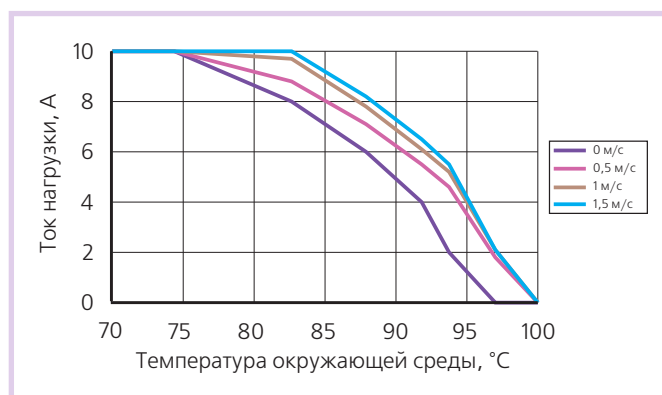
Рис. 20. Зависимость тока нагрузки от температуры окружающей среды и скорости воздушного потока принудительного обдува для SIL10-05W3V3 при входном напряжении 5 В без регулирования выходного напряжения
