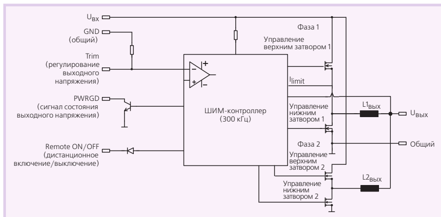
Рис. 25. Упрощённая функциональная схема преобразователя серии SIL30
