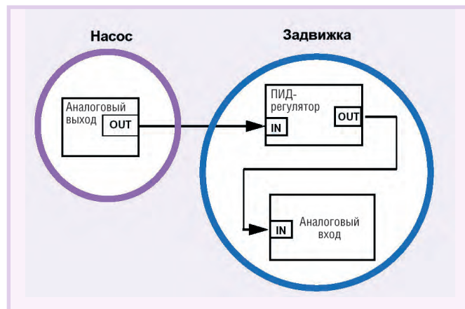
Рис. 4. Настройка алгоритма управления в Foundation Fieldbus
