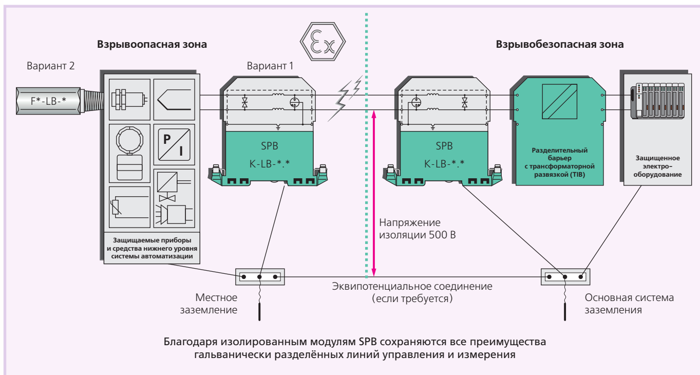
Рис. 8. Применение модулей SPB с электрическими аппаратами, приборами и другими средствами автоматизации, установленными во взрывоопасных зонах
