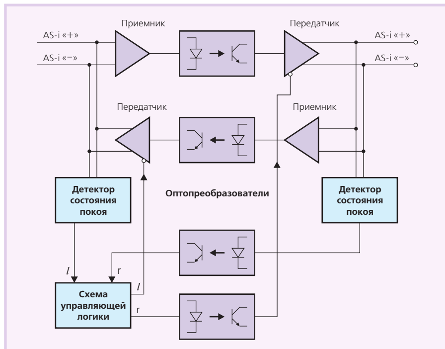
Рис. 15. Структурная схема повторителя
