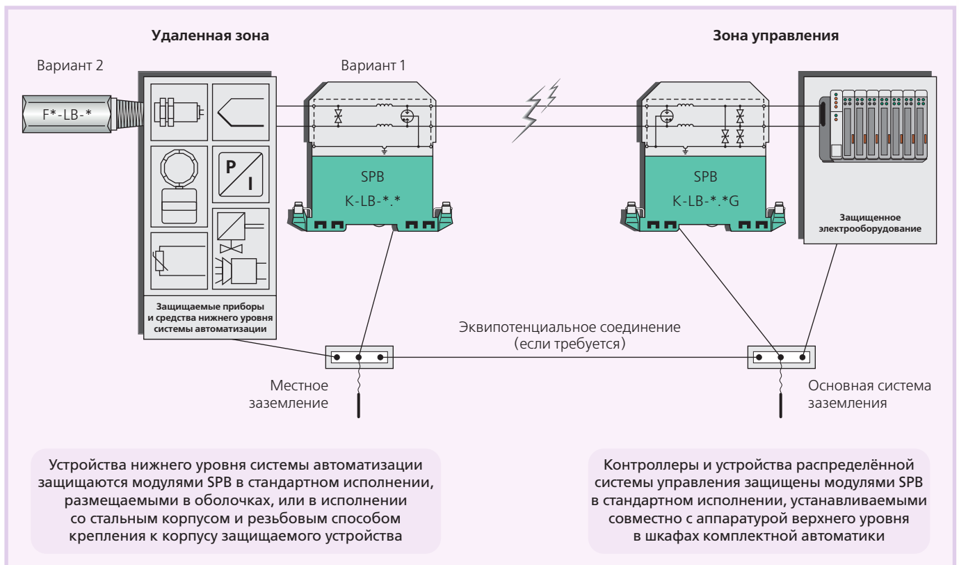
Рис. 7. Применения модулей SPB для защиты выносных устройств систем автоматизации
