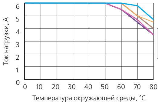
Рис. 10. Зависимости тока нагрузки от температуры окружающей среды и скорости воздушного потока принудительного обдува для SIL06-12SADJ при значении выходного напряжения 5 В
