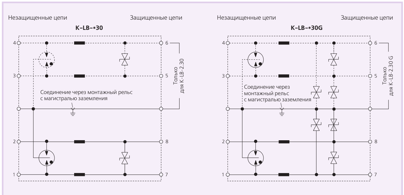
Рис. 6. Электрические схемы устройств ограничения напряжения серий K-LB-*30 и K-LB-*30G
