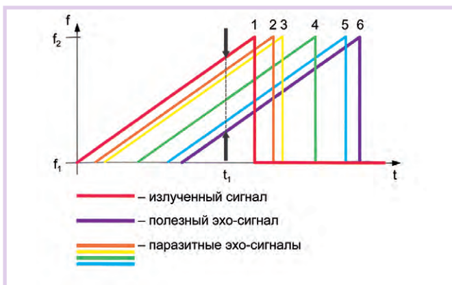
Рис. 2. Паразитные отражения при использовании технологии FMCW
