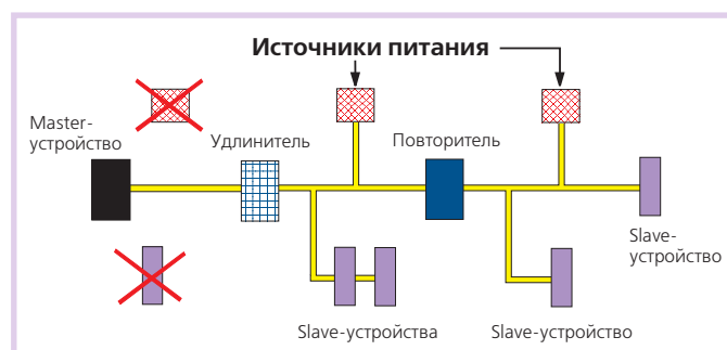
Рис. 6. Топология сети AS-интерфейса с повторителем и удлинителем
