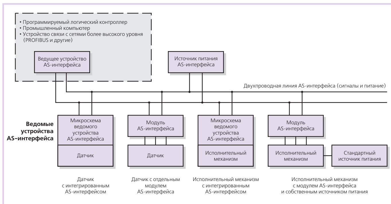
Рис. 1. Схема подключения устройств к AS-интерфейсу
