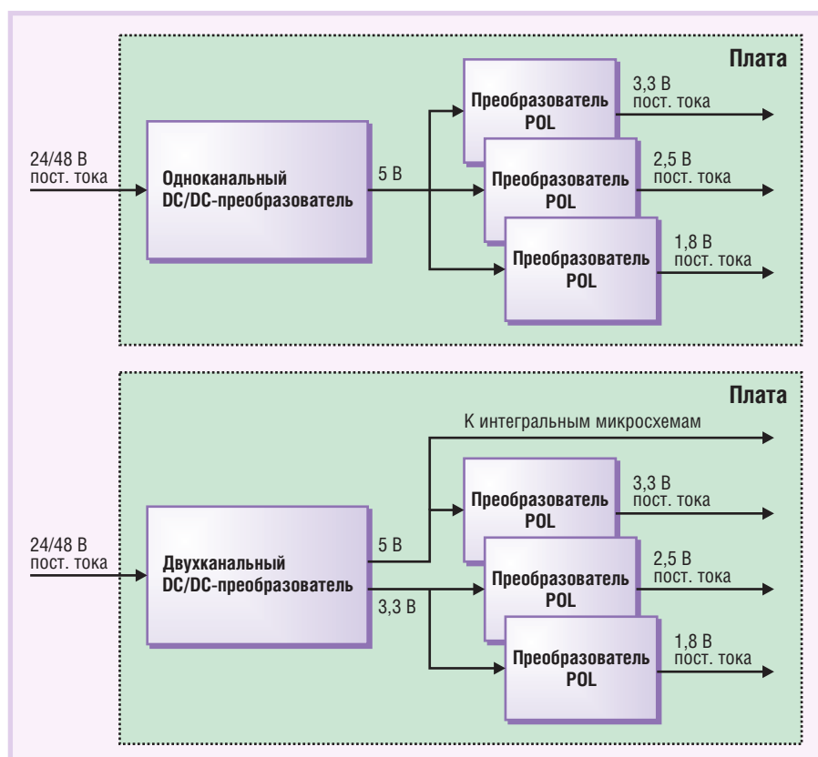
Рис. 5. Система электропитания с формированием напряжений промежуточной шины DC/DC-преобразователем
