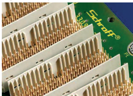
Рис. 4. Метрические соединители
