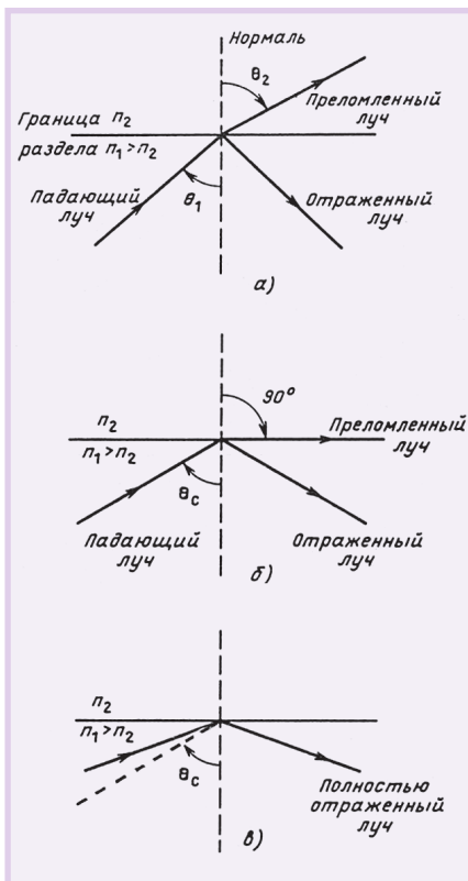
Рис. 1. Отражение и преломление света на границе двух сред
