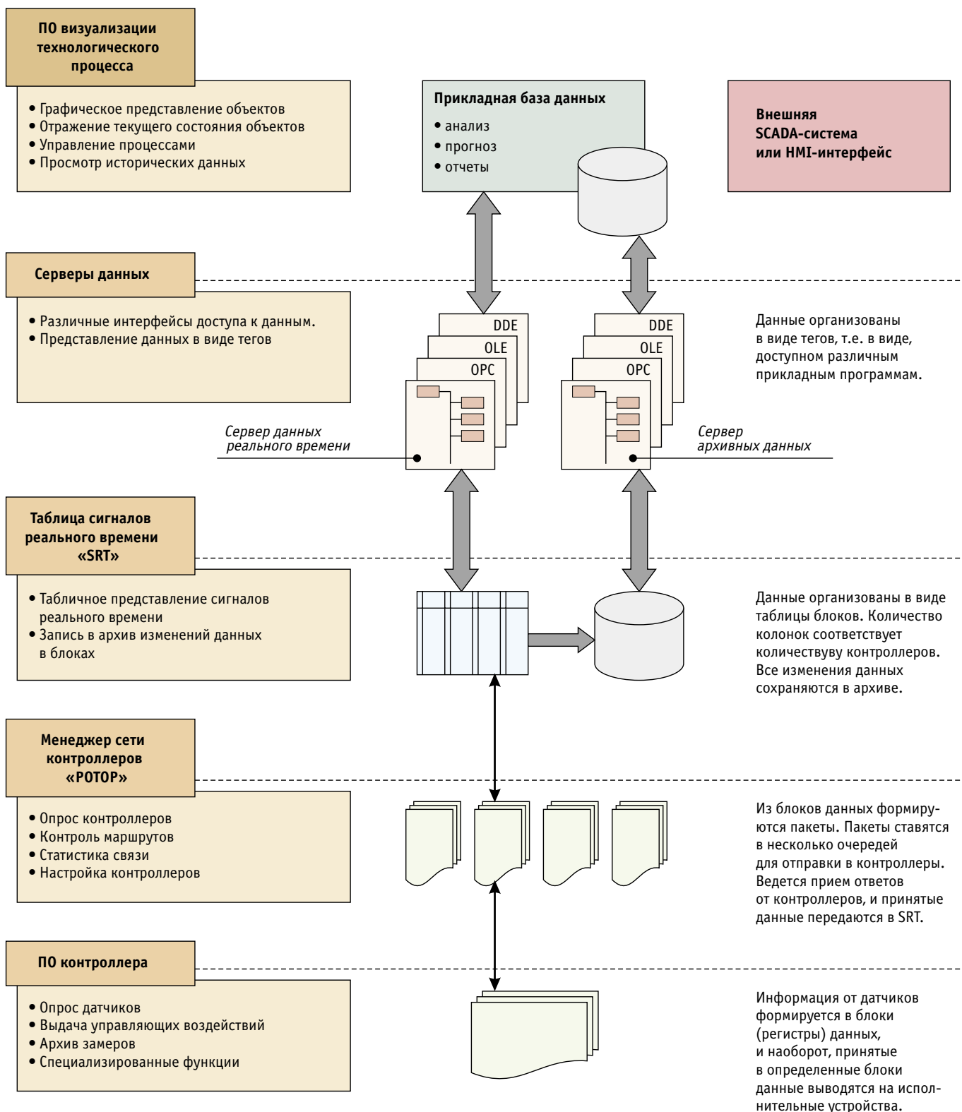
Рис. 5. Структура программного обеспечения системы «Мега»
