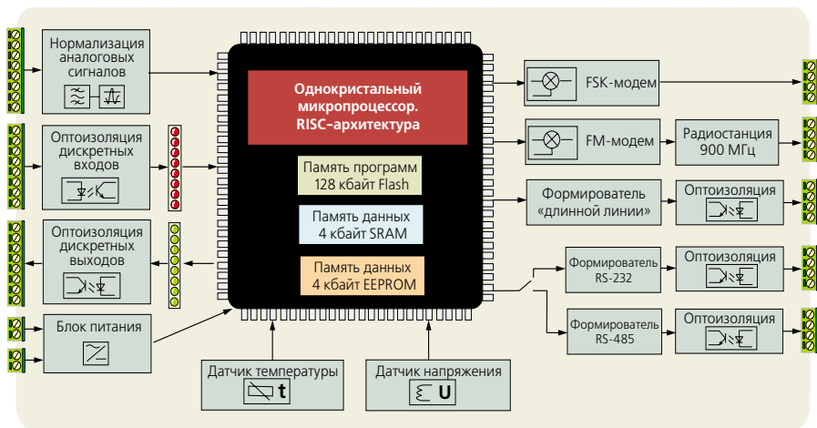
Рис. 7. Структура контроллера «Мега»
