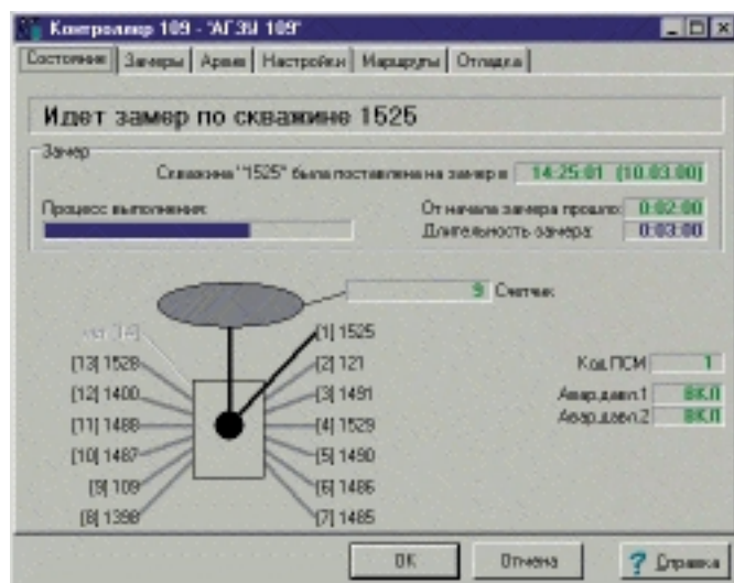
Рис. 12. Замер дебитов по отводам контроллером ГЗУ
