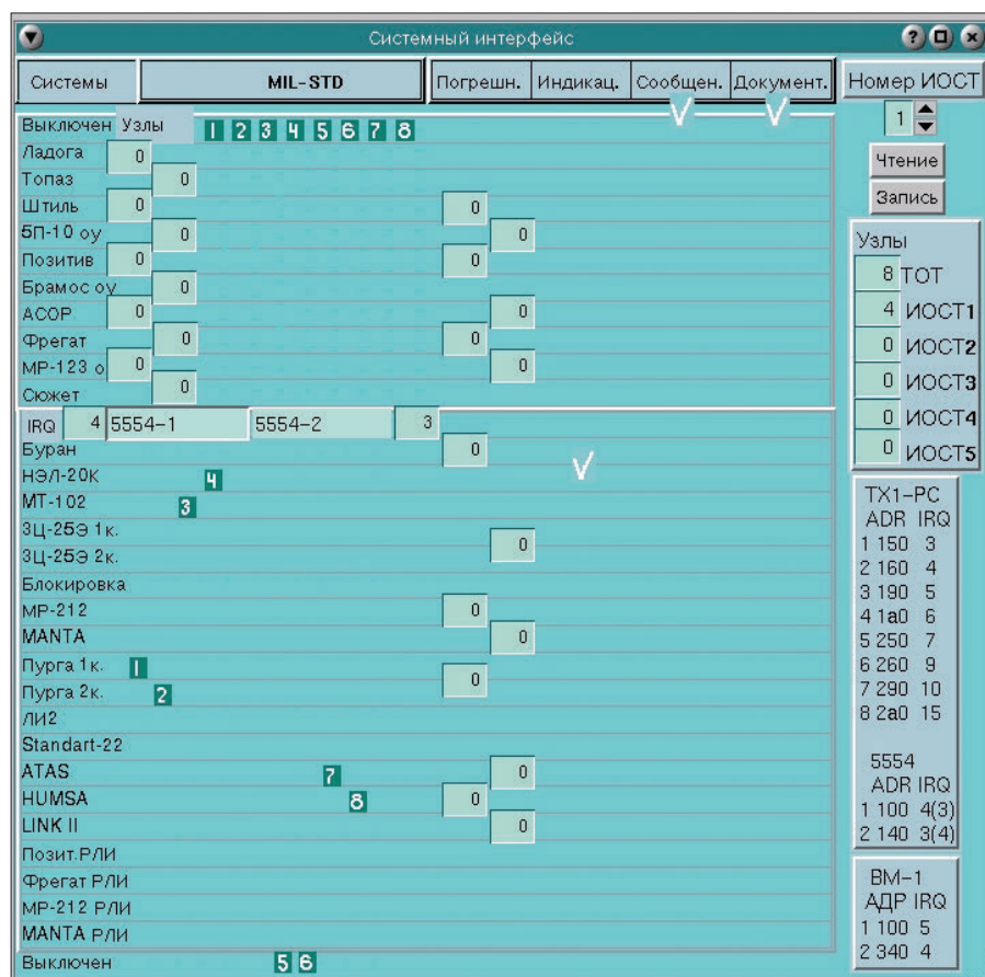
Рис. 10. Окно «Системный интерфейс»
