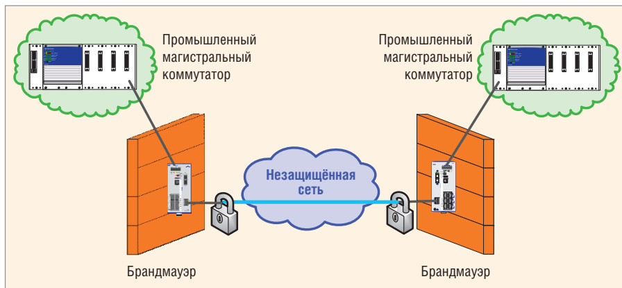
Рис. 3. Реализация защиты соединения между отдельными сетями
