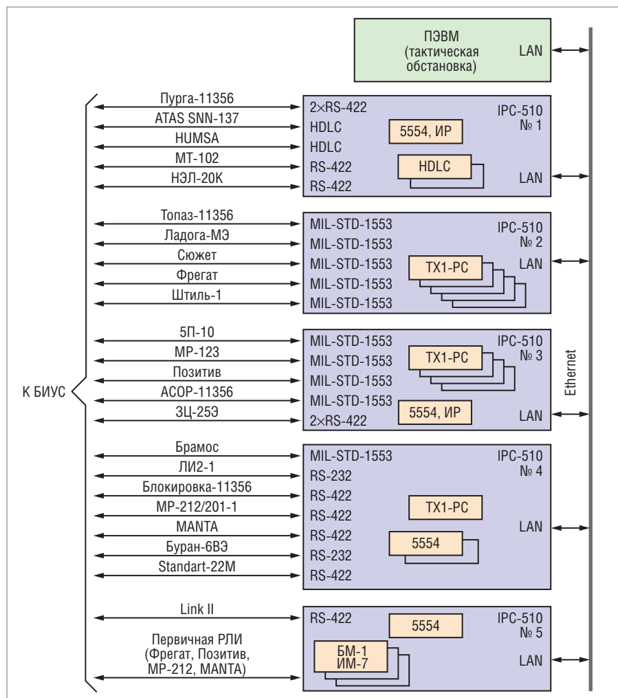
Рис. 1. Структурная схема имитационного комплекса БИУС «Требование-М»
