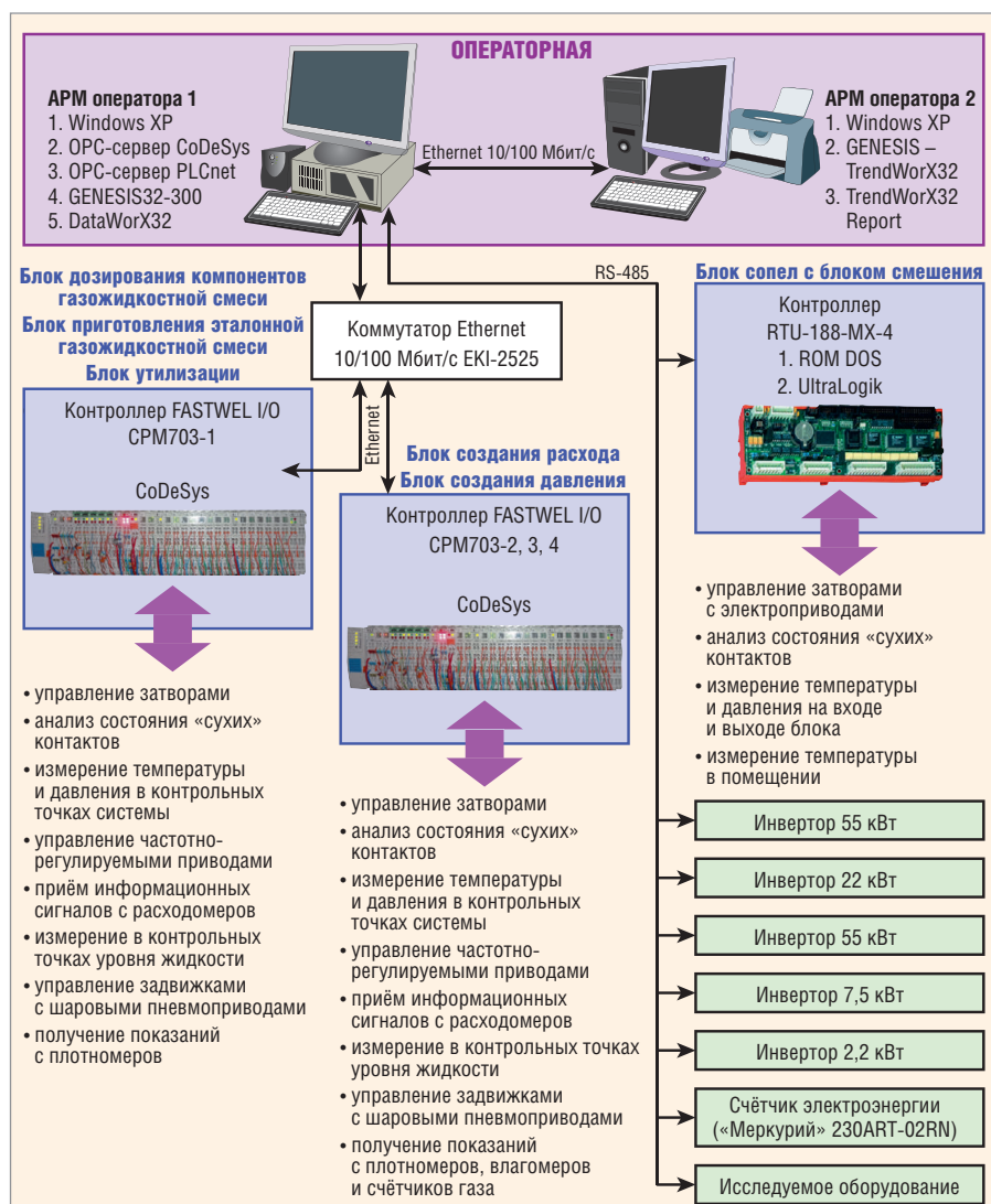
Рис. 4. Структура АСУ ГЭТ 195-2011
