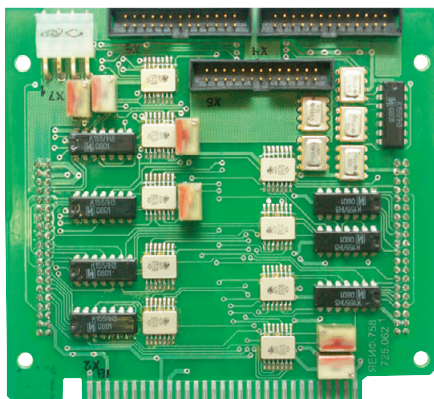
Рис. 4. Модуль ИМ-7
