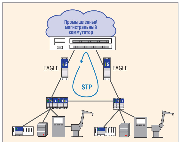
Рис. 9. Использование STP-резервирования
