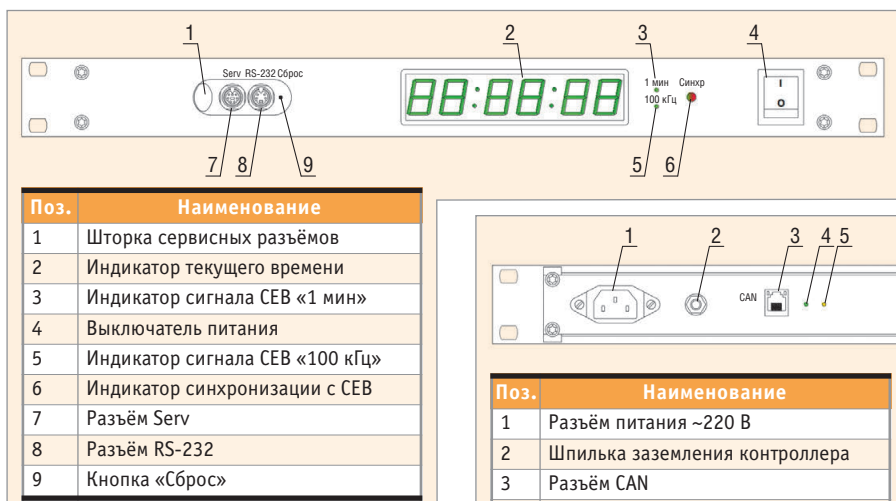
Рис. 2. Чертёж передней панели изделия
