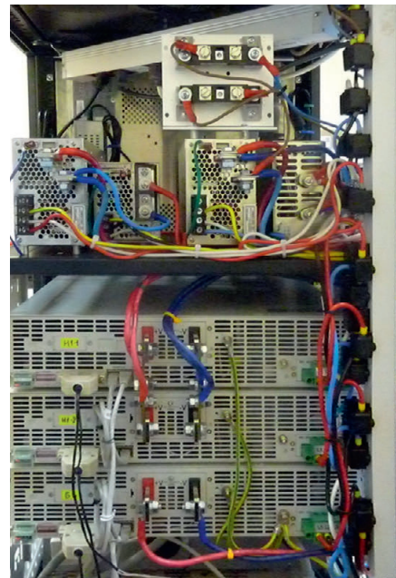
Рис. 9. Внутреннее устройство имитатора варианта 1
