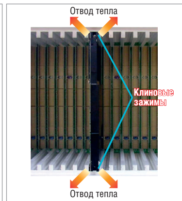
Рис. 3. 6U CompactPCI-модуль с кондуктивным теплоотводом, установленный внутри шасси
