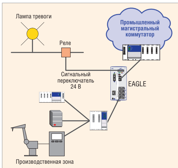
Рис. 8. Использование сигнального маячка для оповещения
