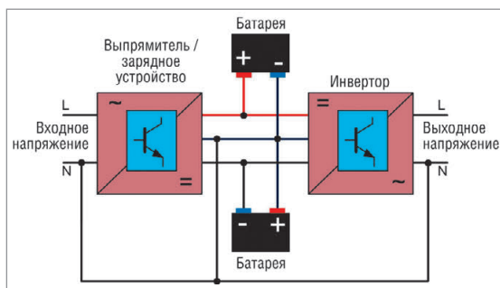
Рис. 4. Структурная схема модуля UPS
