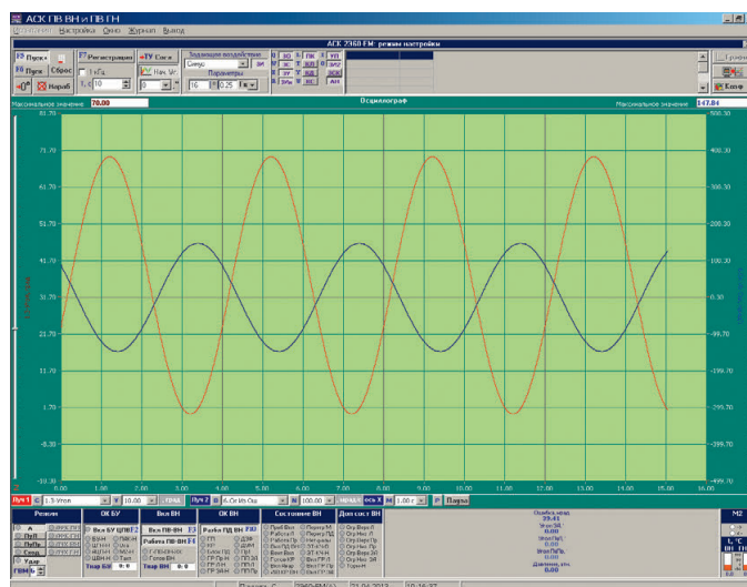
Рис. 4. Вид панели управления в режиме настройки ПНС
