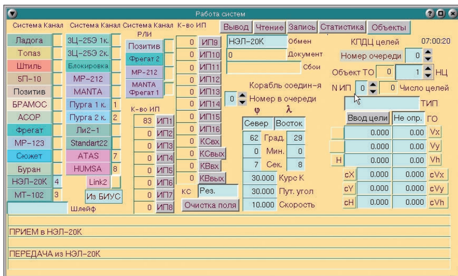
Рис. 7. Окно «Работа систем» модуля IOST
