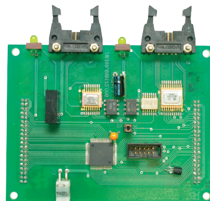
Рис. 2. Модуль БМ-1
