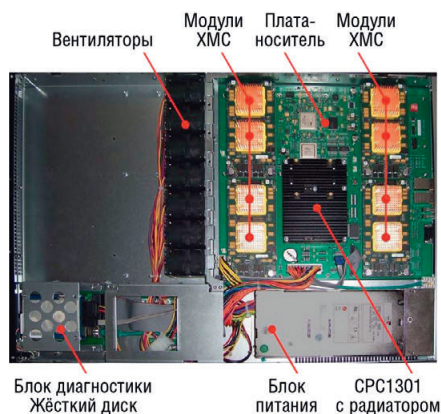
Рис. 1. Общий вид БВР-01
