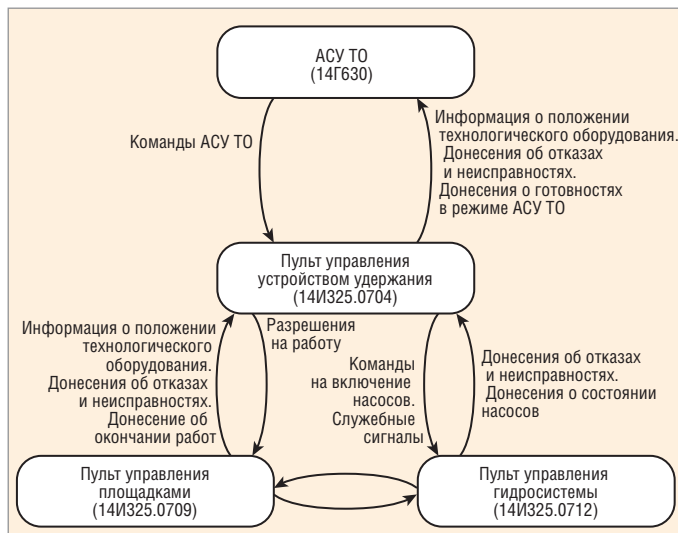
Рис. 4. Функциональные связи оборудования системы управления
