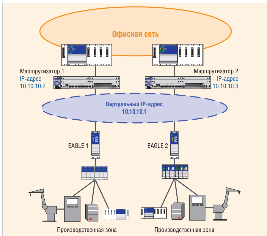
Рис. 6. Фрагмент сети третьего уровня OSI и реализация защиты в ней
