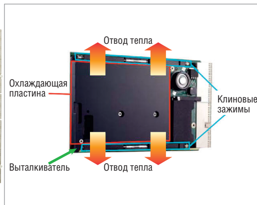
Рис. 2. Расположение теплоотводящей пластины на 3U CompactPCI-модуле с кондуктивным охлаждением
