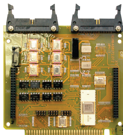
Рис. 3. Модуль ИМ-1
