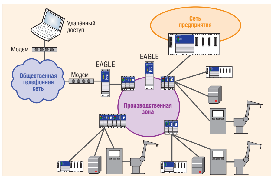
Рис. 5. Использование VPN-туннеля для получения удалённого доступа к сети
