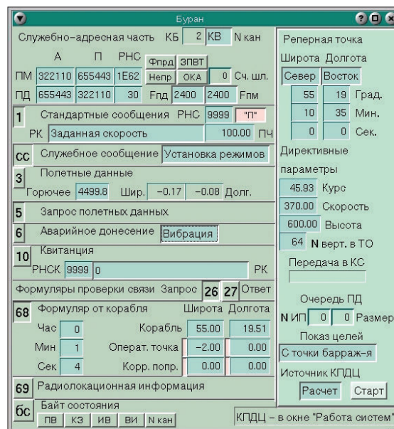
Рис. 8. Окно имитатора системы «Буран»
