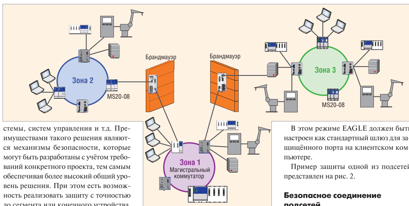
Рис. 2. Реализация защиты отдельной подсети
