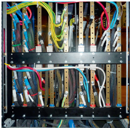
Рис. 7. Расположение входных соединителей (а) и выходных шин питания постоянного тока (б) внутри имитатора варианта 1
