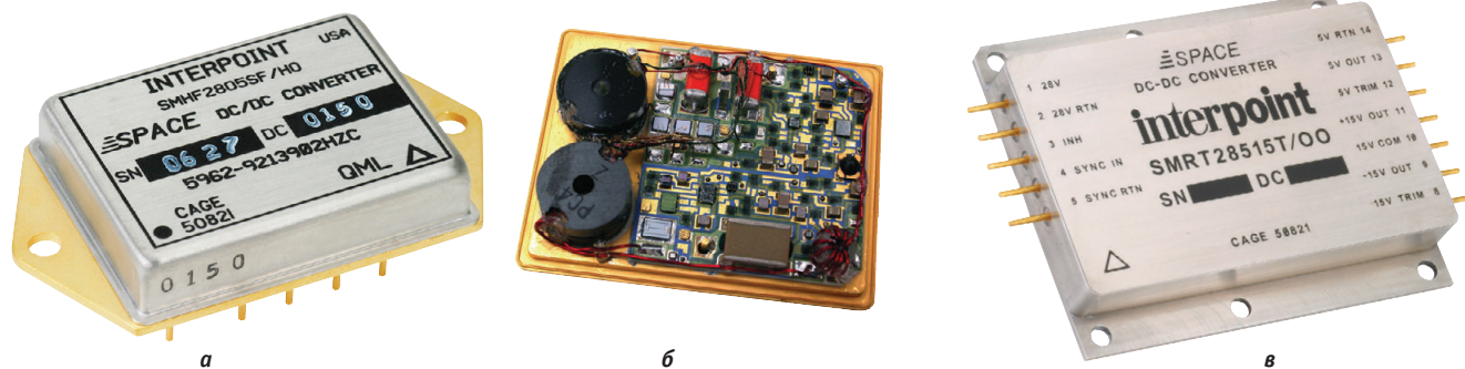
Рис. 1. Внешний вид конструкции: а – радиационно-стойкого интегрально-гибридного DC/DC-преобразователя серии SMHF с крепёжными фланцами; б – преобразователя серии SMHF без крышки; в – радиационно-стойкого DC/DC-преобразователя серии SMRT
