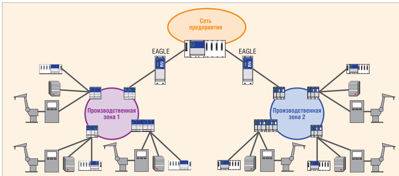
Рис. 4. Реализация защиты при использовании одинаковых сегментов сети
