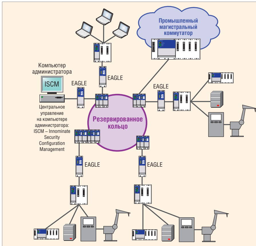
Рис. 7. Использование системы ISCM для конфигурирования параметров безопасности
