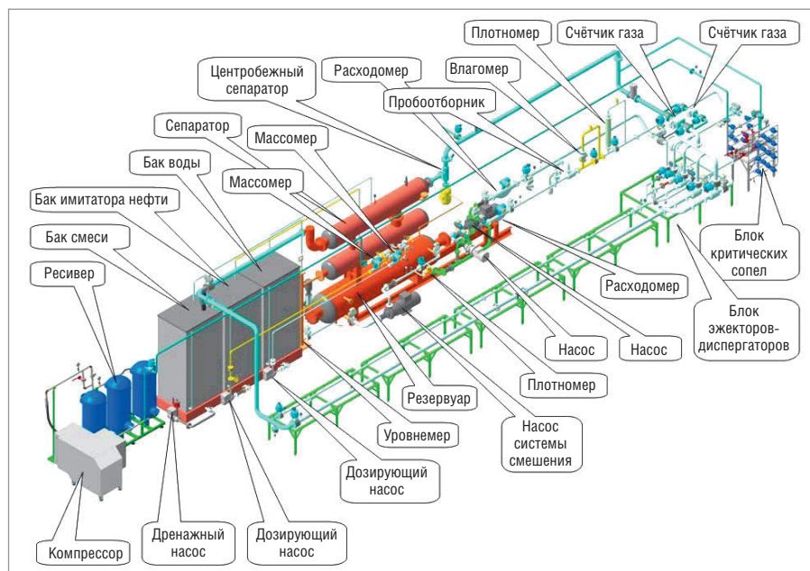
Рис. 3. Схема ГЭТ 195-2011
