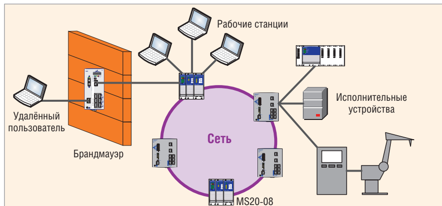
Рис. 1. Реализация защиты сервисного порта
