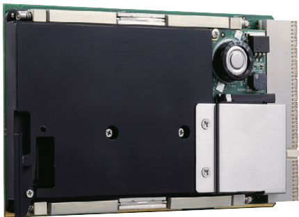
Рис. 4. CompactPCI-модуль с кондуктивным теплоотводом CT-31
