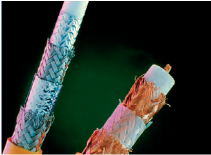
Рис. 13. Оплётка
