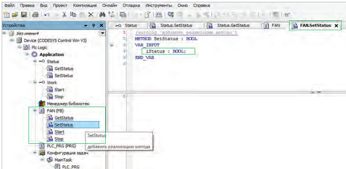
Рис. 8. Созданный класс вентиляторов Fan (методы, созданные в интерфейсе, автоматически перенесены в этот класс)
