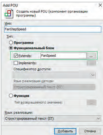
Рис. 16. Класс FanStepSpeed, созданный на базе класса FanSpeed
