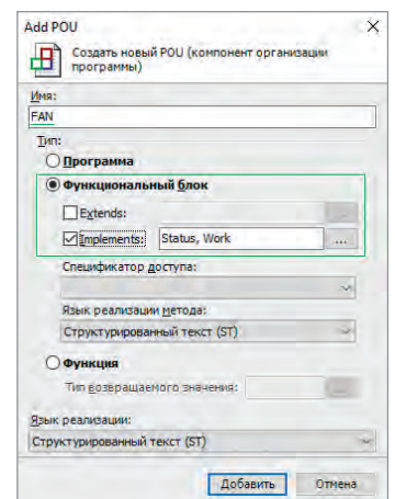
Рис. 7. Поле Implements позволяет добавлять интерфейсы, реализованные в данном классе
