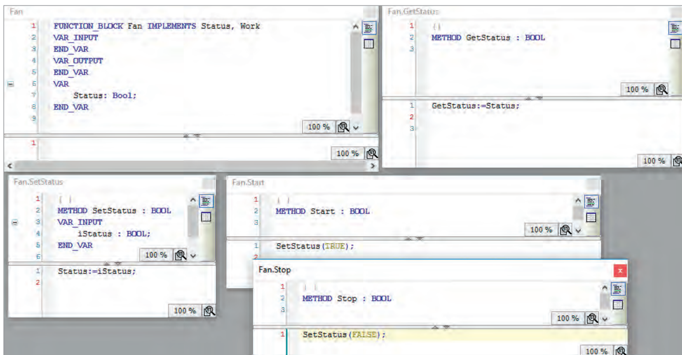
Рис. 9. Реализация методов класса Fan
