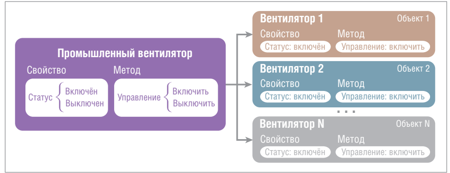
Рис. 3. N объектов (экземпляров), относящихся к классу вентиляторов
