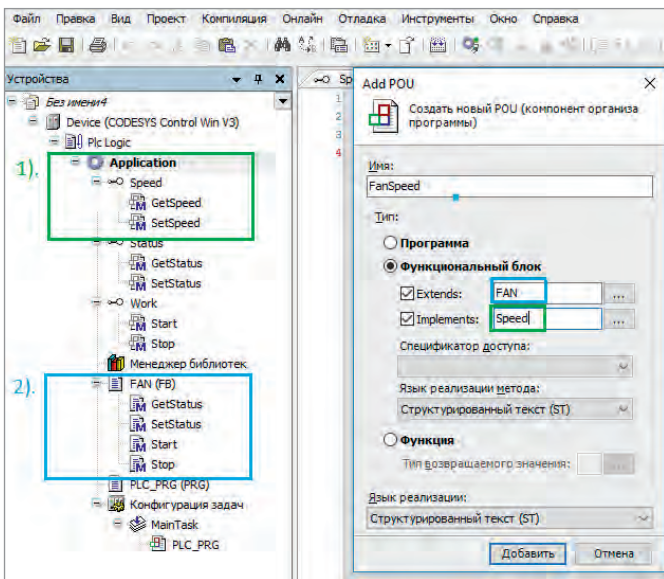
Рис. 12. Создание нового класса FanSpeed
